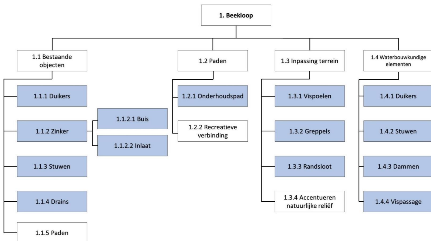
Figuur 6: Objectenboom
