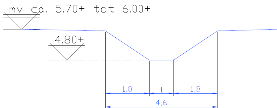
Figuur 3: nieuw profiel A-watergang noordzijde
