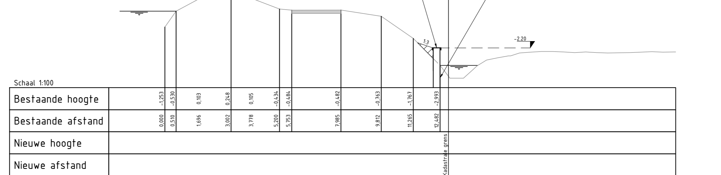
Dwarsprofiel 07-07 0,000 N.A.P.
