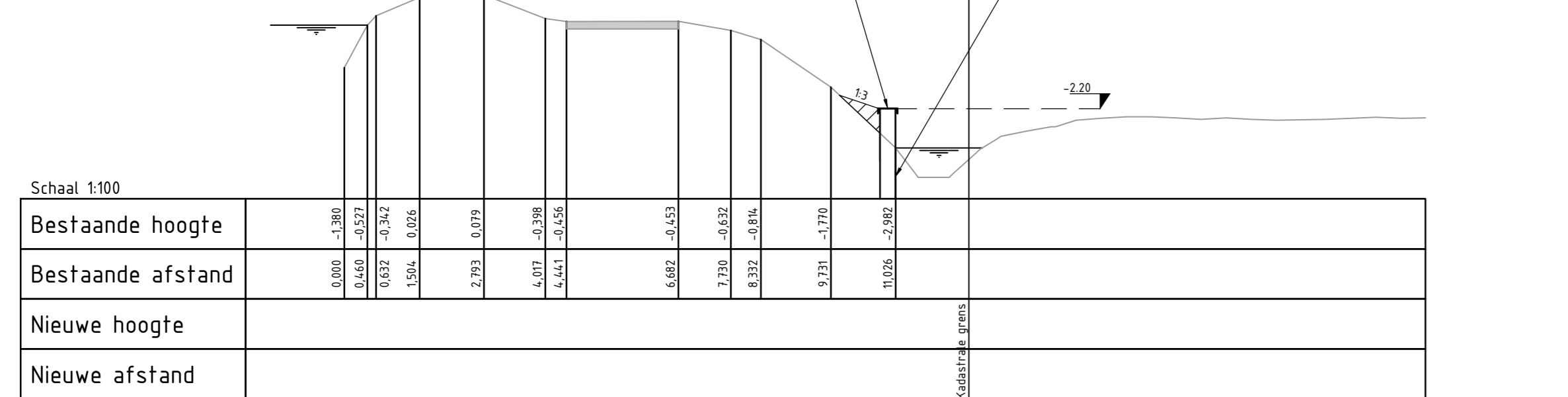
Dwarsprofiel 04-04 0,000 N.A.P.
