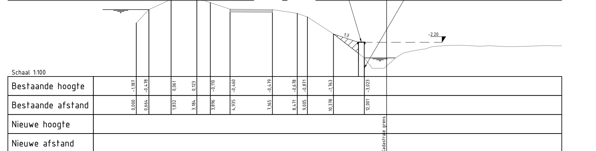
Dwarsprofiel 05-05 0,000 N.A.P.
