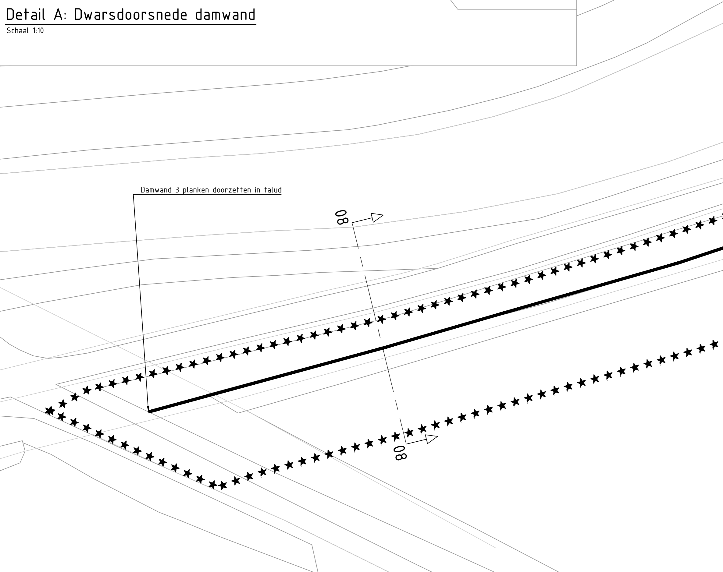
Bovenaanzicht Locatie 1 Schaal 1:250
