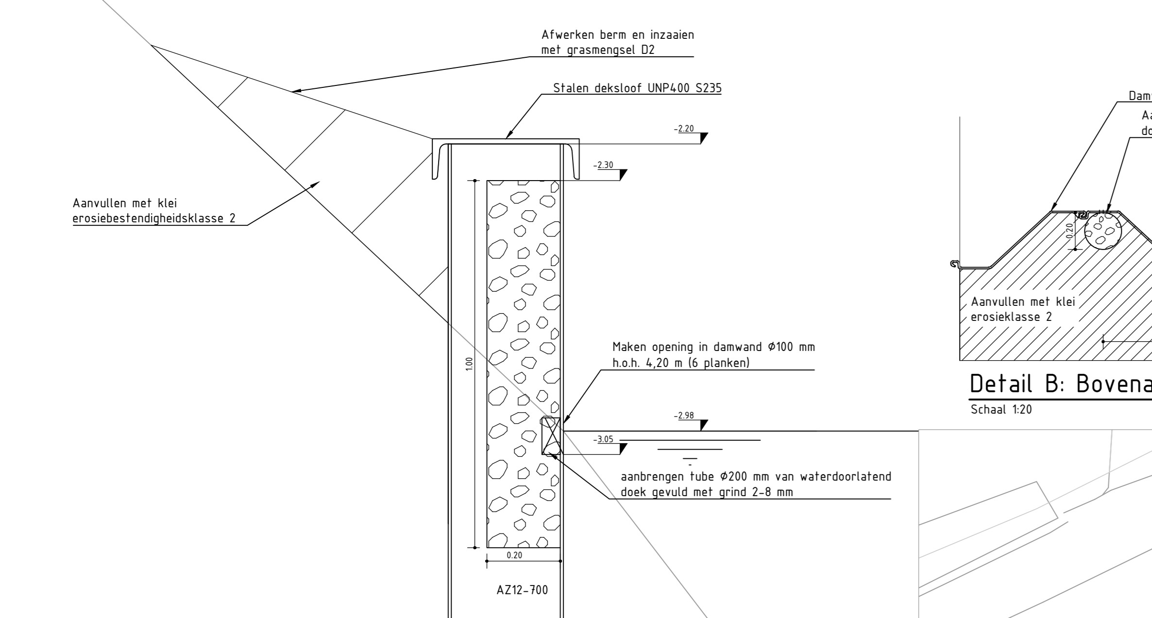
Detail A: Dwarsdoorsnede damwand Schaal 1:10
