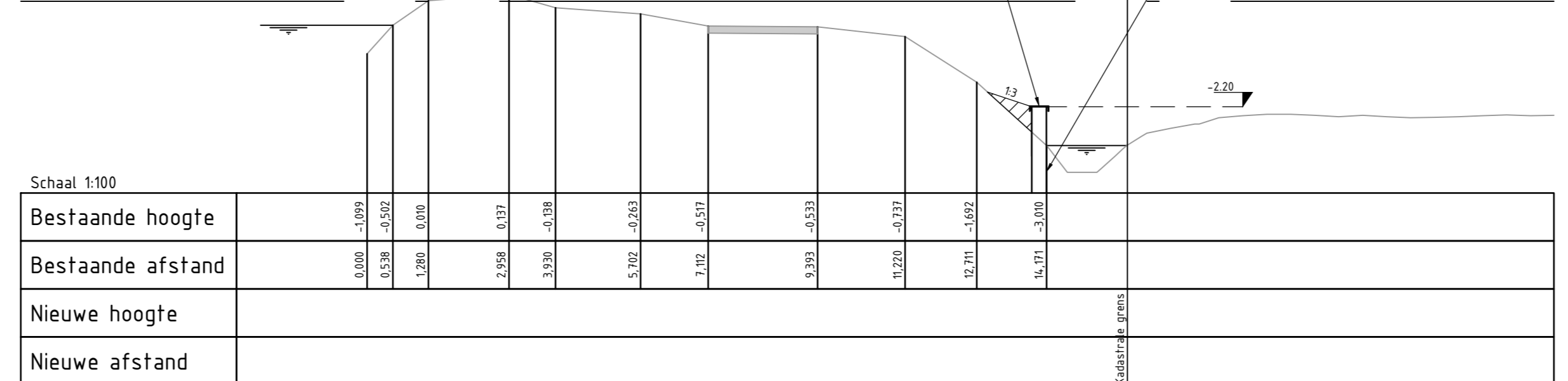
Dwarsprofiel 08-08 0,000 N.A.P.
