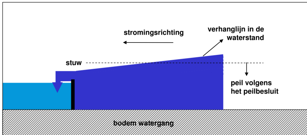
Afbeelding 8.5 Verhanglijn in de waterstand bij een afvoersituatie
