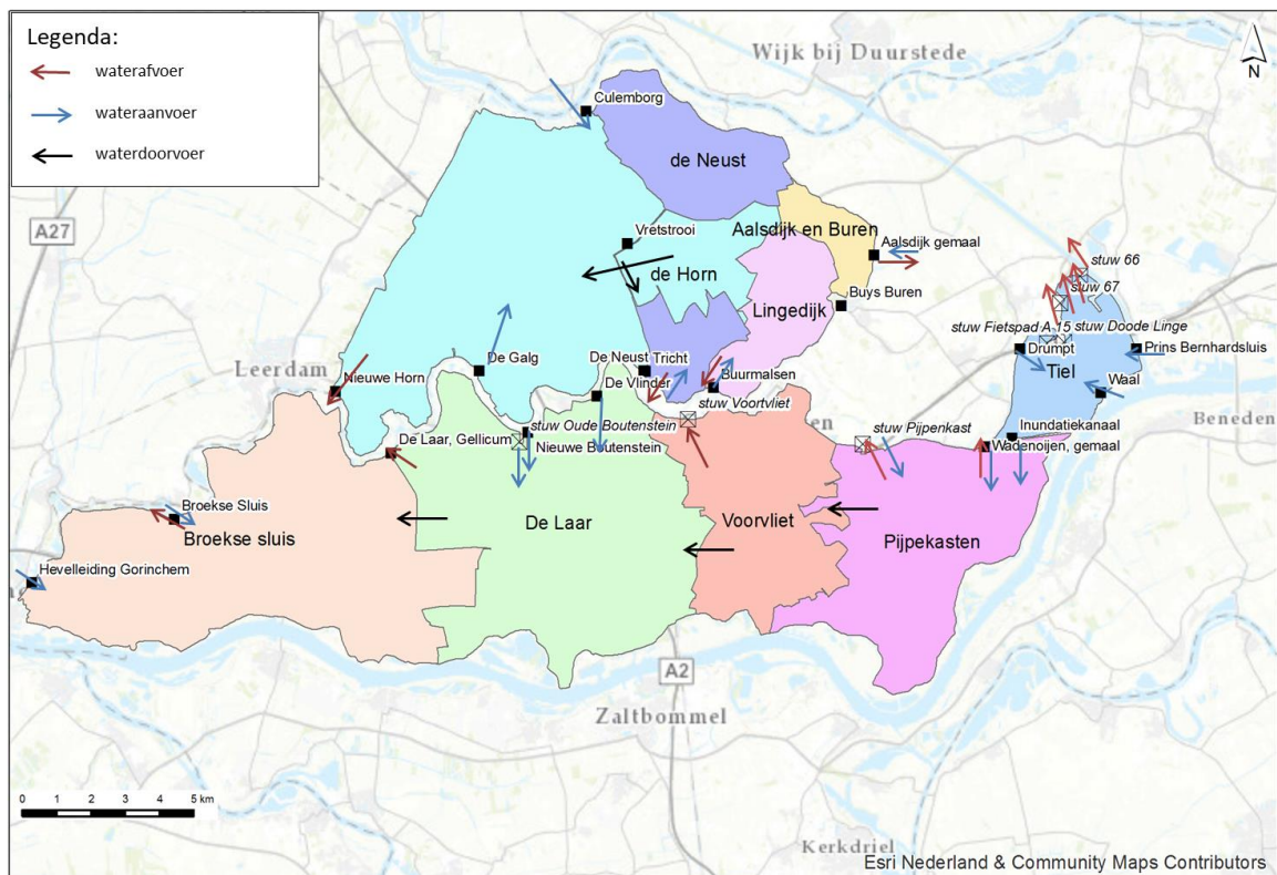
Afbeelding 2.7 Schematische tekening watersysteem Tielervwaard en Lek & Linge
