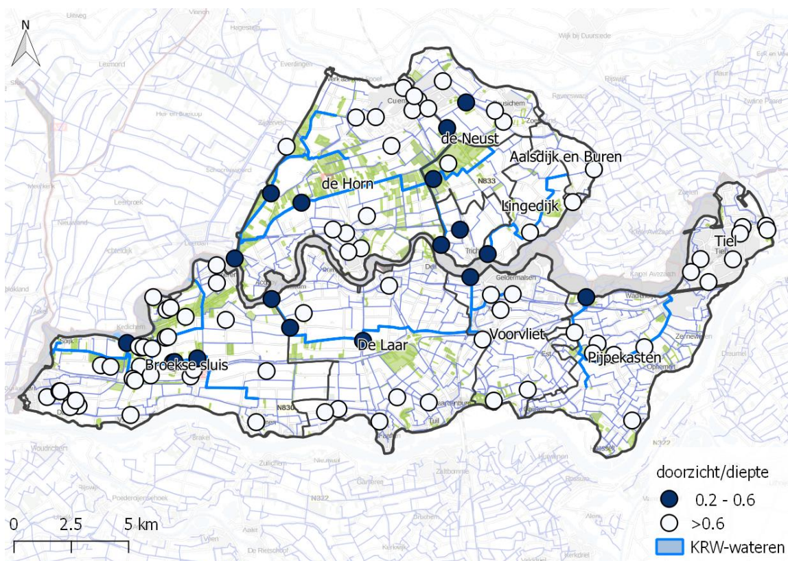
Afbeelding I.2 Lichtklimaat (doorzicht/diepte, periode 2012 t/m 2016)
