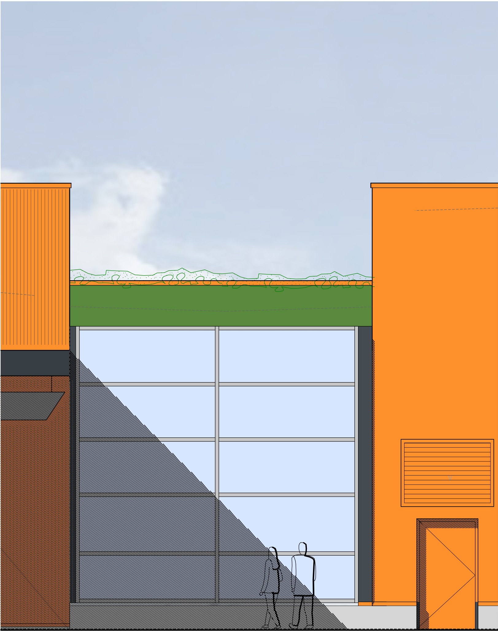
GEVEL (s 1:50)
