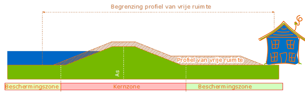
1. Buiten profiel van vrije ruimte
