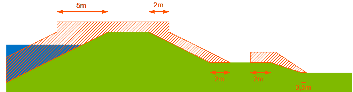
Figuur 4: boomvrij profiel
