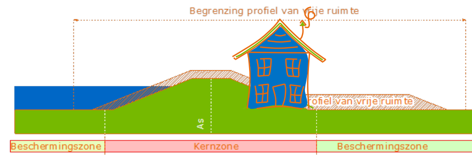
4. Binnen talud van de dijk
