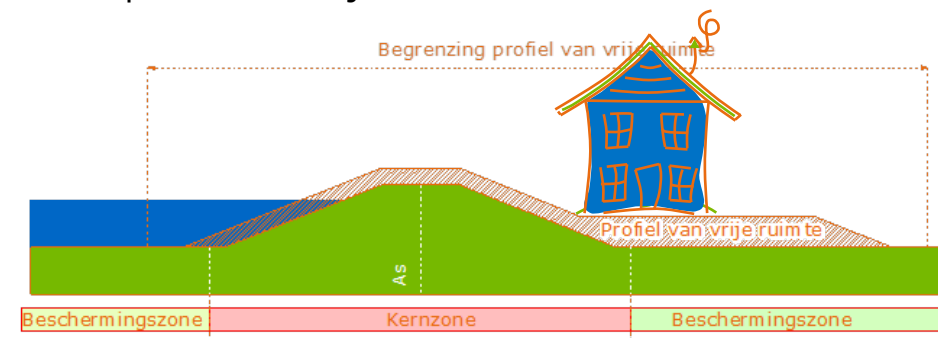
3. Boven profiel van vrije ruimte
