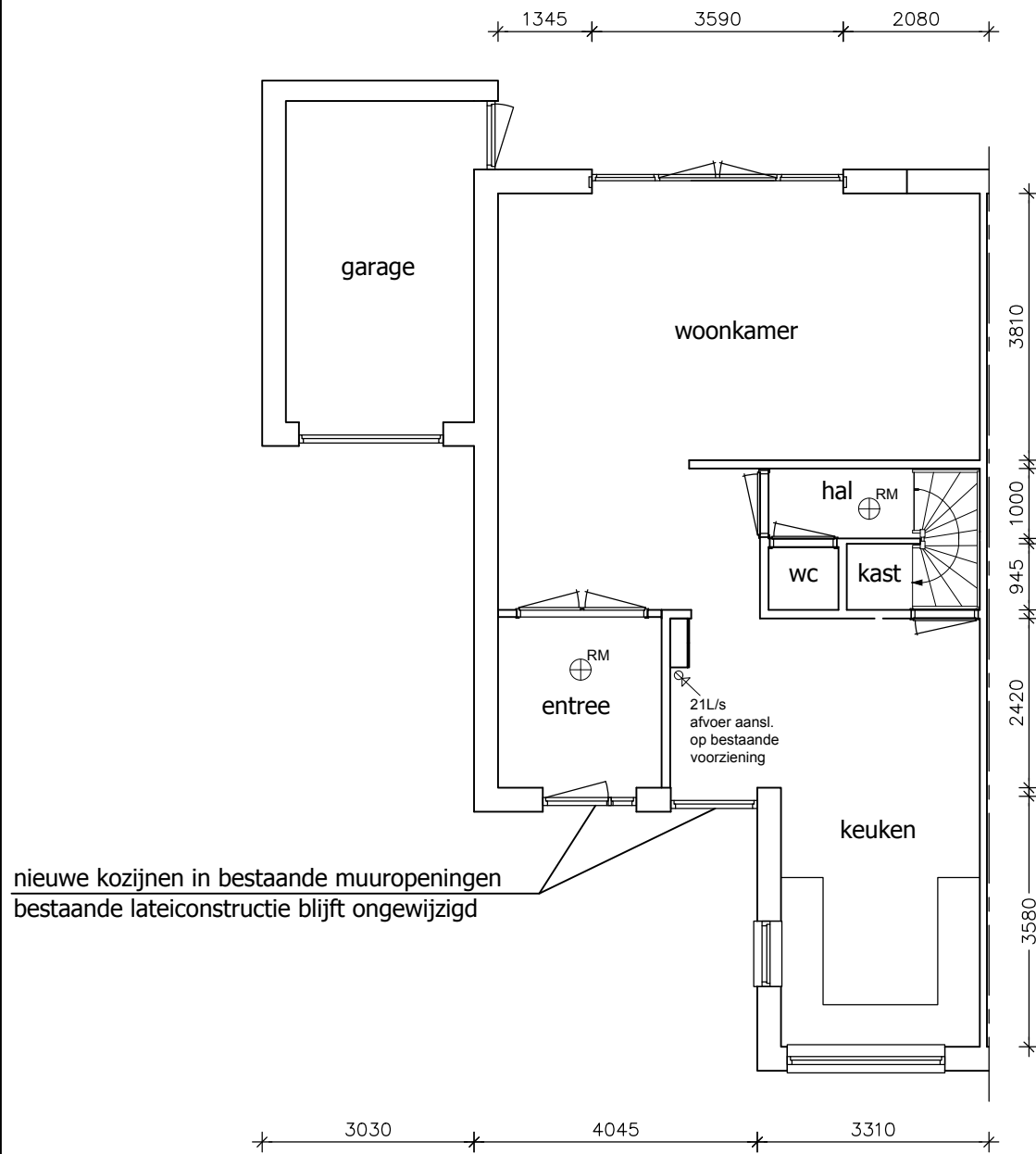
berekening adviesbureau Sterk : Projectnummer : 13276 d.d. 12-04-2019 CONSTRUCTIE nieuw
