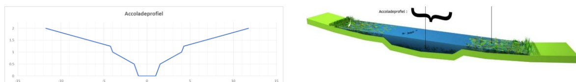
Figuur 10 Principeprofielen accoladeprofiel
