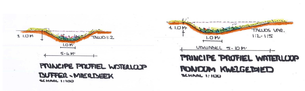
Afbeelding 6: Impressies van de profielen ten behoeve van de Mierbeek.
