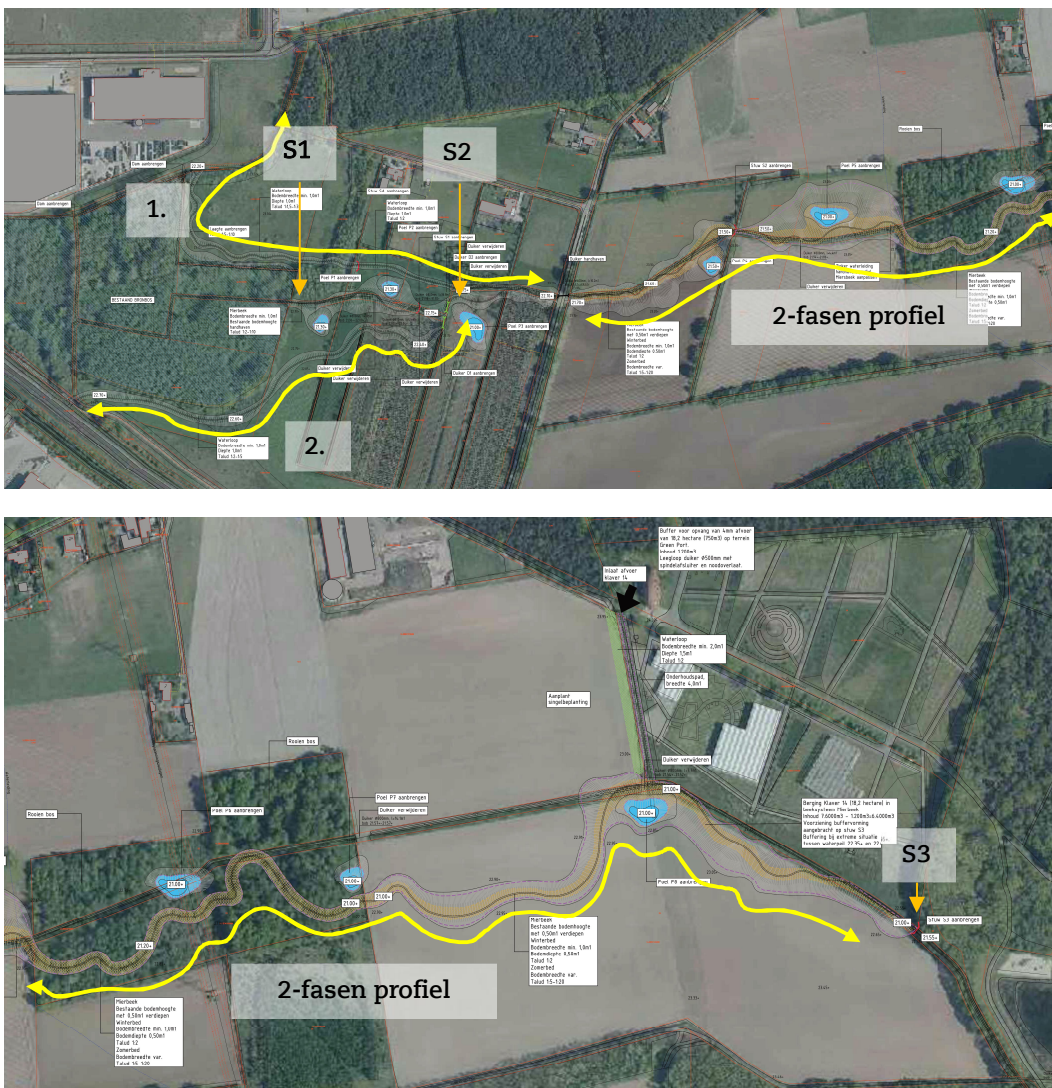
Afbeelding 4: Verkleinde weergaven van de ontwerptekeningen uit Bijlage 3.
