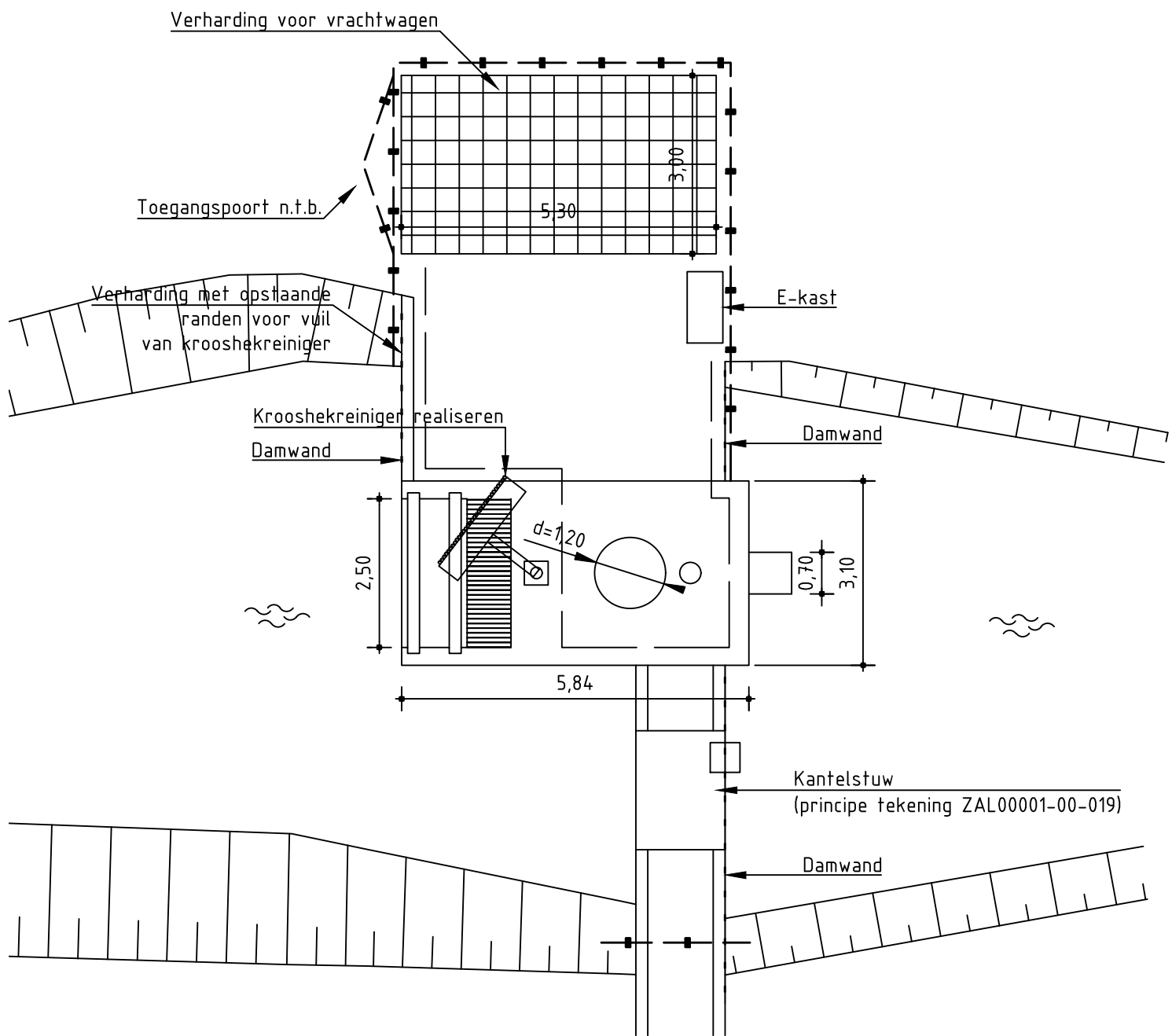
Bovenaanzicht Schaal 1:100
