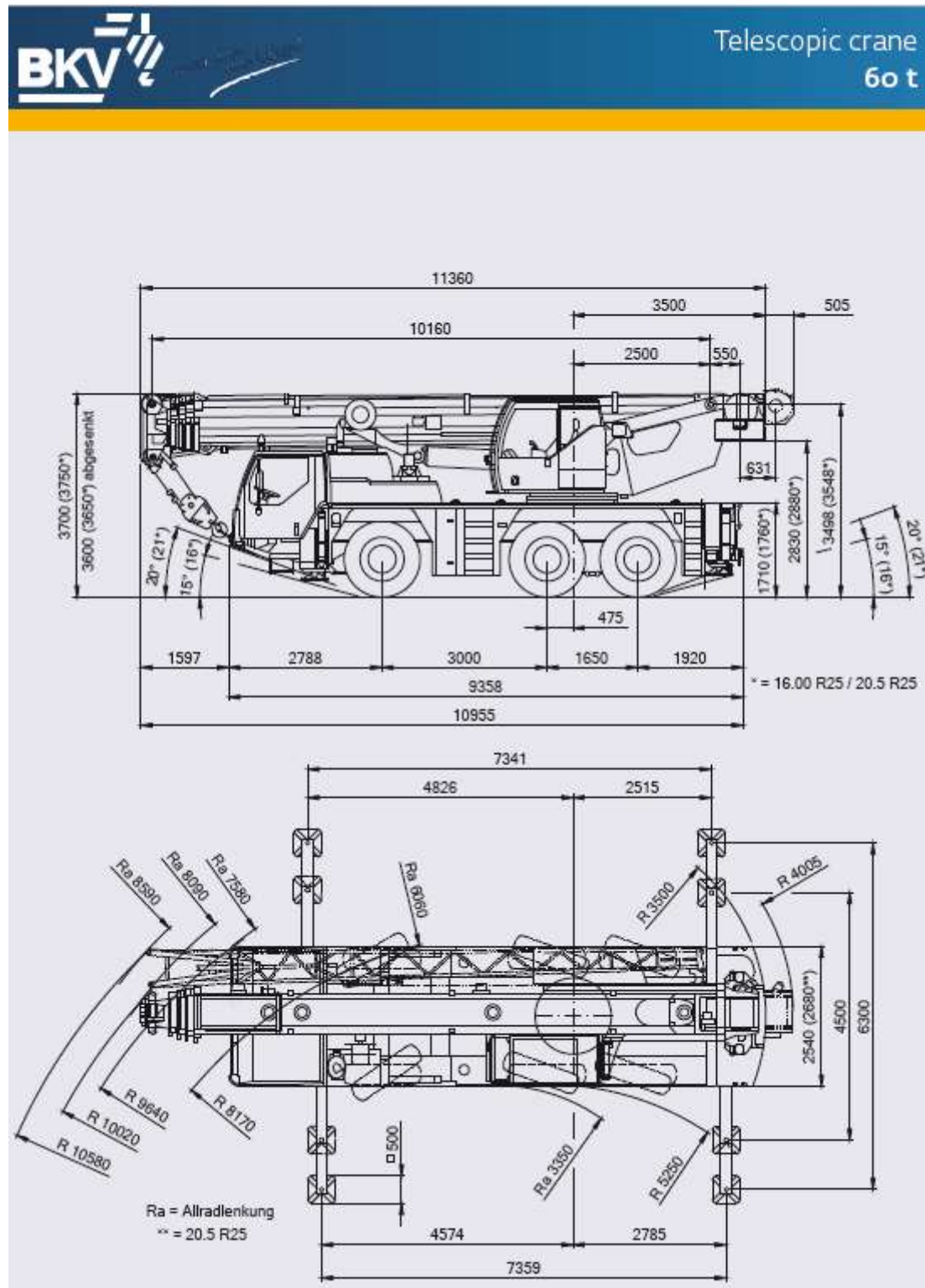
Afbeelding 4.3 Datasheet 60 tons kraan
