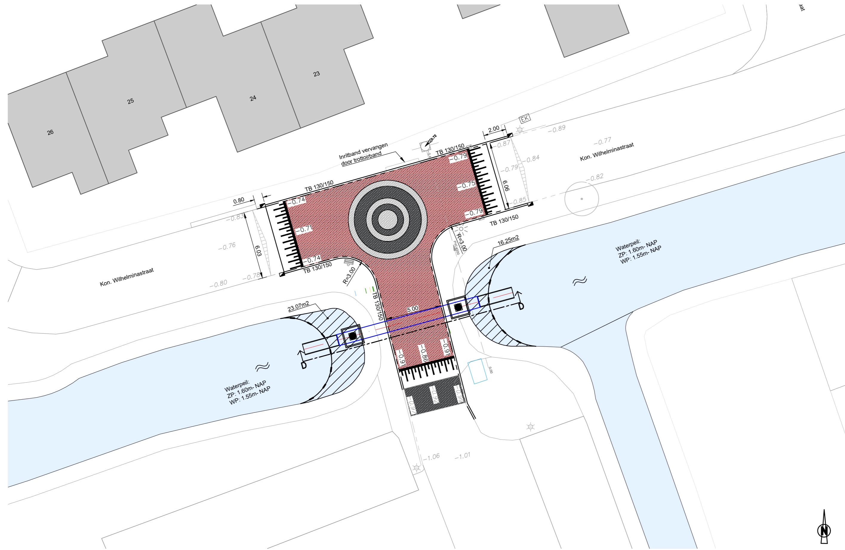
Nieuwe situatie 1:200
