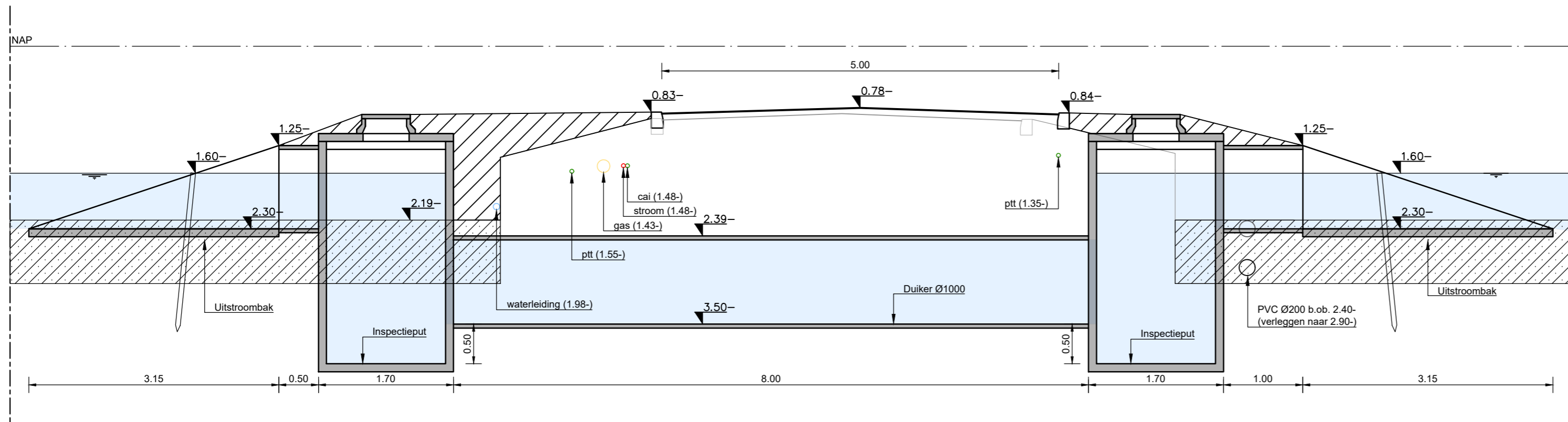
Dwarsdoorsnede D-D 1:50
