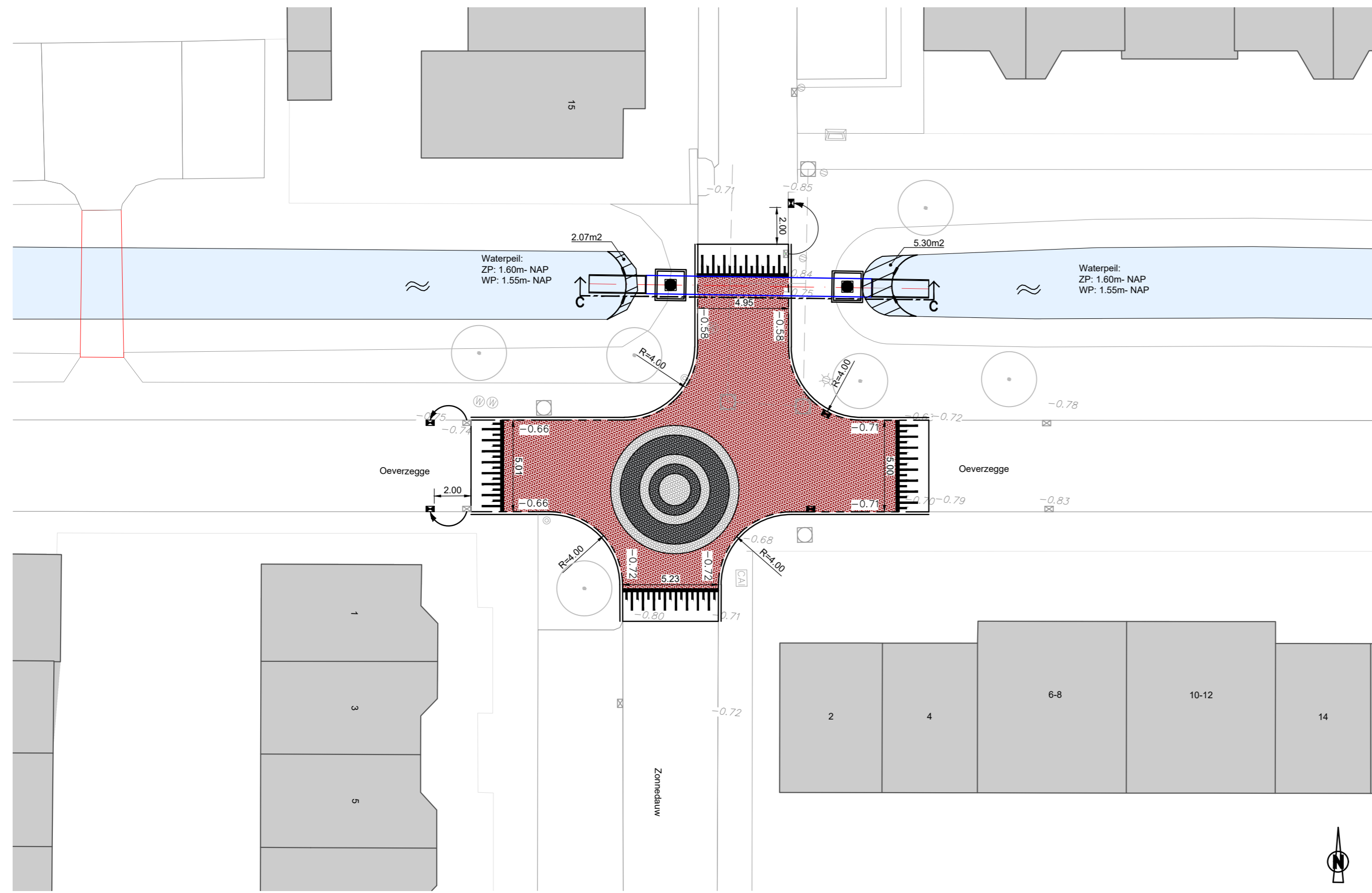
Nieuwe situatie 1:100
