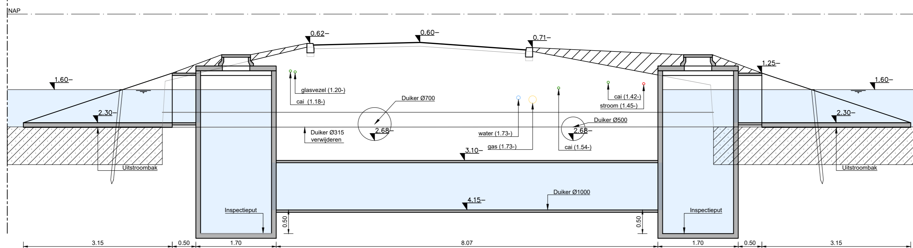
Dwarsdoorsnede C-C 1:50
