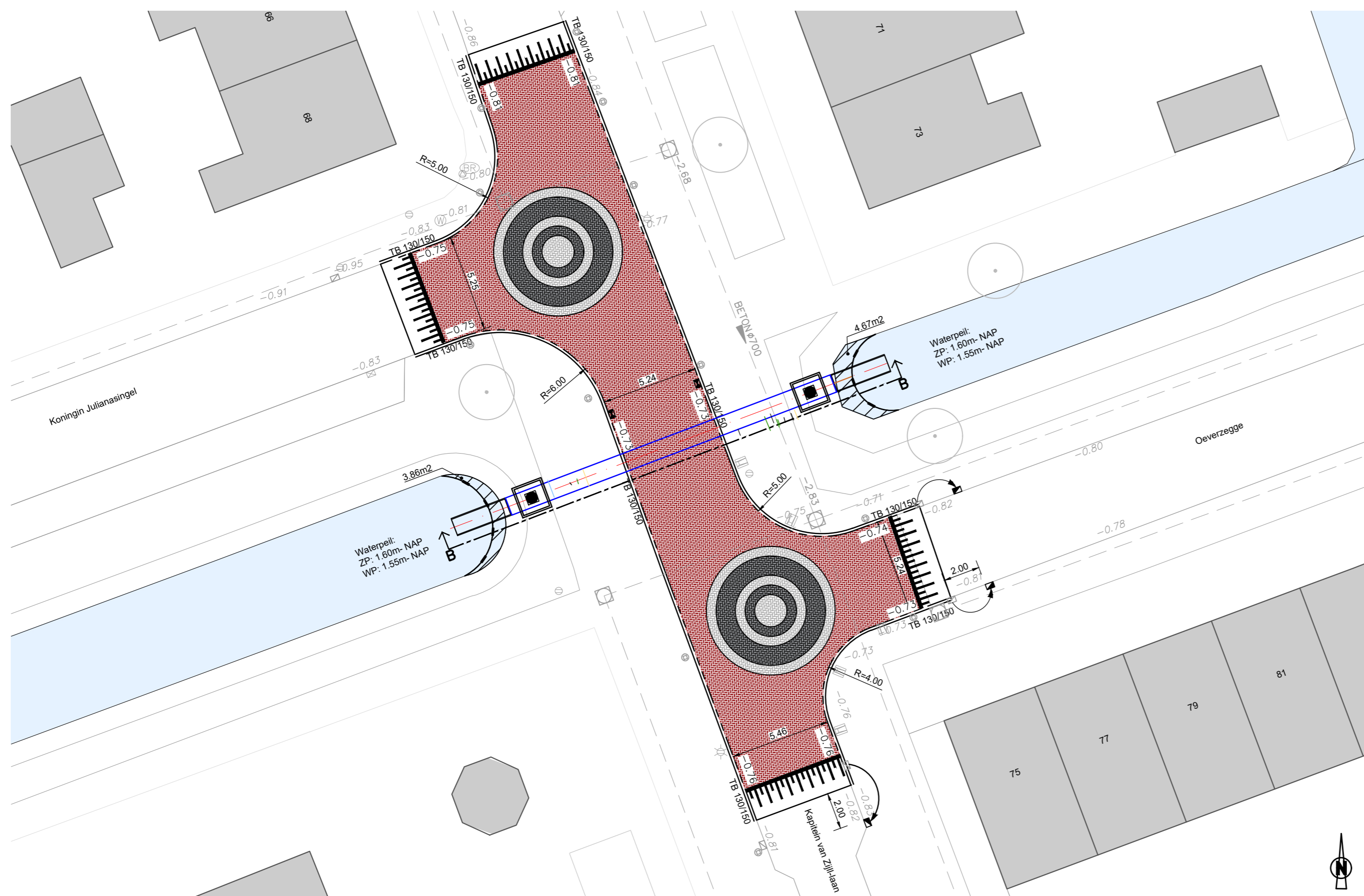
Nieuwe situatie 1:100
