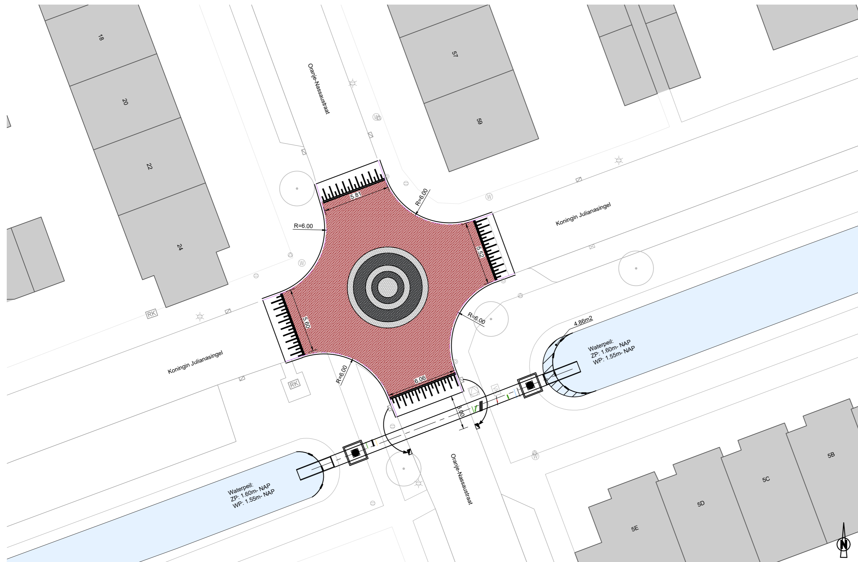
Nieuwe situatie 1:100
