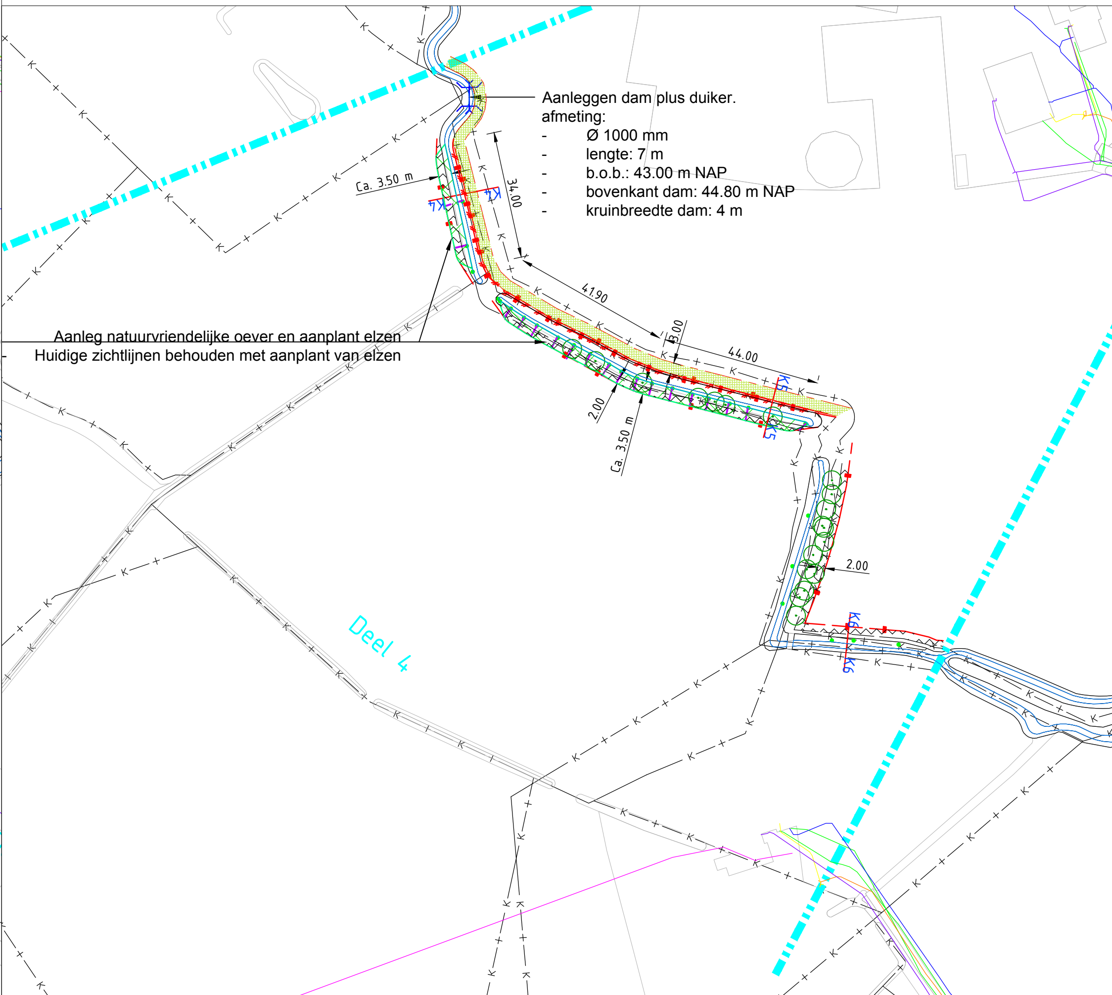
Detail Kloosterhuizenbeek deel 4 1:1000
