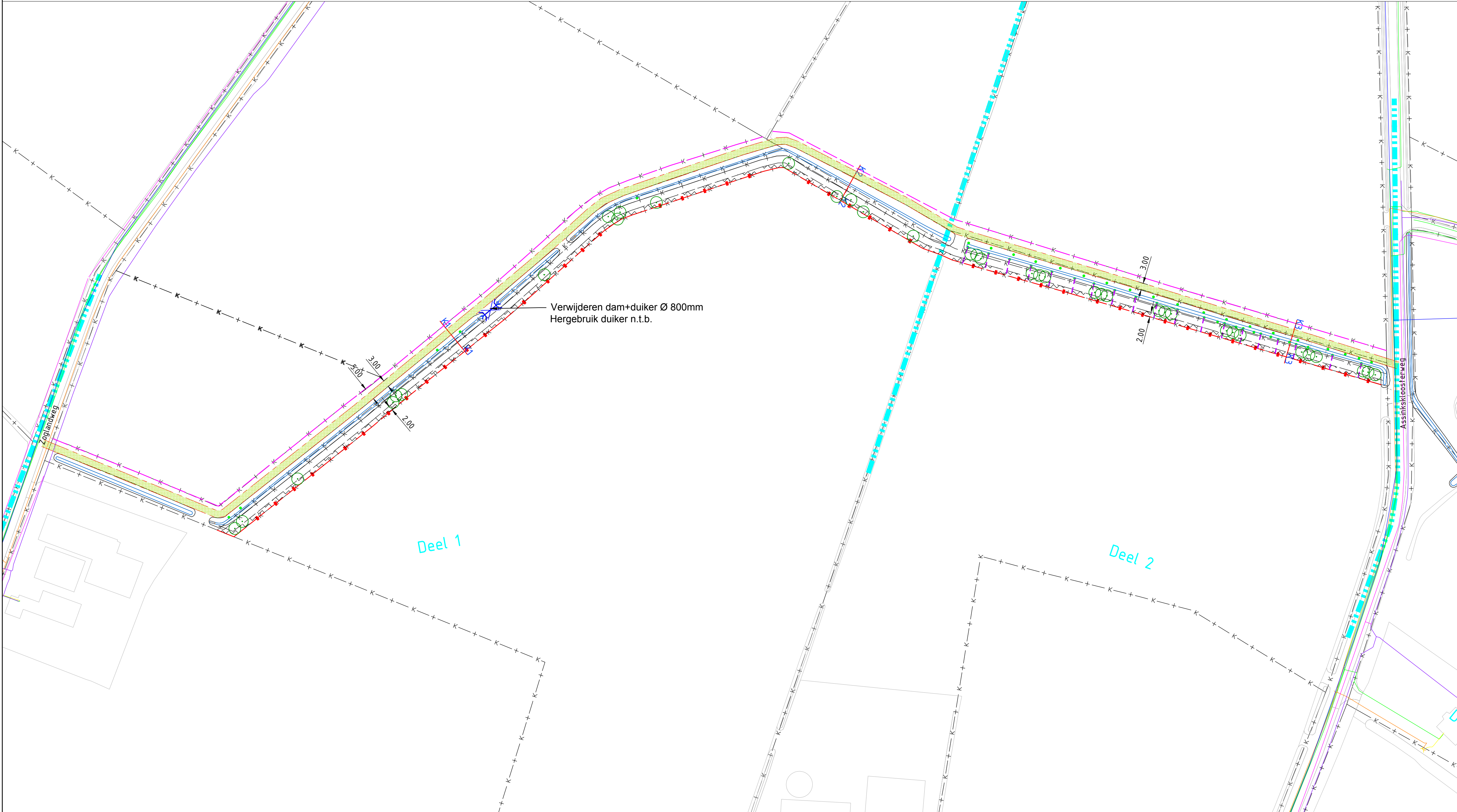
Detail Kloosterhuizenbeek deel 1 en 2 1:1000
