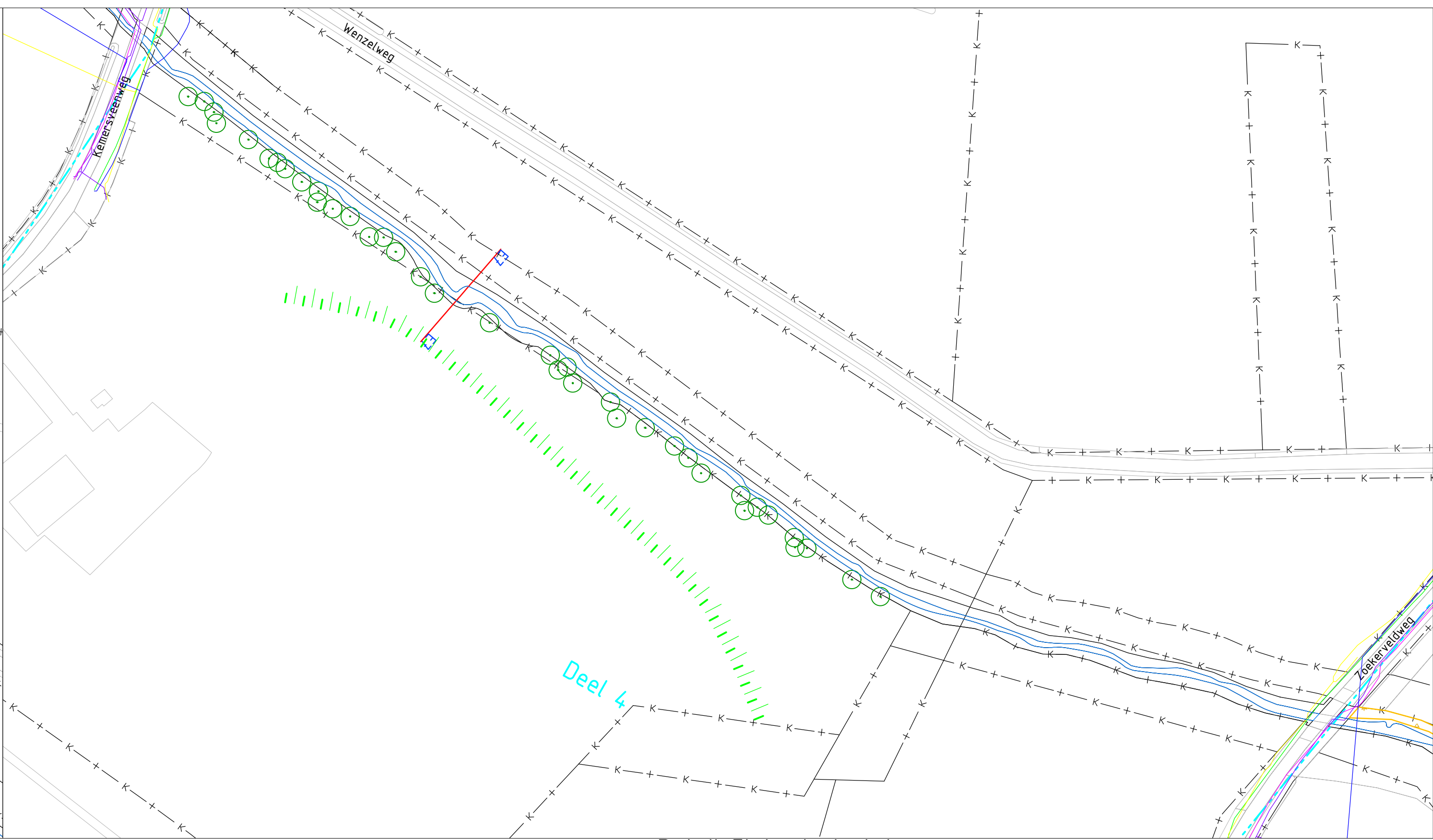
Detail Elsbeek deel 4 1:1000
