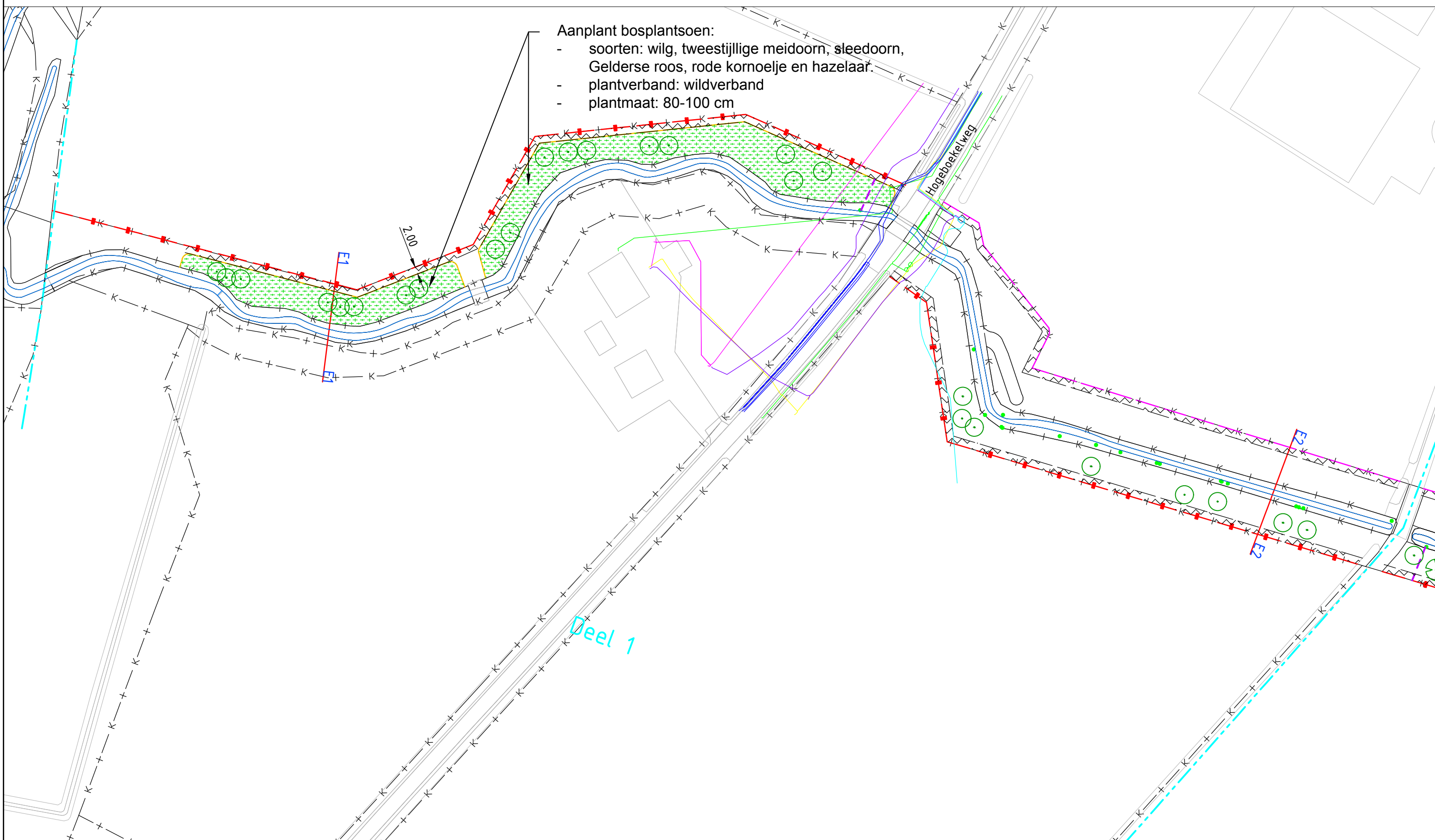
Detail Elsbeek deel 1 1:1000
