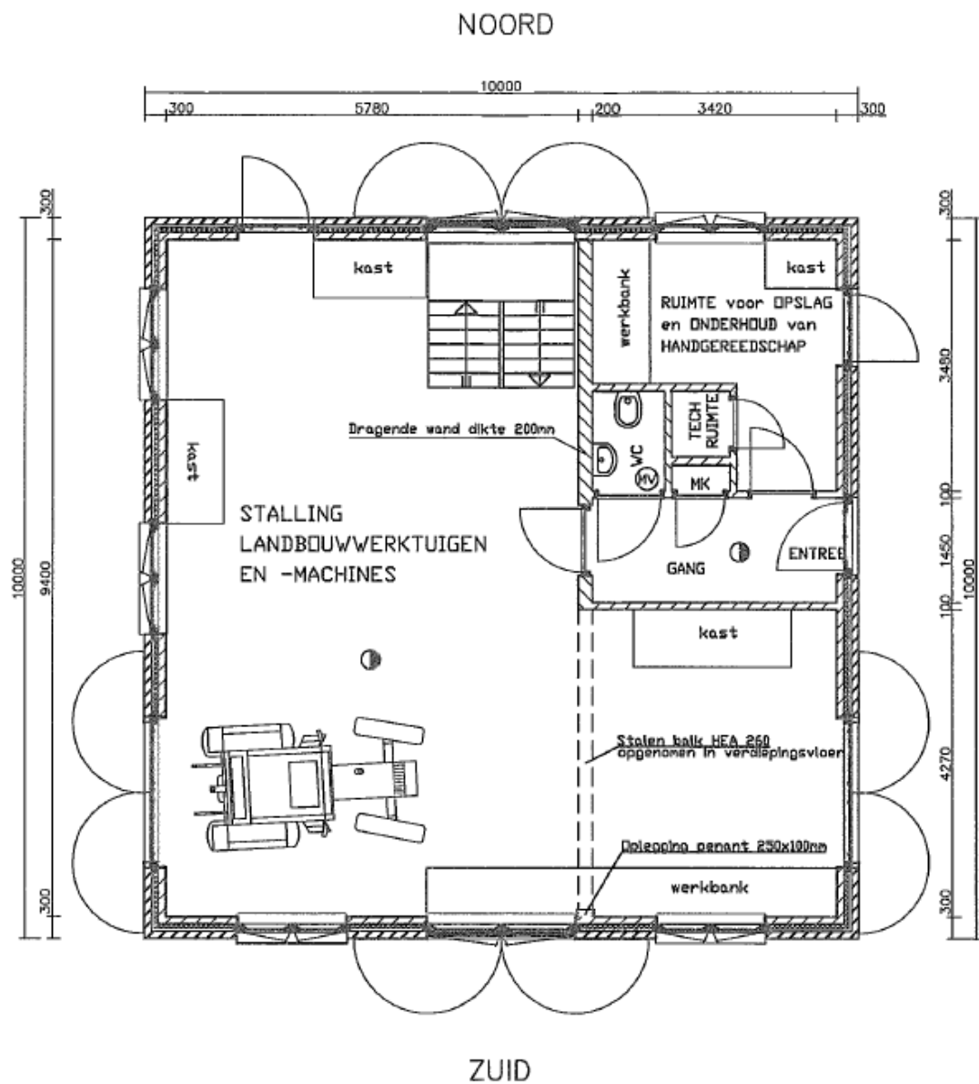
Plattegrond van te wijzigen schuur naar woning (Proosdijweg 1)
