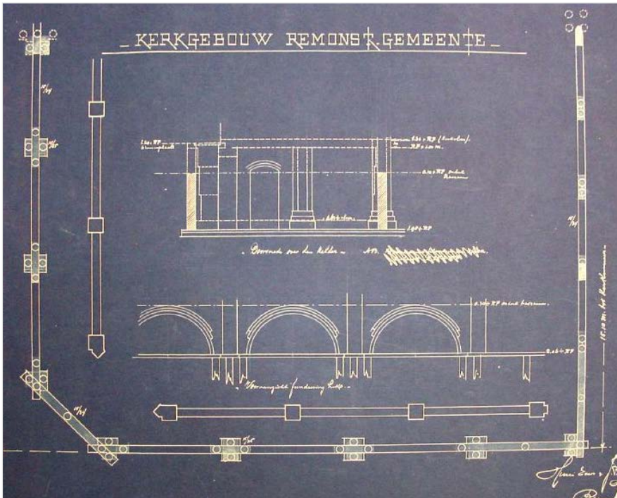
Fundering van de hekwerken rondom het voorplein, 1887. Bron: RA.
