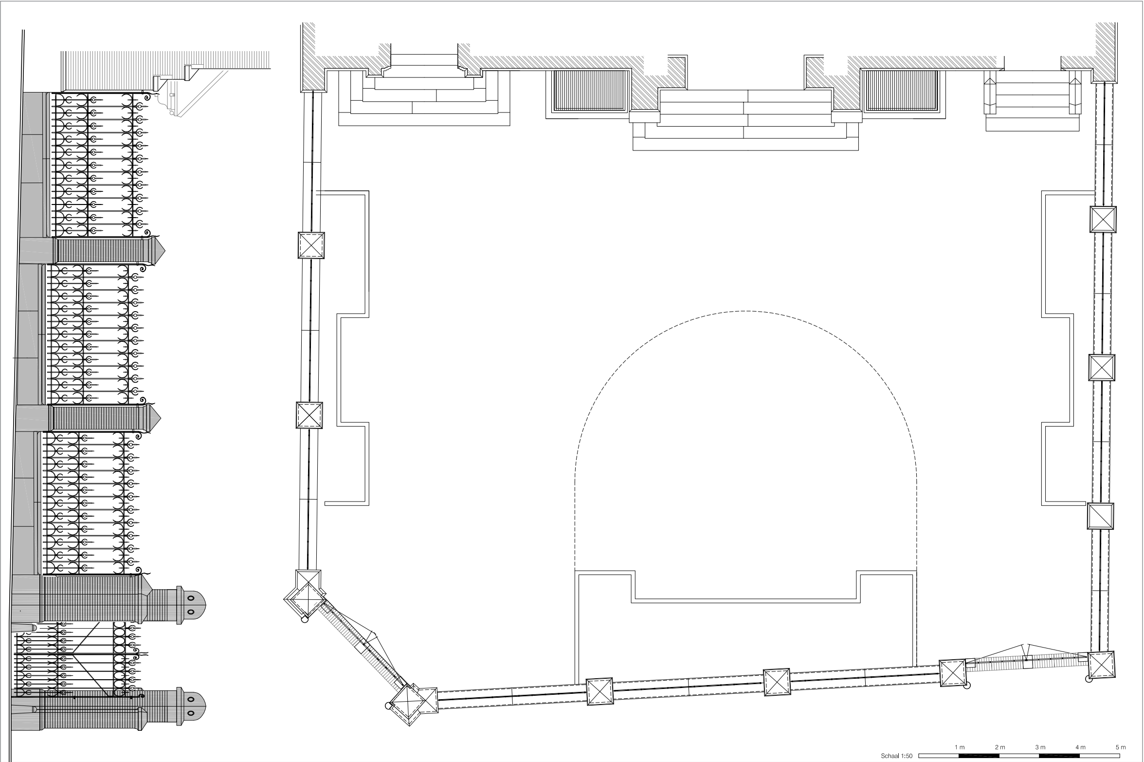
Ontwerp reconstructie hekwerk
