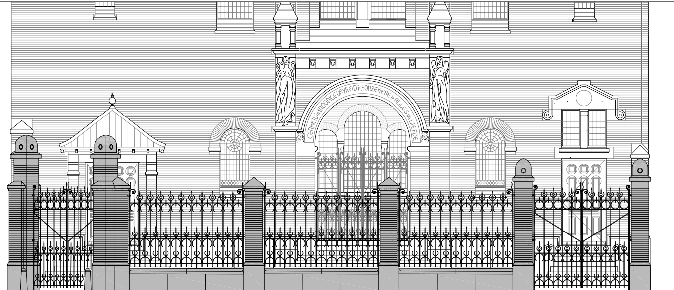
Ontwerp reconstructie hekwerk
