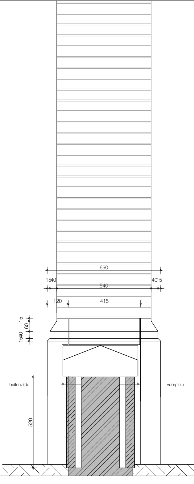
Fragment ontwerp pijler hekwerk
