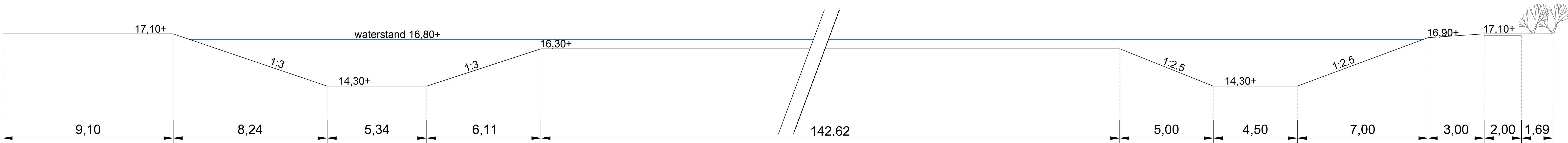
Dwarsprofiel B-B'
