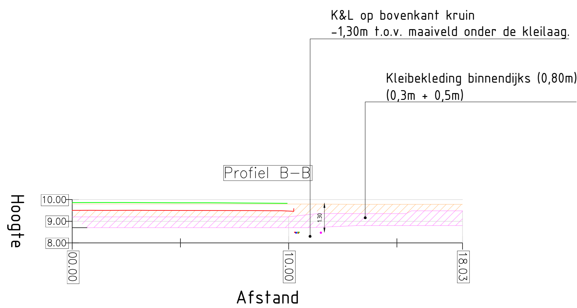
Dwarsprofiel B-B Schaal 1:100
