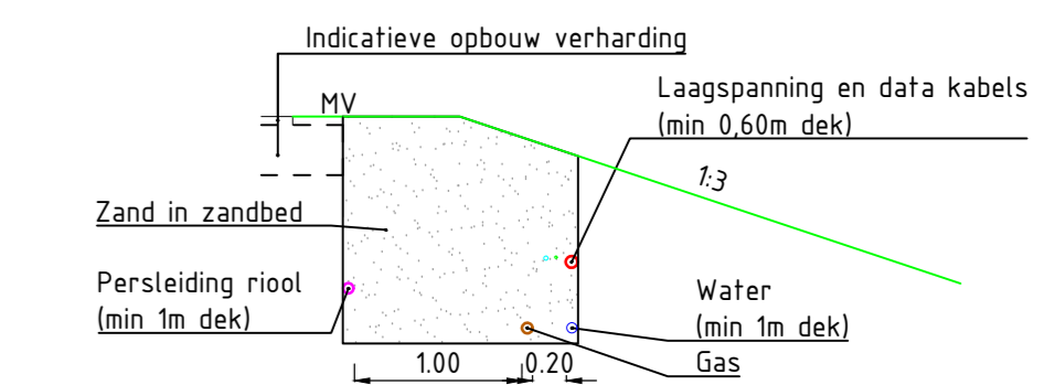
Principedetail A: k&l tracé Marconi parkeerplaatsen Schaal 1:50
