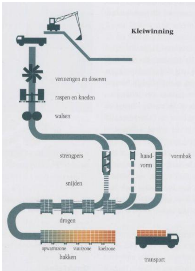
Afbeelding 2 Proces steenproductie
