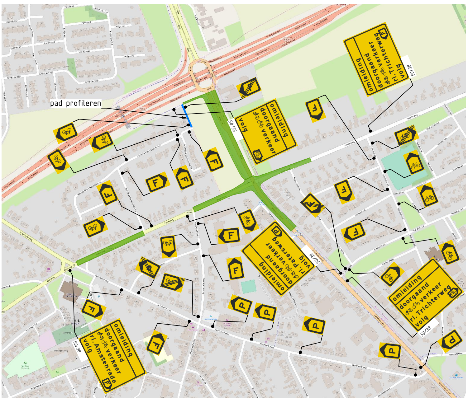
detail omleiding fase 1a & 2 t.b.v. (brom)fietssers
