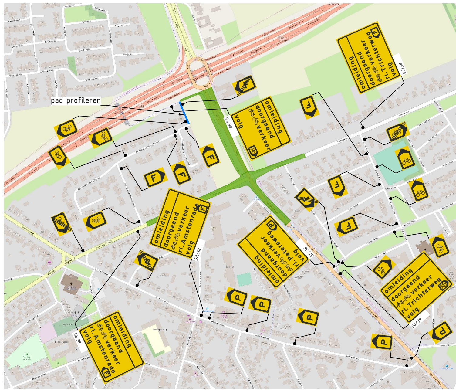
detail omleiding fase 1b t.b.v. (brom)fietssers
