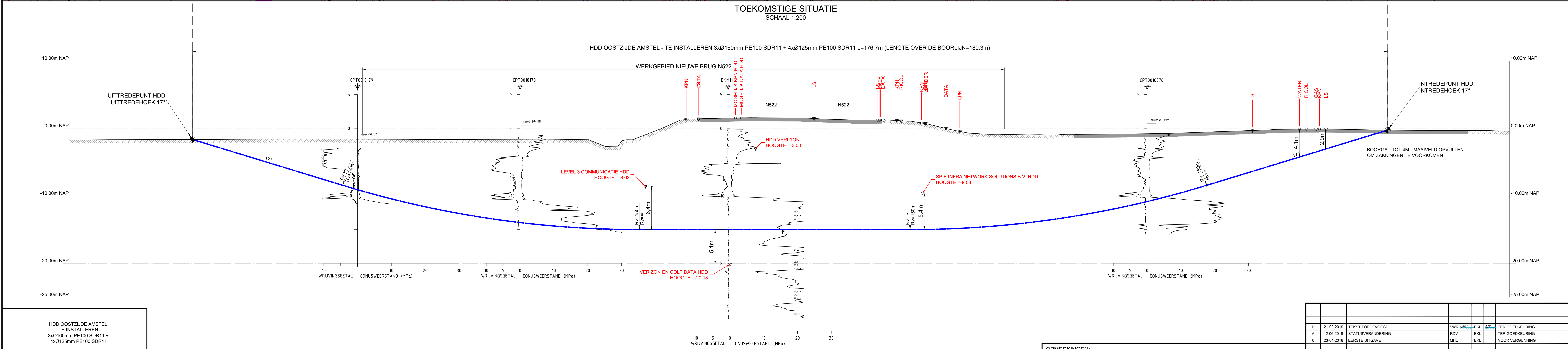
LENGTEPROFIEL HDD SCHAAL 1:200
