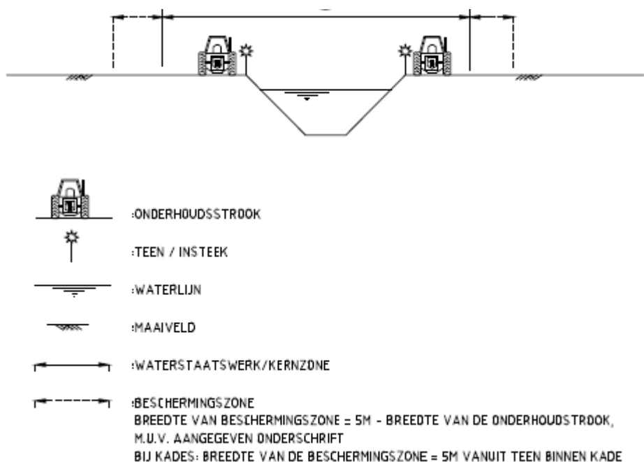
figuur 2.1 schematische weergave van de kernzone en beschermingszone van een watergang
