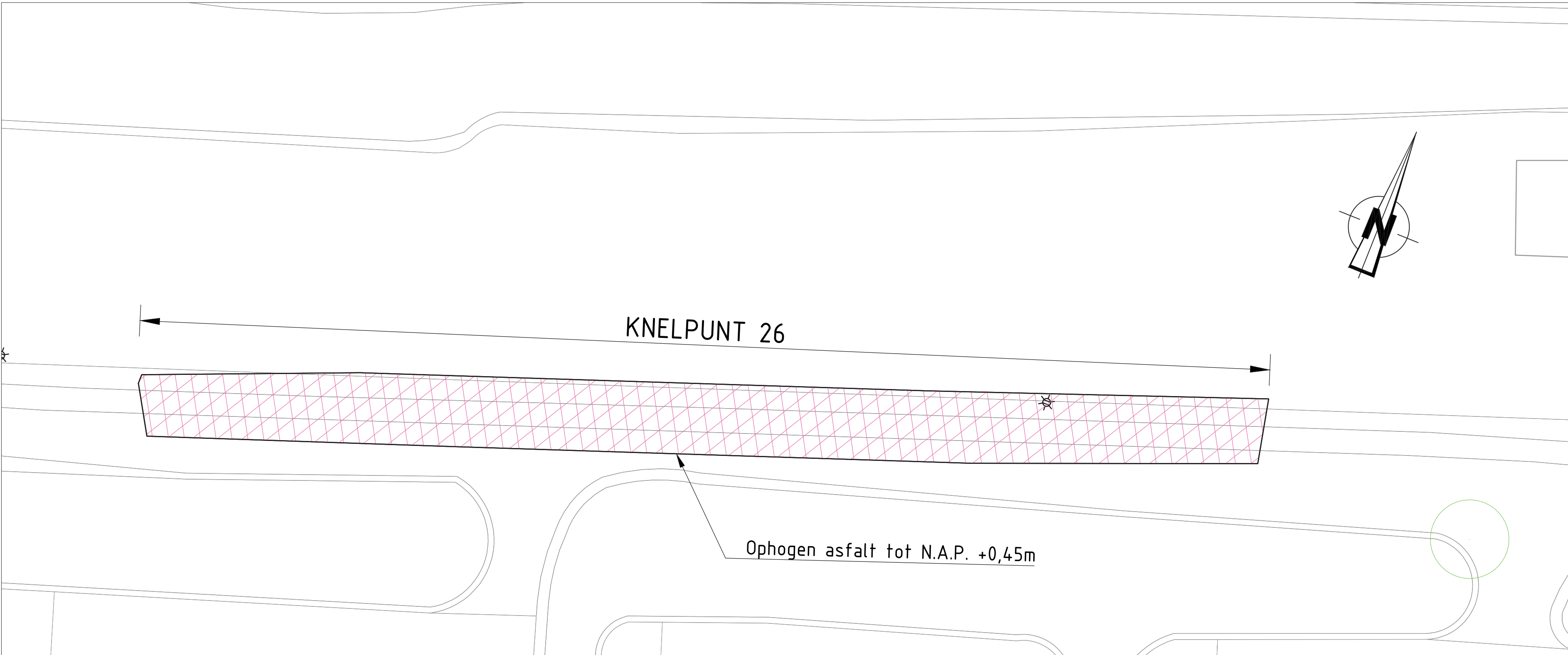
Bovenaanzicht 2 Schaal 1:200
