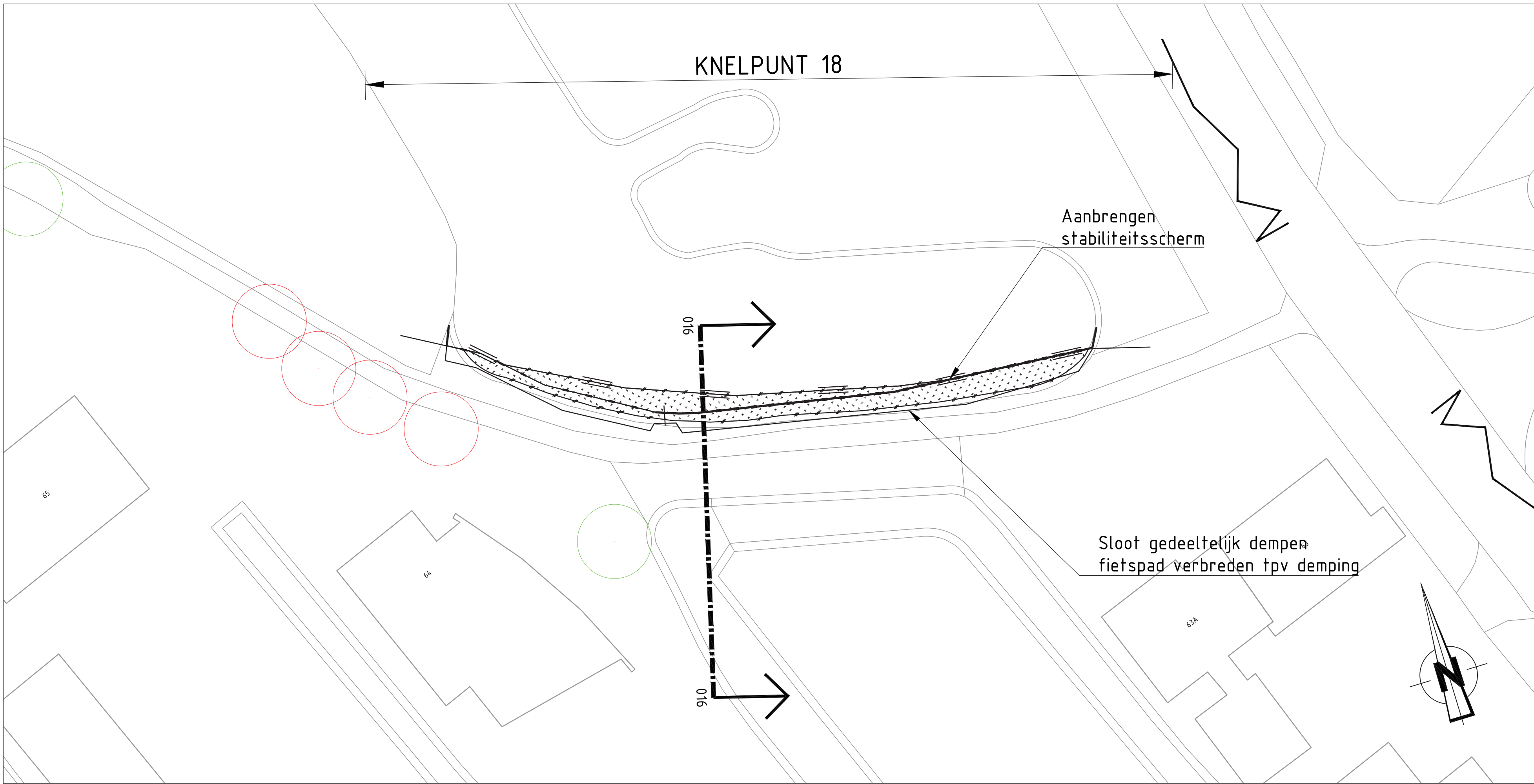
Bovenaanzicht 1 Schaal: 1:200
