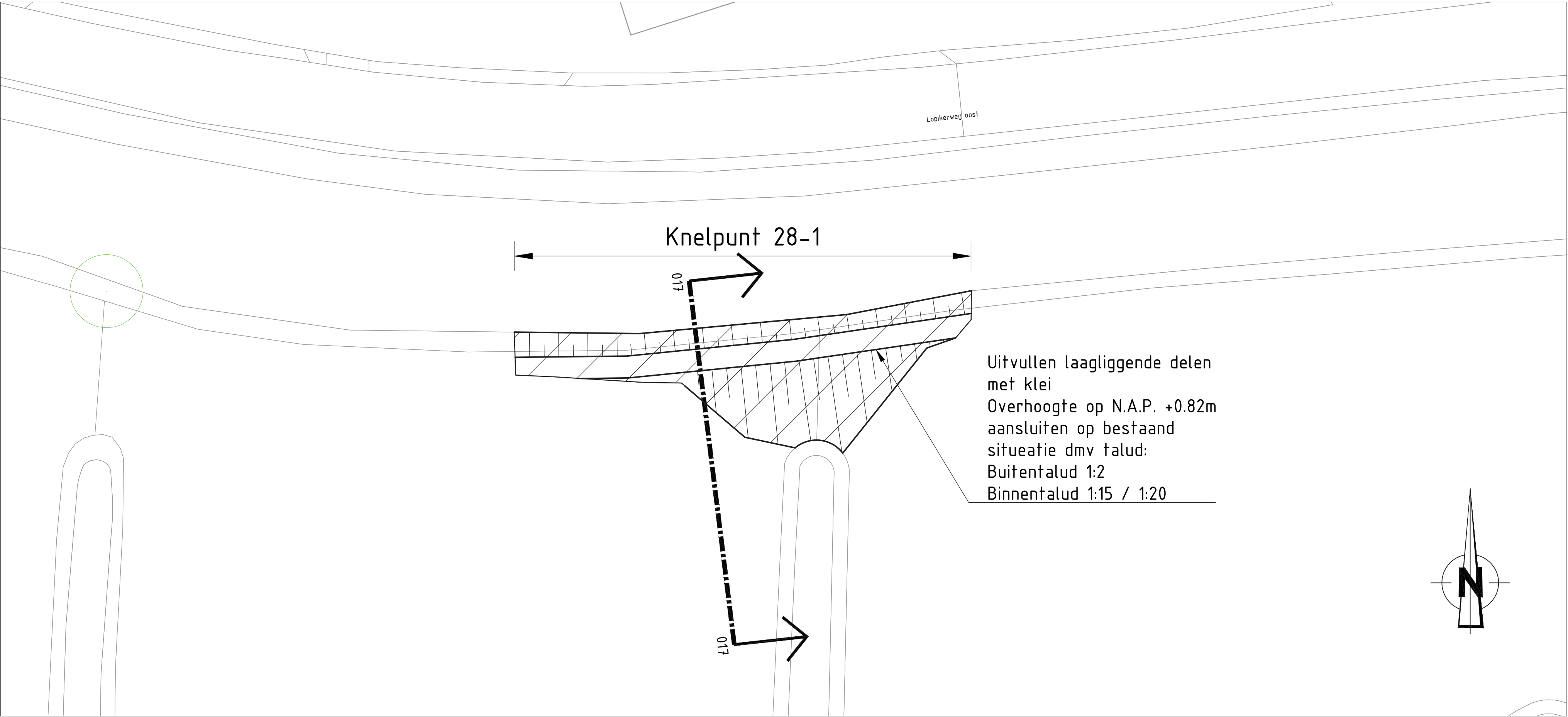
Bovenaanzicht 1 Schaal 1:200
