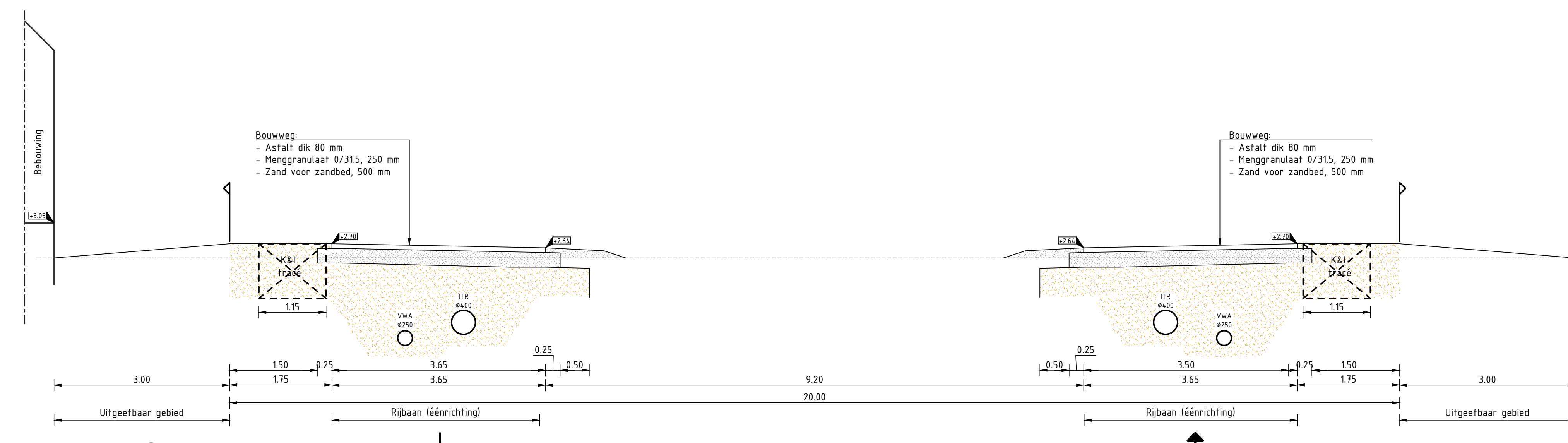
DOORSNEDE 5 SCHAAAL 1 : 50 Blad 05
