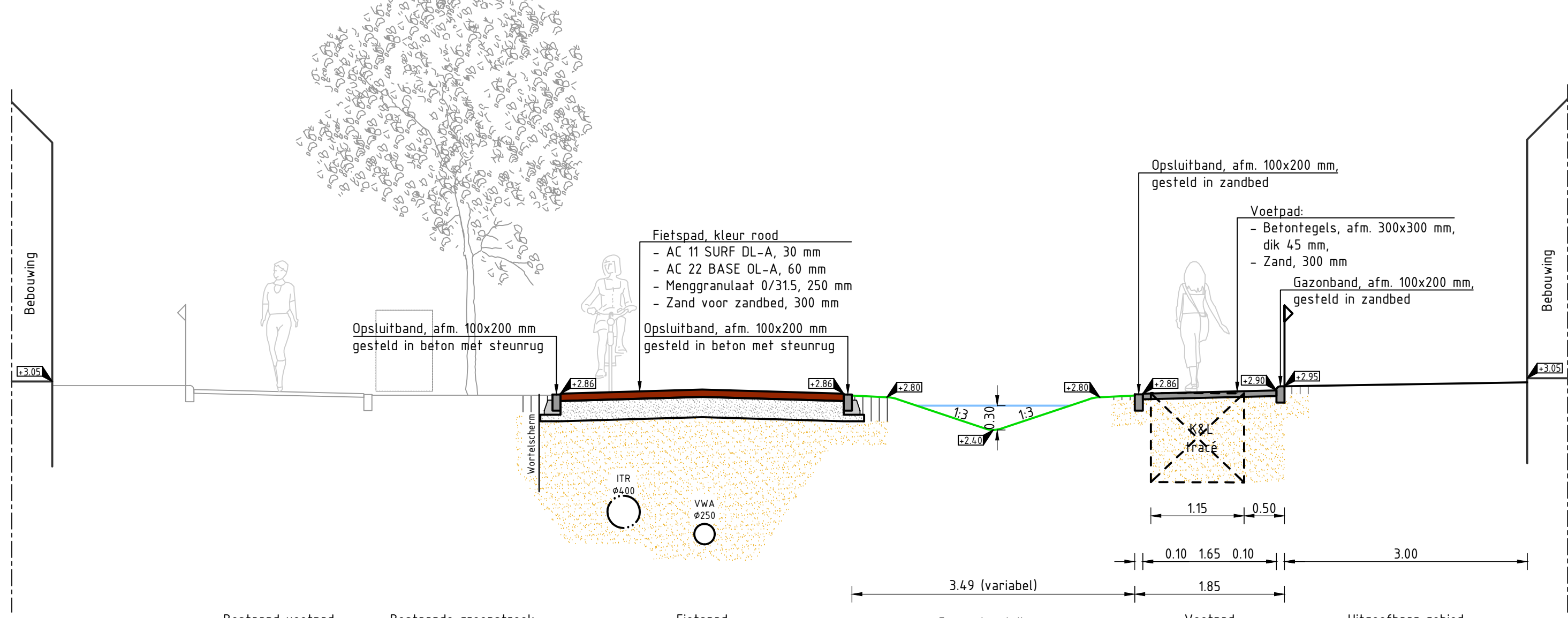
DOORSNEDE 2 SCHAAAL 1 : 50 Blad 02
