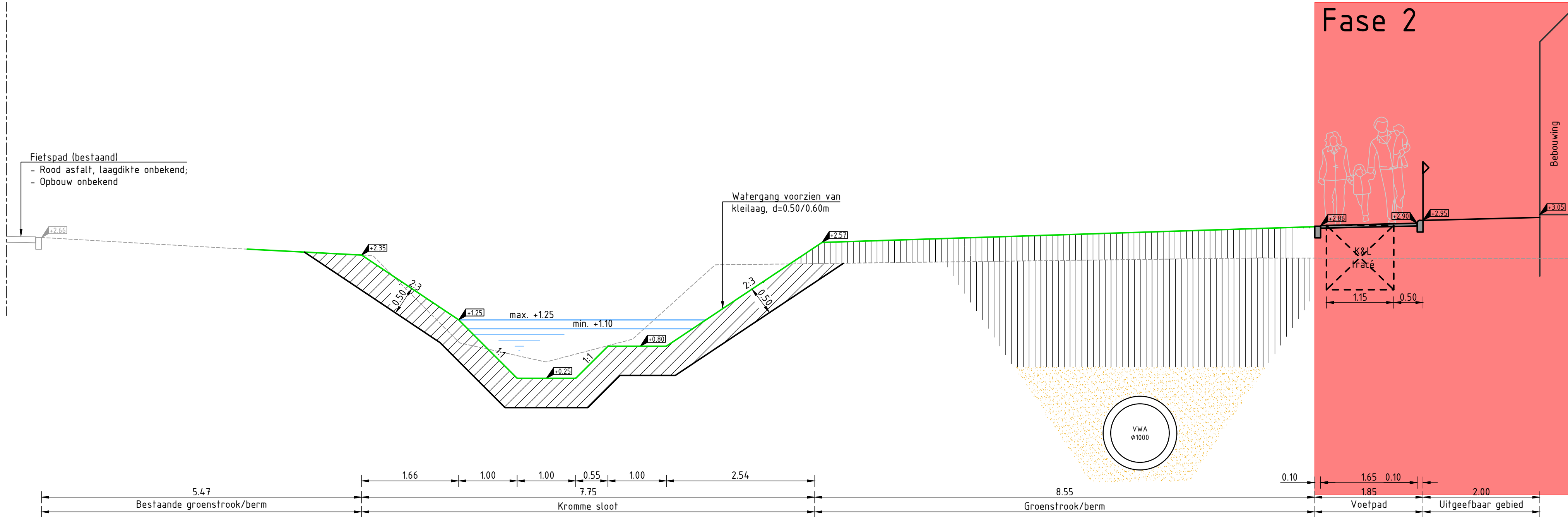
DOORSNEDE 4 SCHAAAL 1 : 50 Blad 04
