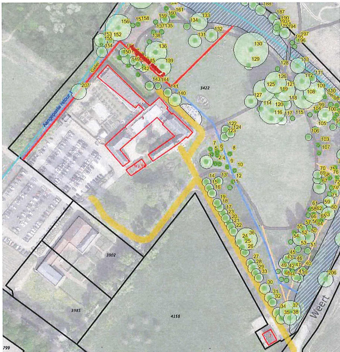
Afbeelding 1; Aangepaste retourleiding.
