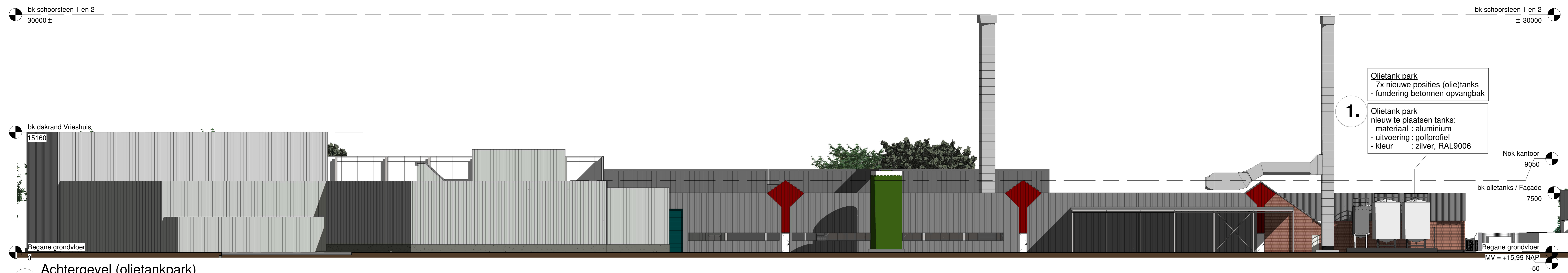
3 Achtergevel (olietankpark) 1 : 200
