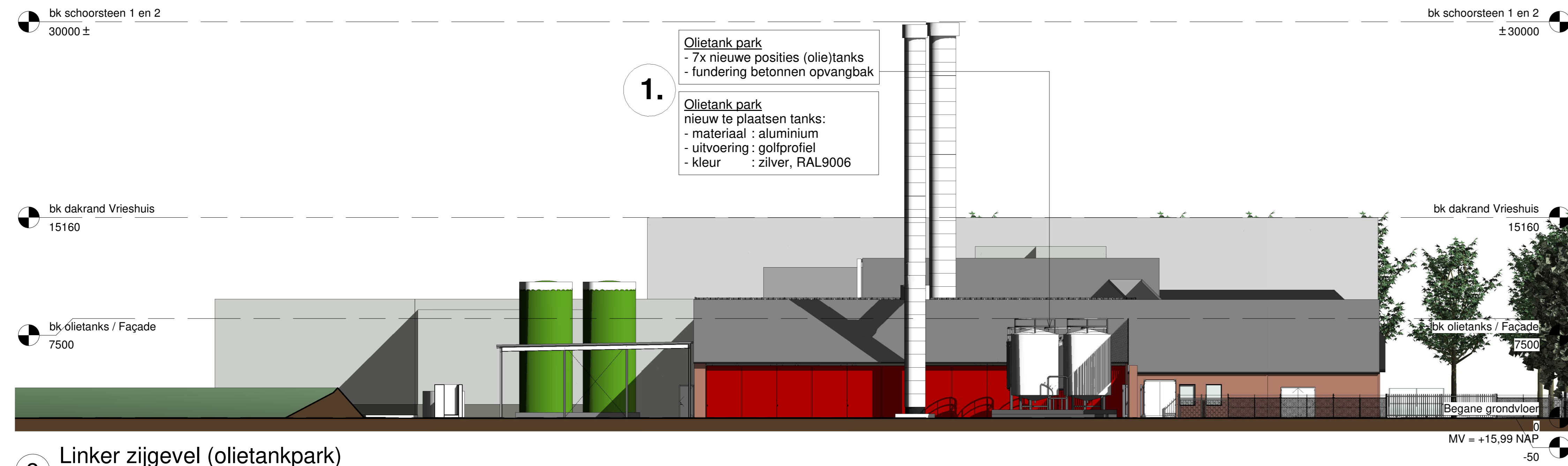
2 Linker zijgevel (olietankpark) 1 : 200
