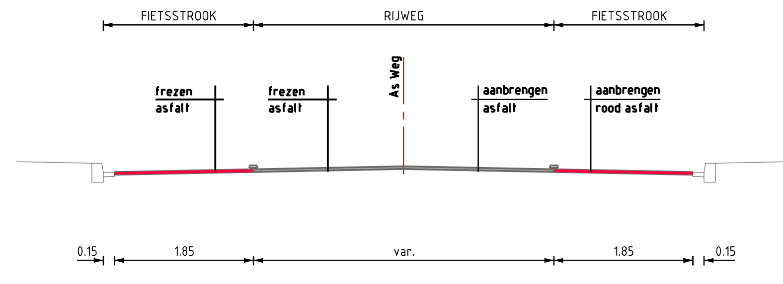
Principe dwarsprofiel schaal 1 : 50
