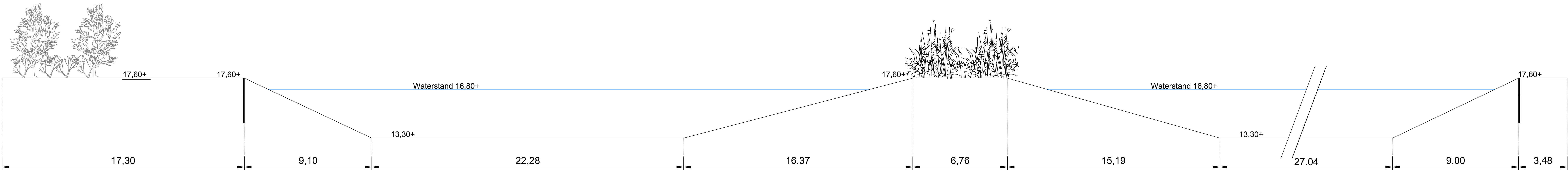
Dwarsprofiel C-C'
