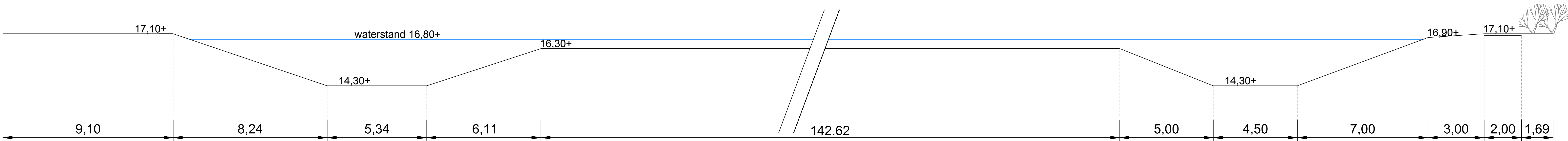
Dwarsprofiel B-B'
