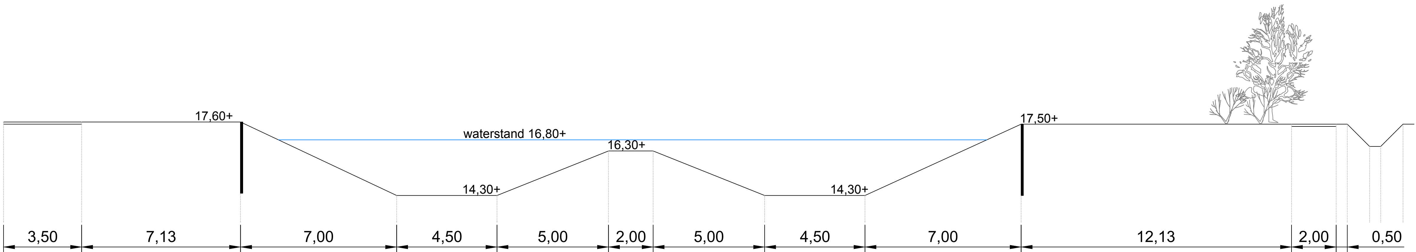
Dwarsprofiel A-A'
