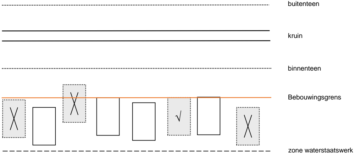
Figuur 37.2: Plaatsen van bouwwerken -nieuwbouw en aanbouw- in de zone waterstaatswerk bij regionale waterkeringen en overige waterkeringen (bovenaanzicht)
