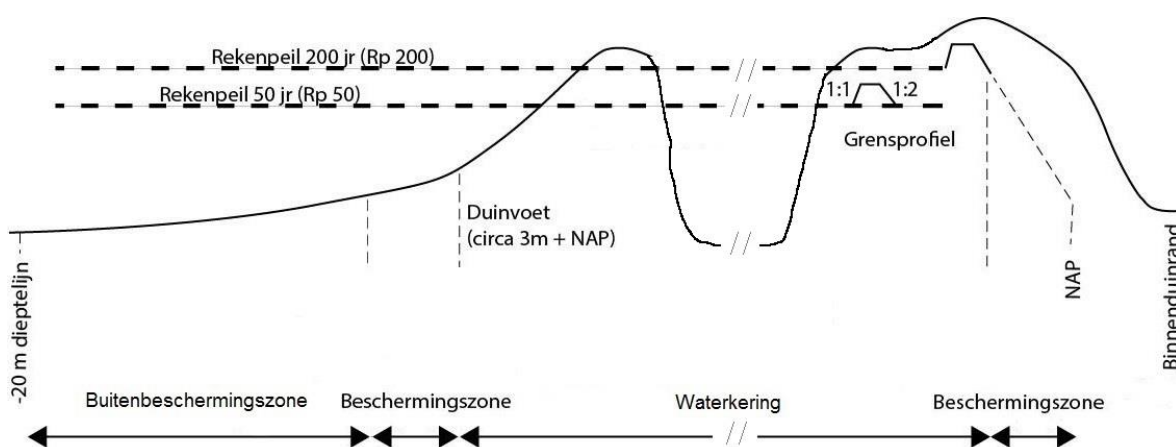
Figuur 7. Zonerings behorende bij de brede primaire duinwaterkering
