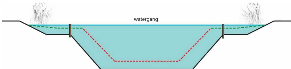
Figuur 2d. Toelichting: Bovenstaande afbeelding is een voorbeeld van een watergang met een natuurvriendelijke oever, die ruim voldoende diepte en breedte heeft. Het integrale profiel is kleiner als het feitelijk aanwezige profiel.
