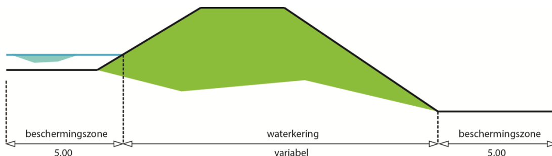
Figuur 12: Zonering behorende bij de regionale waterkering
