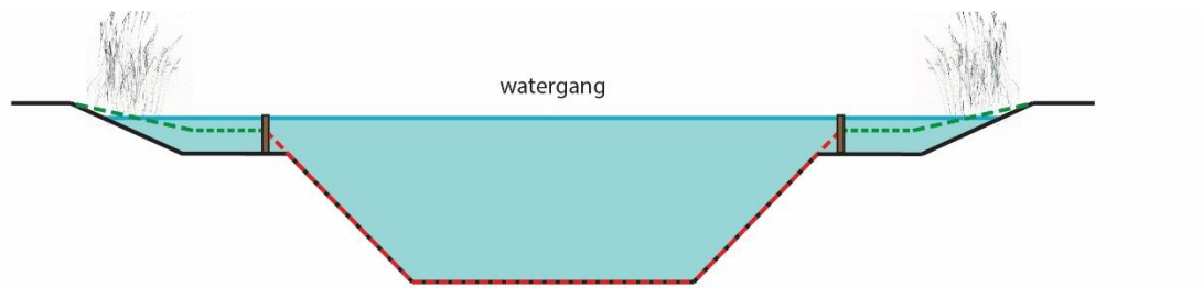
Figuur 2b. Toelichting: Bovenstaand is een voorbeeld van een watergang met een natuurvriendelijke oever. Het integrale profiel komt overeen met feitelijk aanwezige profiel.
