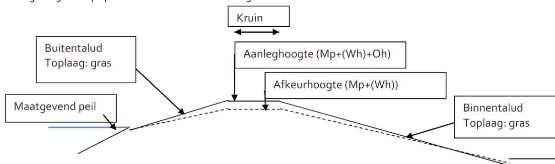
Figuur 13: Principe profiel van een lokale waterkering
