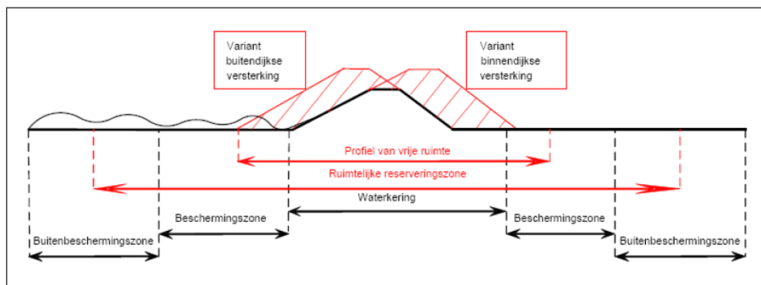
Figuur 6: principetekening zonerings primaire waterkering
