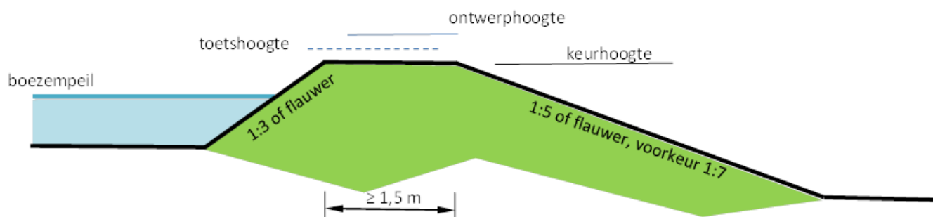
Figuur 11: principe profiel polderdijk
