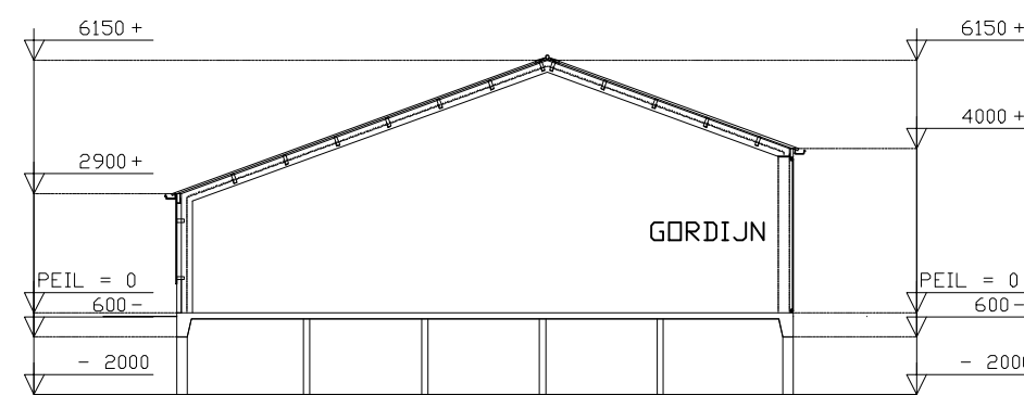
DOORSNEDE STAL 2
