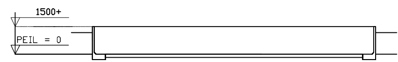
DOORSNEDE OPSLAG VASTE MEST
