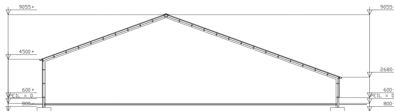
DOORSNEDE STAL 3
