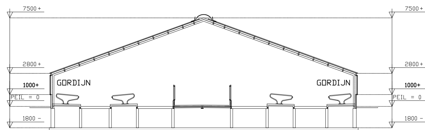
DOORSNEDE STAL 1
