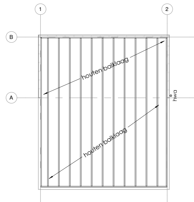
KAPPLAN
