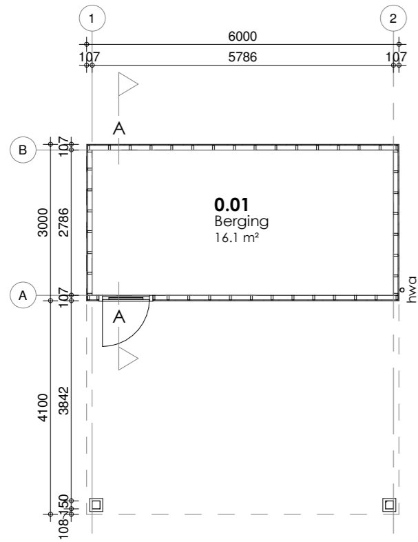
BEGANE GROND
