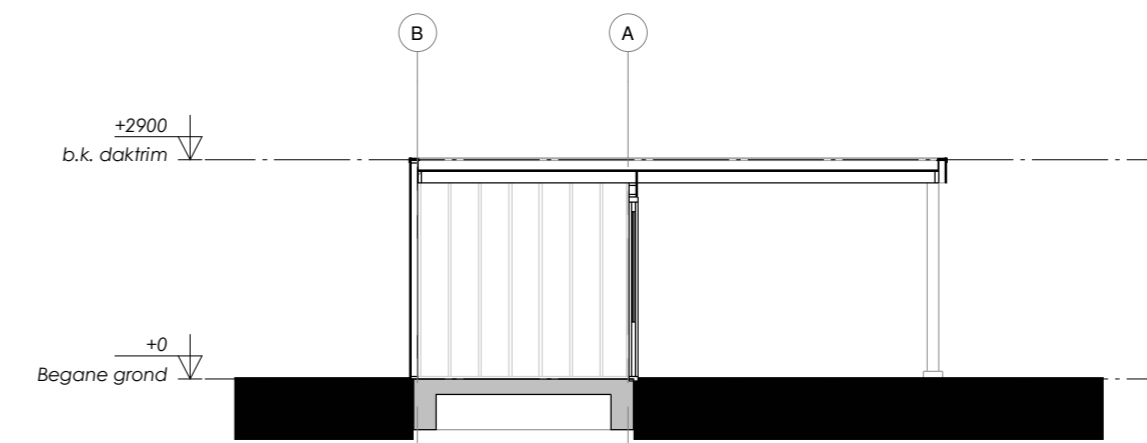
DOORSNEDE A-A
