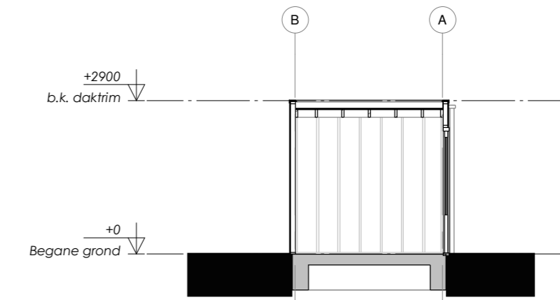
DOORSNEDE A-A
