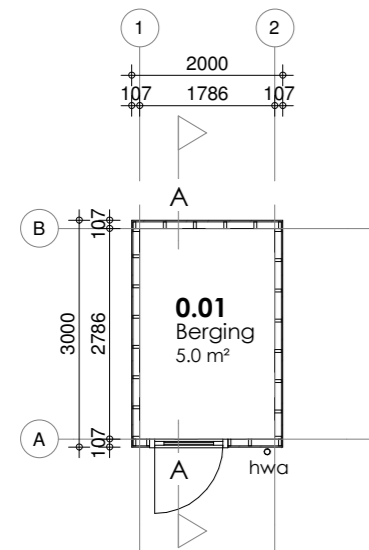
BEGANE GROND
