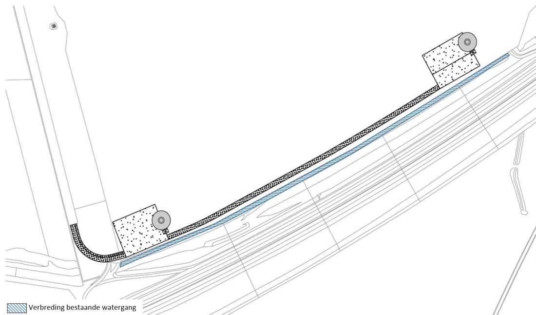
Figuur 3.2 Watercompensatielocatie tussen windturbines 1 en 2.
