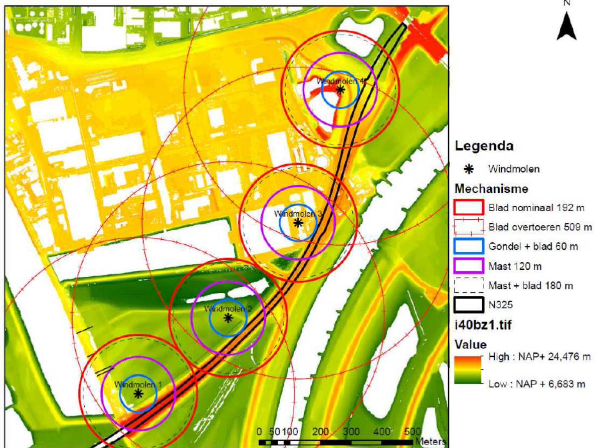
Figuur 2.1 overzicht invloedsgebieden per faalmechanisme windturbine
