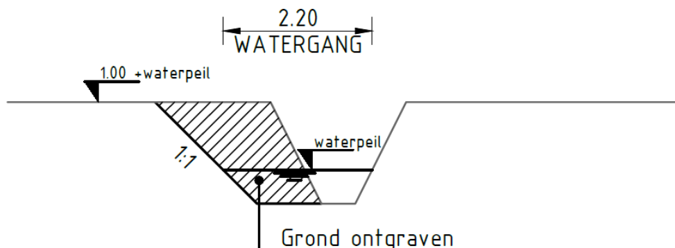
Figuur 3.3 Principeprofiel te verbreden watergang tussen windturbines 1 en 2.
