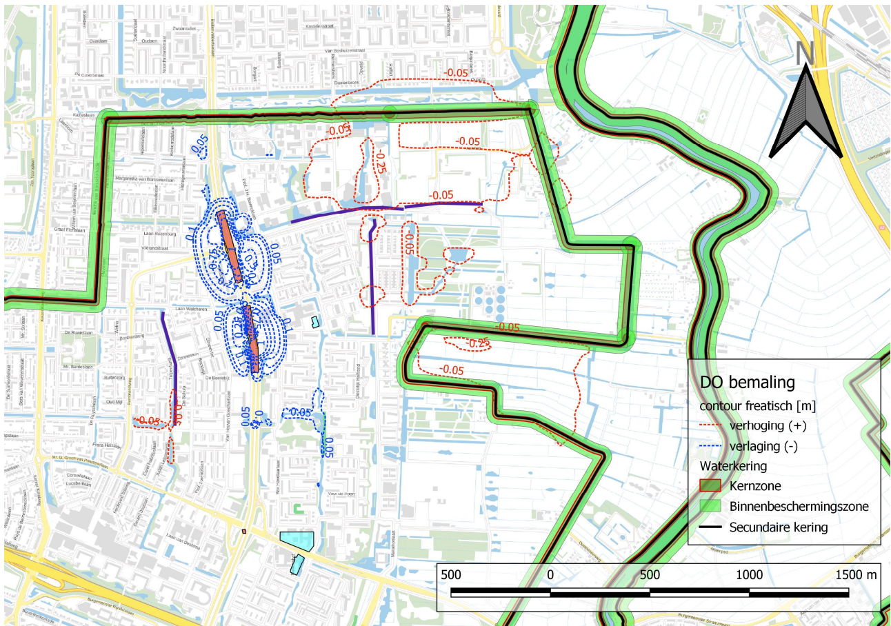
Figuur 40. Verlagingcontouren in veenlaag en omgevingseffecten
