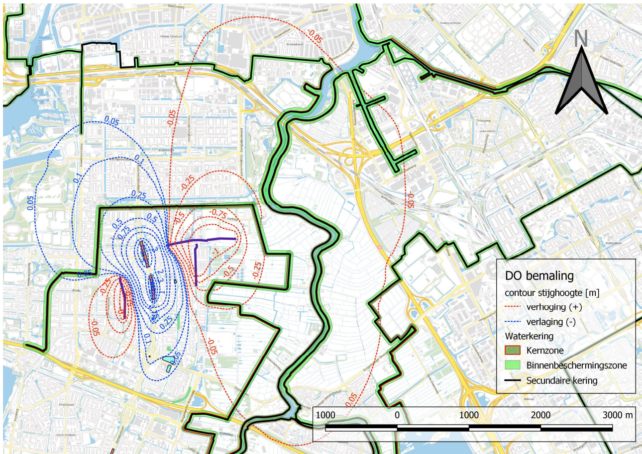
Figuur 42. Verlagscontouren in 1 e WVP en omgevingseffecten..
