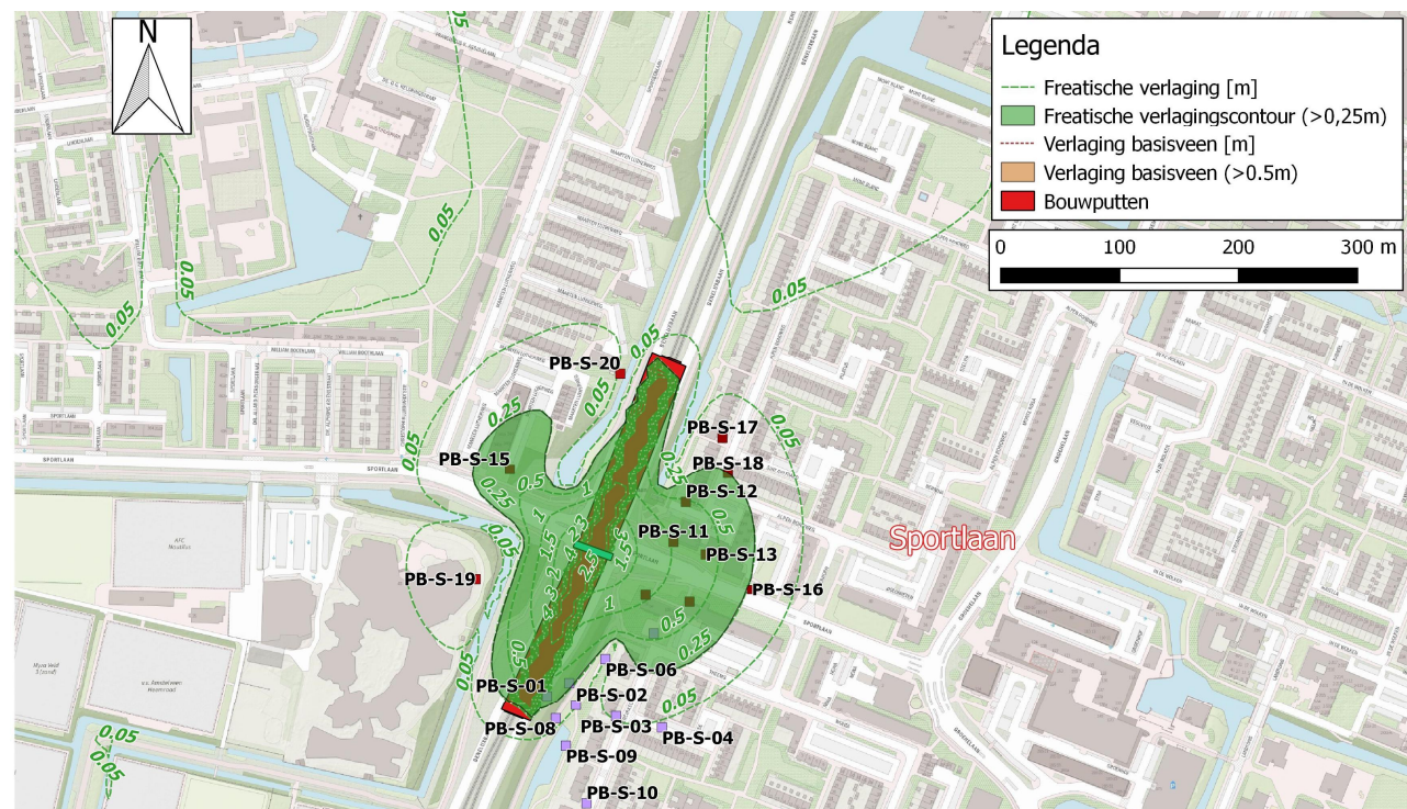
Figuur 49. Verlagsingscontouren (freatisch) en in groen de arcering waarbinnen mogelijk grondwaterstand verder verlaagd wordt dan de signaalwaarde. Hiervoor zijn monitoringspeilbuizen gezet om dit nader te monitoren (paars=locatie monitoringspeilbuizen). Zie hoofdstuk 7.1.1 en 8 voor nadere informatie.
