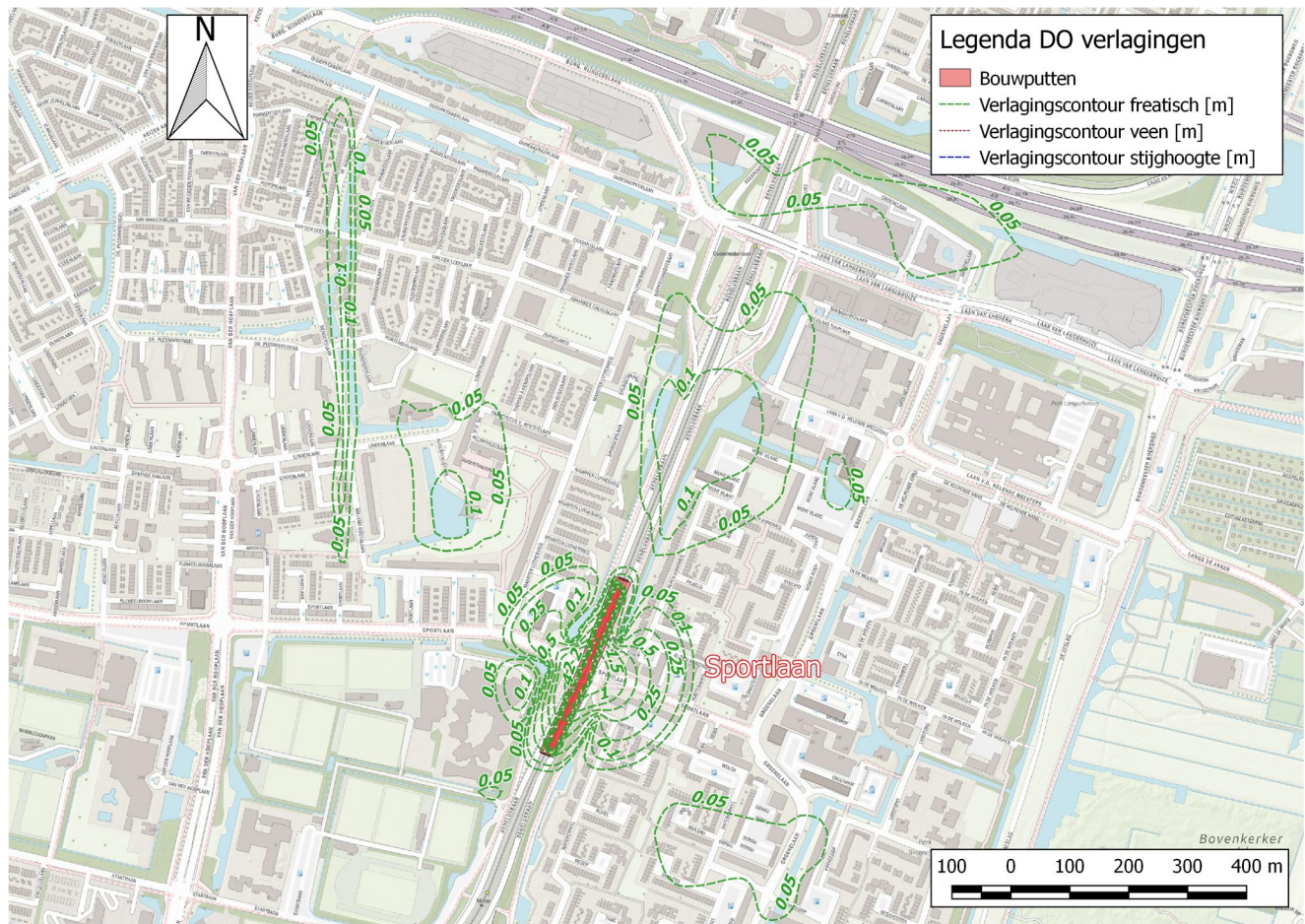
Figuur 31. Verlagsingscontouren Sportlaan in de kleilaag (freatisch). Inclusief bemaling waterkelder.
