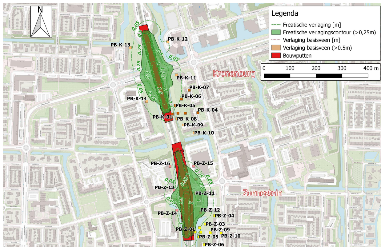
Figuur 43. Verlagscontouren (freatisch) en in groen de arcering waarbinnen mogelijk grondwaterstand verder verlaagd wordt dan de signaalwaarde. Hiervoor zijn monitoringspeilbuizen gezet om dit nader te monitoren (oranje/geel=locatie monitoringspeilbuizen). Zie hoofdstuk 7.1.1 en 8 voor nadere informatie.
