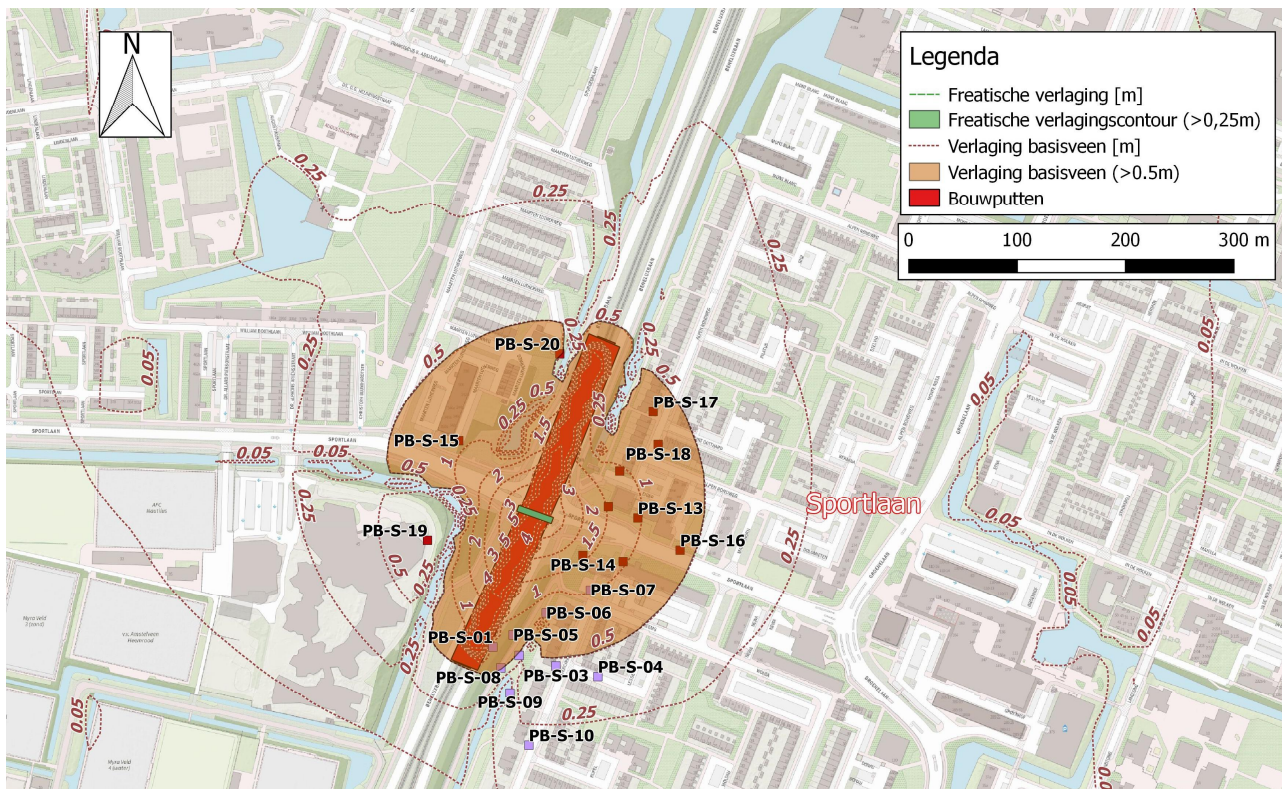
Figuur 50. Verlagingcontouren (veen) en in bruin de arcering waarbinnen mogelijk grondwaterstand verder verlaagd wordt dan de signaalwaarde. Hiervoor zijn monitoringspeilbuizen gezet om dit nader te monitoren (paars=locatie monitoringspeilbuizen). Zie hoofdstuk 7.1.1 en 8 voor nadere informatie.
