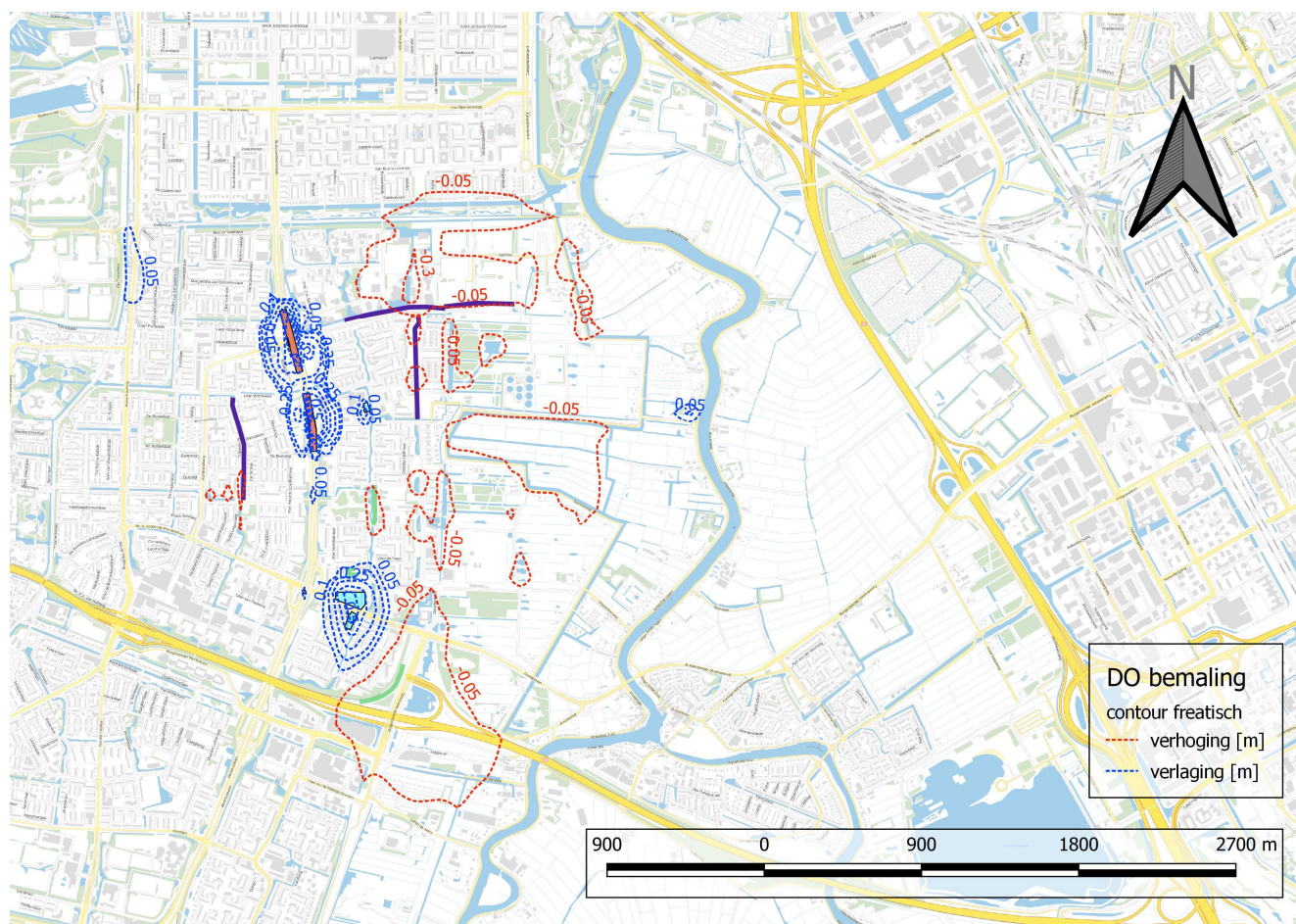
Figuur 21. Freatische verlagingcontouren.
