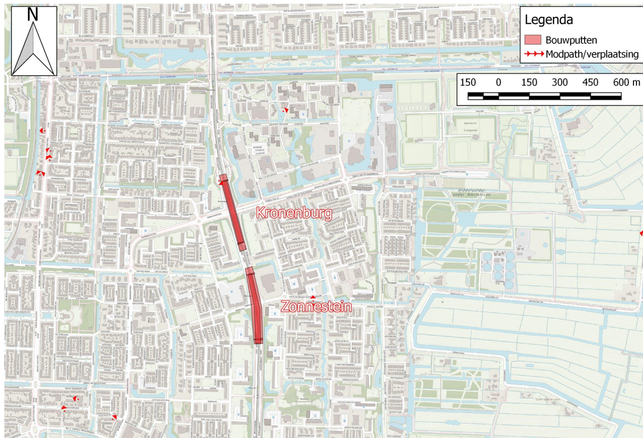
Figuur 52. Verplaatsing verontreiniging. De peil geeft de richting van de verplaatsing aan. De verplaatsing is minimaal, tussen 1,2 en 5,0 m.
