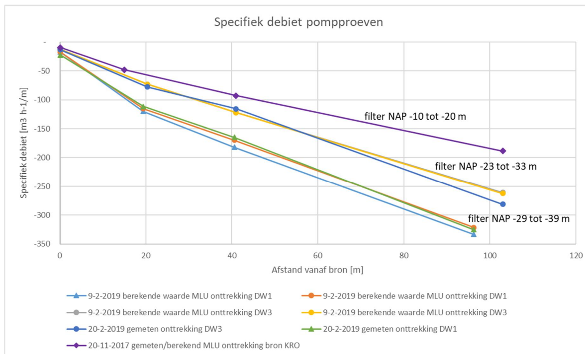
Figuur 71 Specifiek debiet en verlaging
