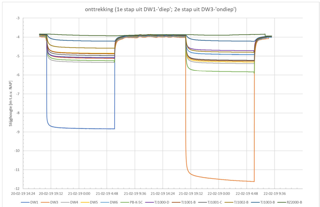
Figuur 66 Gemeten stijghoogtes 20 tot 22 november 2019 (Tjaden)
