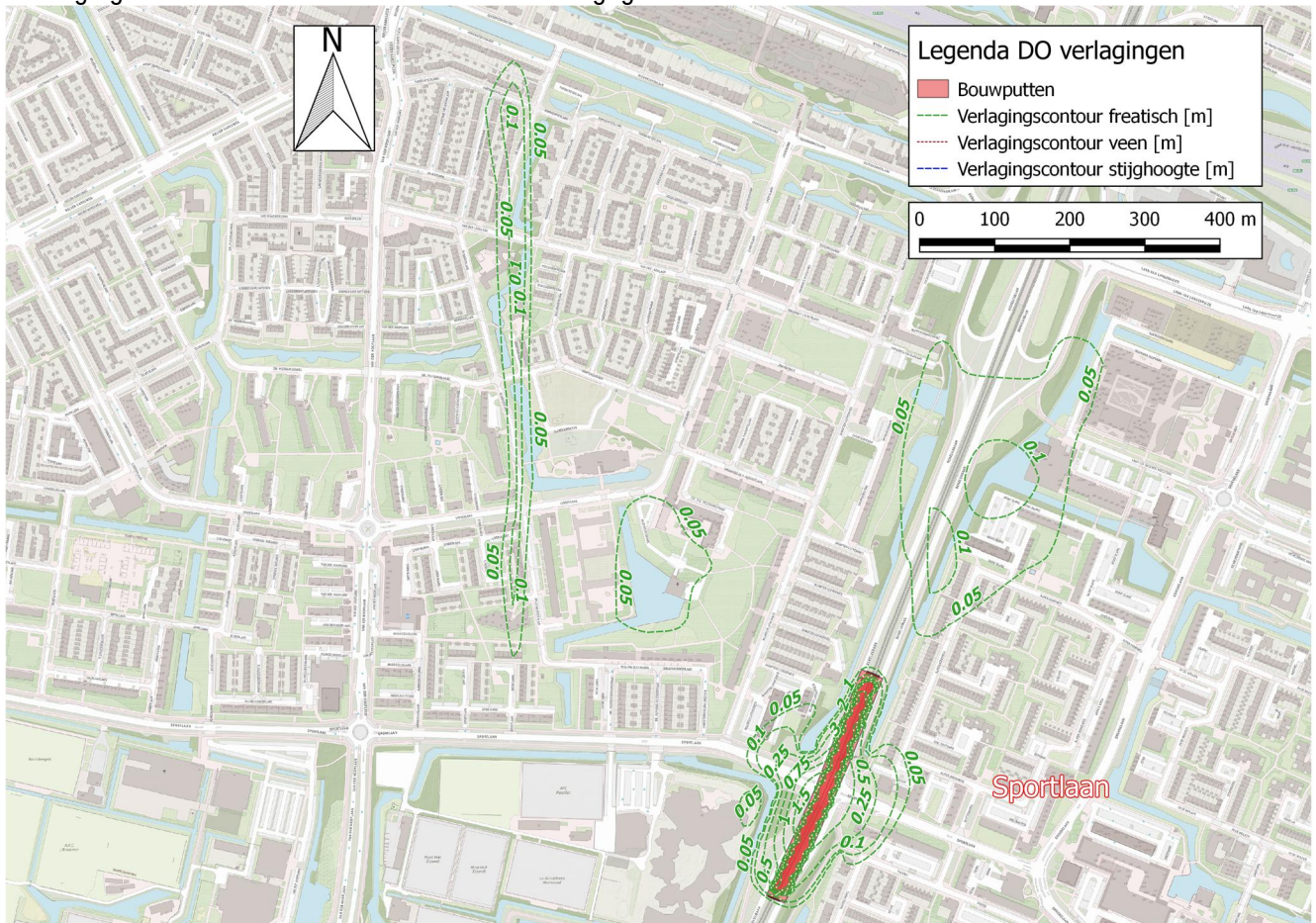
Figuur 28. Freatische verlagingscontouren. Deze contouren weergeven het effect zonder bemaling van de waterkelder.
