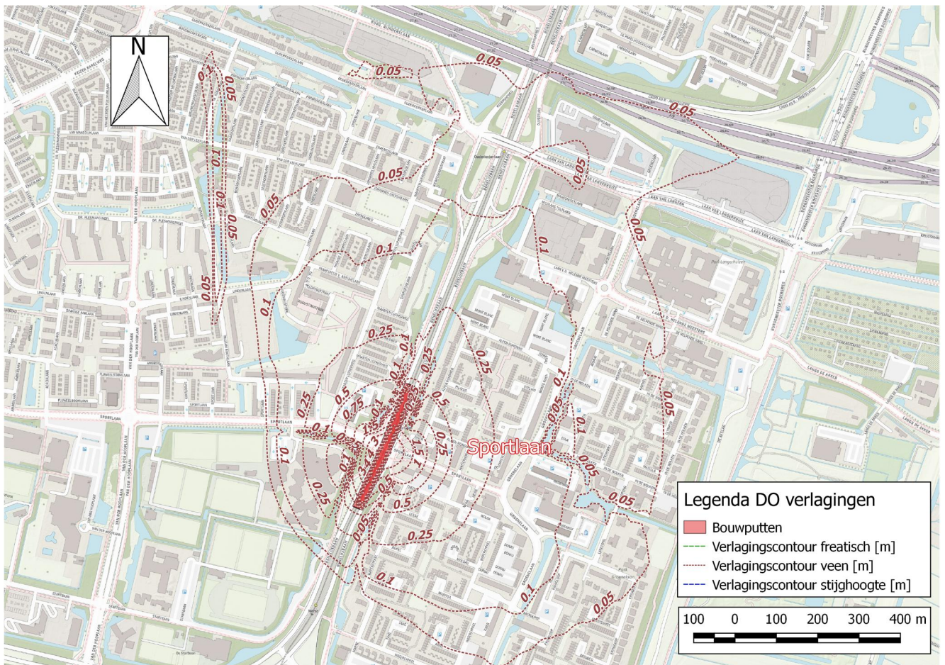
Figuur 32. Verlagingscontouren Sportlaan in de basisveenlaag. Inclusief bemaling waterkelder.
