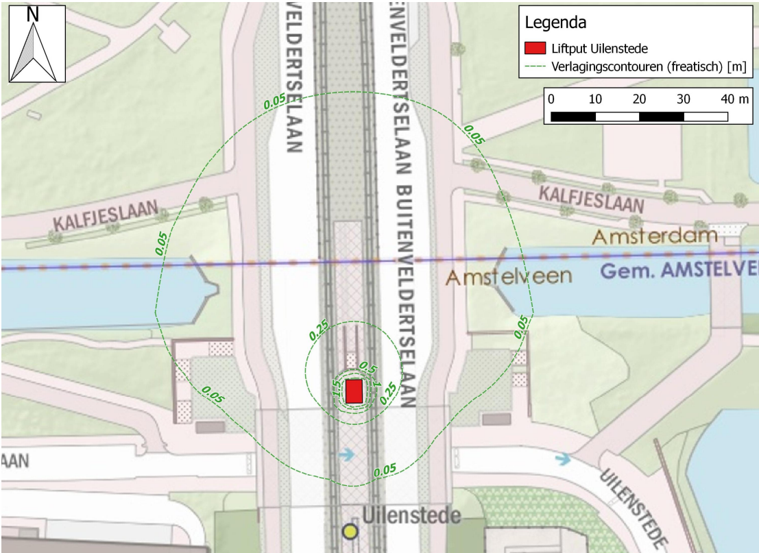
Figuur 26. Freatische verlagingscontouren Uilenstede.
