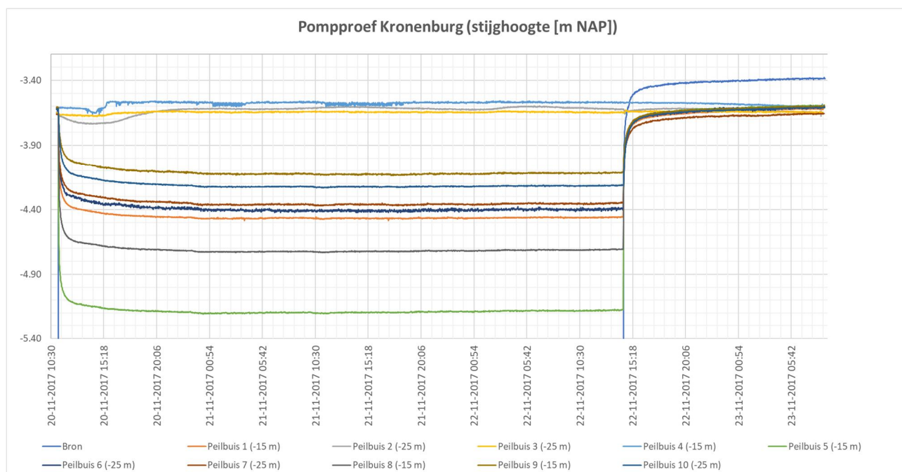
Figuur 56. Verlaging stijgheogte pompproef Kronenburg (stijgheogte in bron is NAP -8,3 m).
