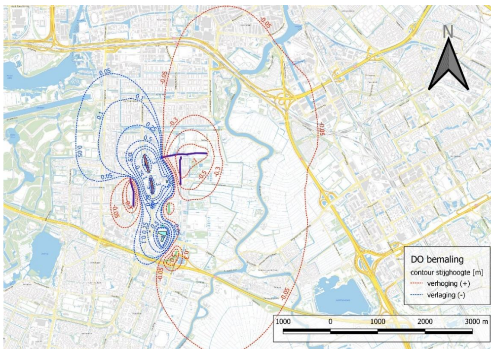
Figuur 3 – Verlagingen [+] en verhogingen [-] in het 1 e wvp bij VDL Kronenburg en Zonnestein (situatie bemaling tijdens zomer TBGN inclusief raakvlak met omliggende bemalingen Straat van Messina 10, Klaasje Zeversterstraat 1 en Bankrashof 3)
