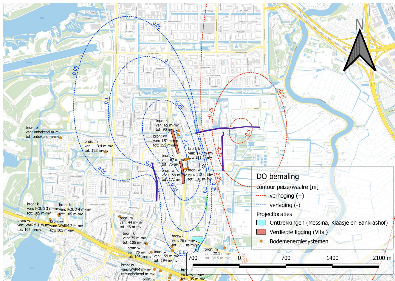
Figuur 14 Verlagscontouren Kronenburg/Zonnestein in het Peize Waalre zand (zandpakket waar WKO systemen aanwezig zijn). Enkele systemen liggen binnen de verhogingscontouren en verlagingcontouren
