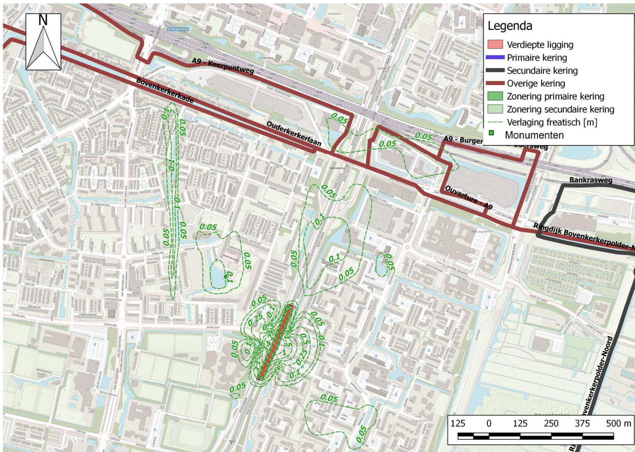
Figuur 45. Omgevingseffecten freatische verlaging.
