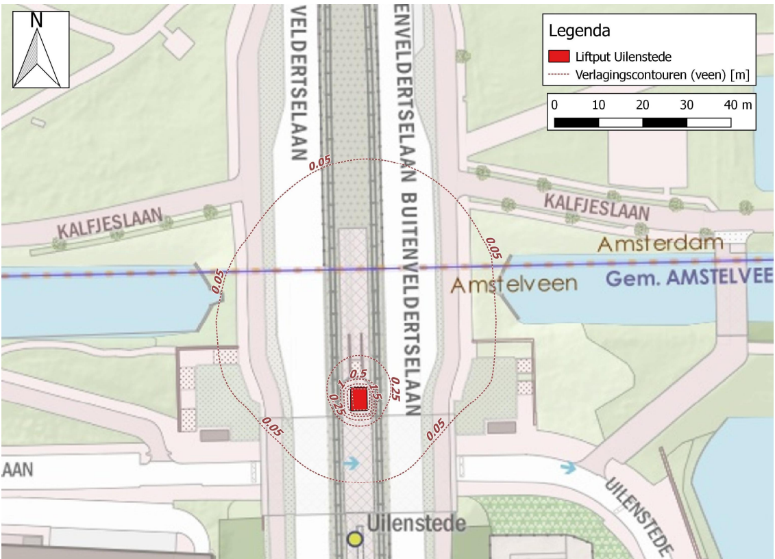
Figuur 27. Verlagingscontouren in de veenlaag tijdens liftwerkzaamheden halte Uilenstede.
