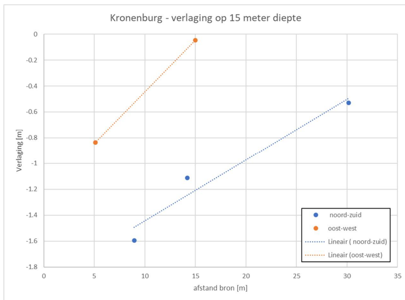
Figuur 57. Waarneming anisotropie op 15 m-mv nabij Kronenburg.
