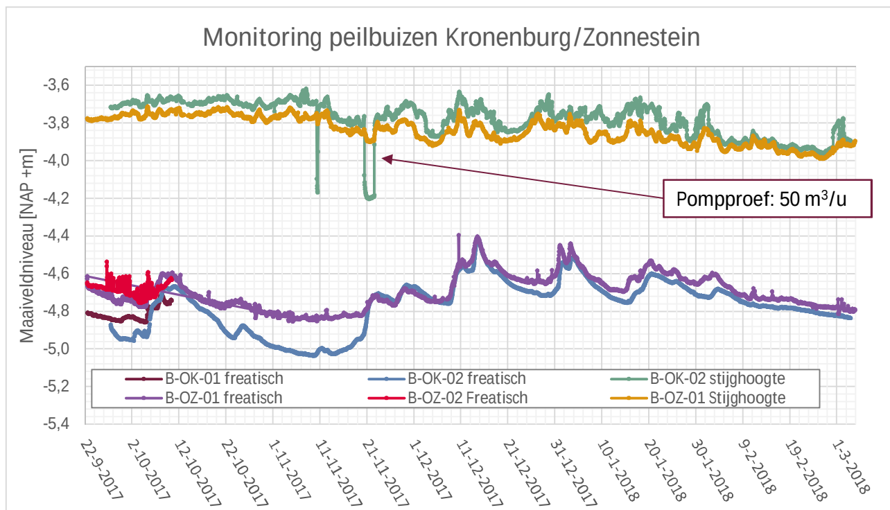
Figuur 73. Fluctuatie grondwaterstanden Kronenburg (OK) en Zonnestein (OZ) september 2017 – maart 2018
