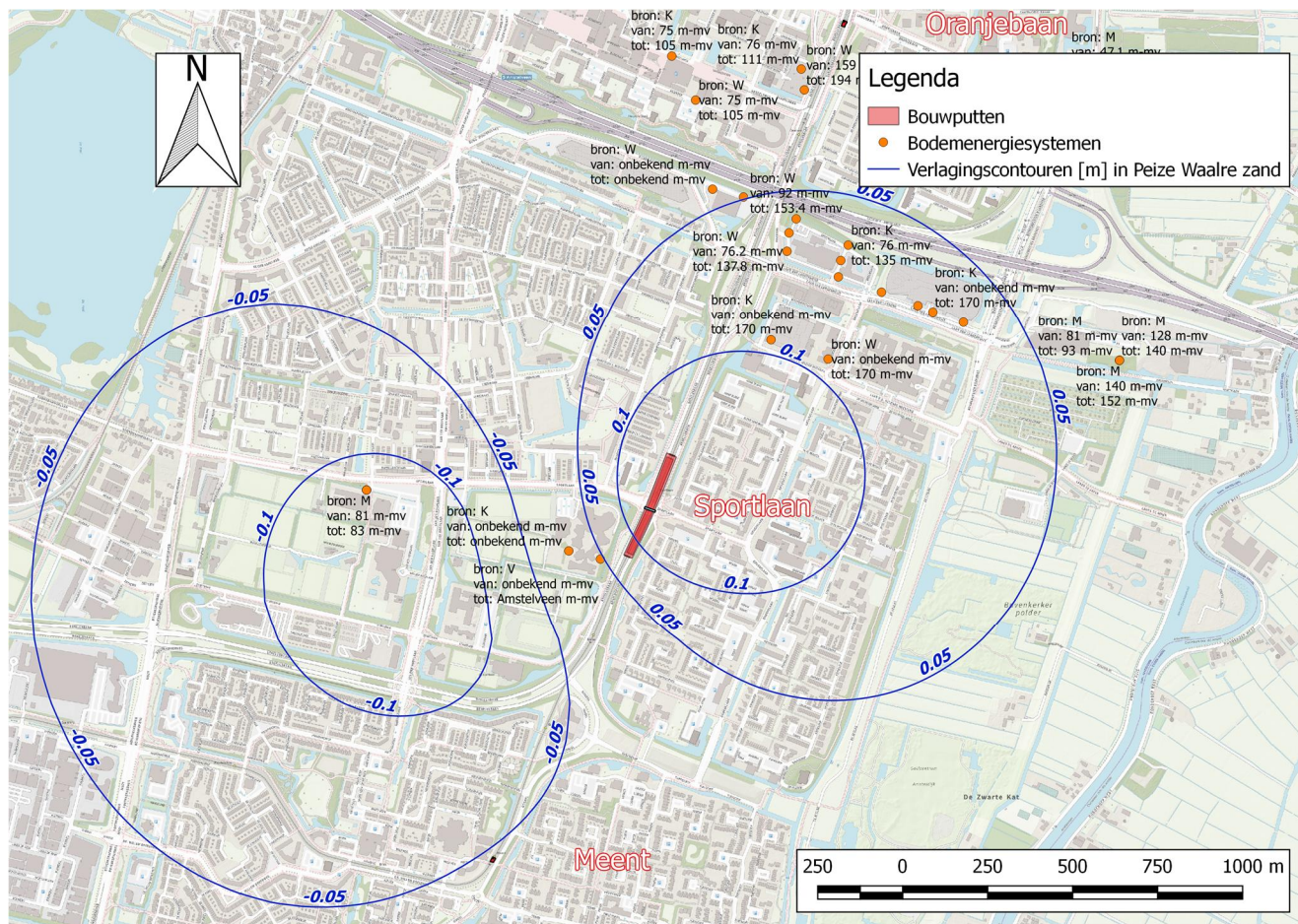
Figuur 13. Verlagscontouren Sportlaan in het Peize Waalre zand (zandpakket waar WKO systemen aanwezig zijn). Enkele systemen liggen binnen de verlagscontouren of verhogingscontouren.
