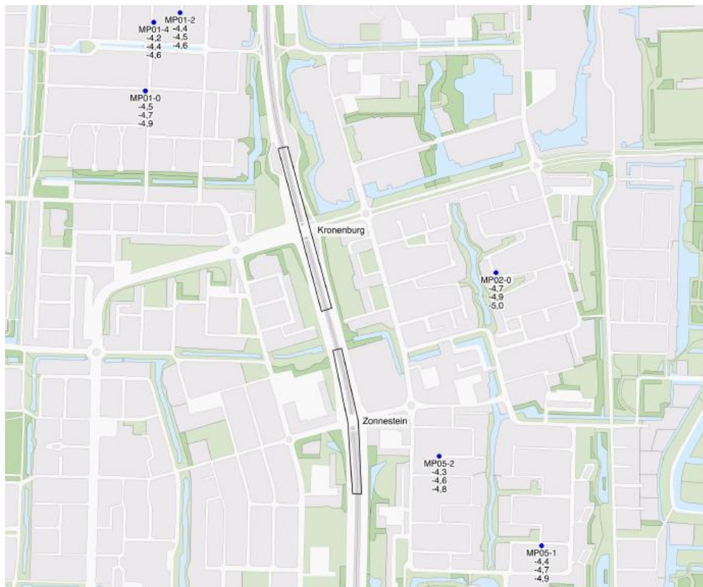
Figuur 74. Locatie peilbuizen gemeente Amstelveen.
