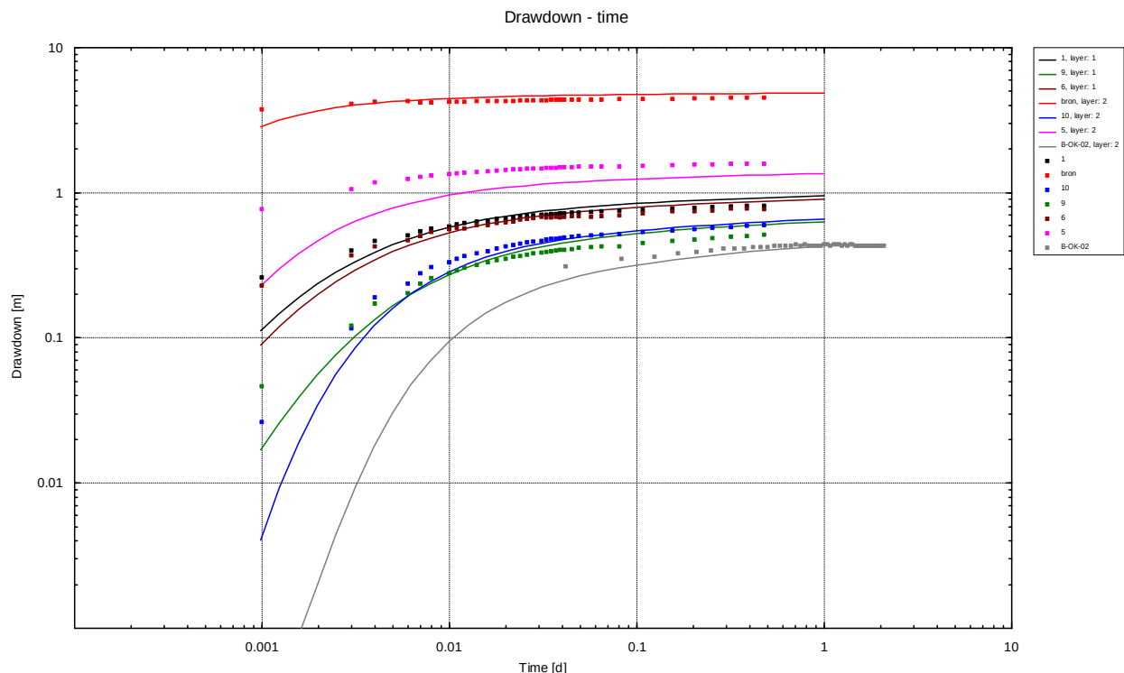
Figuur 70 Tijd versus verlaging Bron Kronenburg nov 2017 (49 m 3 /h) met MLU fit
