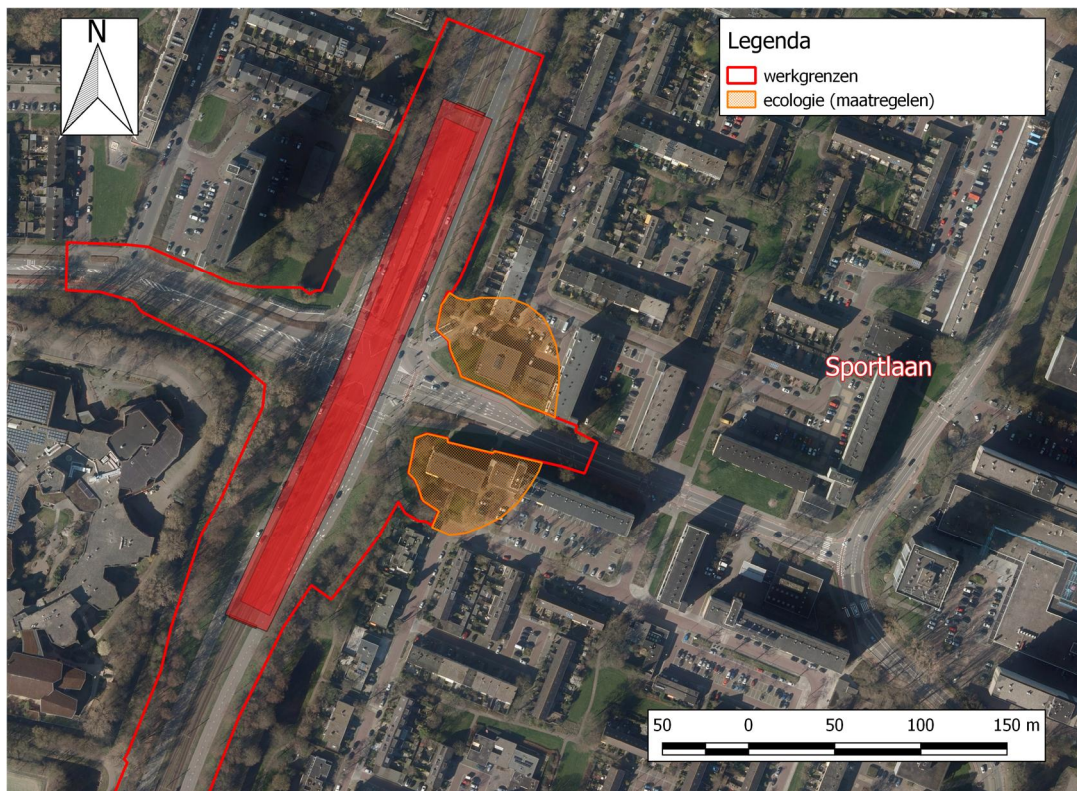
Figuur 16. In het oranje gearceerde gebied zijn maatregelen voor ecologie benodigd. De bomen die binnen de rode werkgrenzen vallen worden verwijderd.
