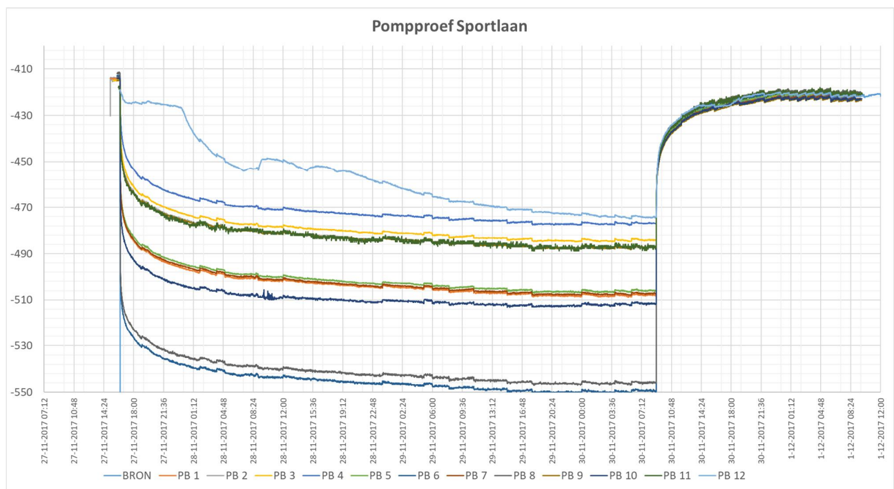
Figuur 60. Verlaging stijghoogte pompproef Sportlaan (stijghoogte in bron is NAP -7,5 m).
