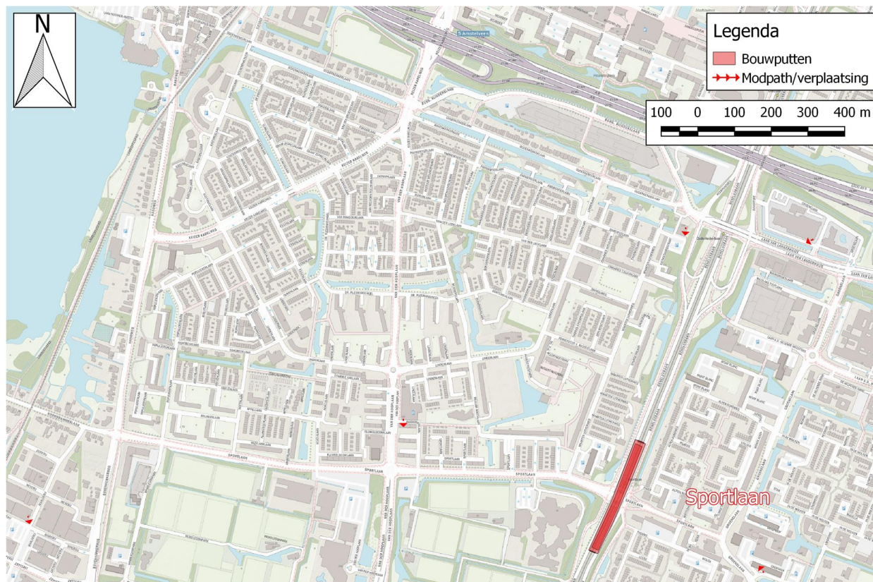
Figuur 53. Verplaatsing mogelijke verontreinigingen nabij Sportlaan. Verplaatsing is tussen 1,8 en 5,2 m. De freatische verlagingcontouren en de verlagingcontouren in de veenlaag reiken niet de locatie van de verontreinigingen. De verplaatsing is dus onder invloed van natuurlijke stroming.
