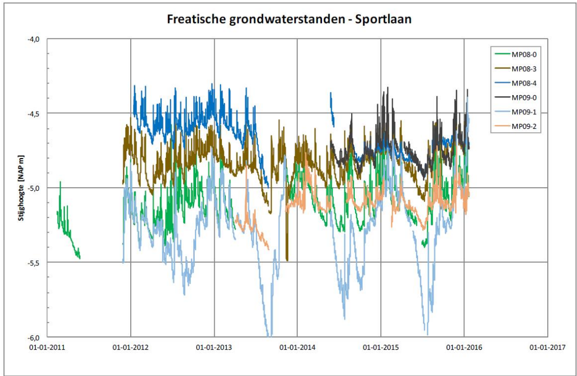
Figuur 77. Grondwaterreeks Sportlaan gemeente Amstelveen.
