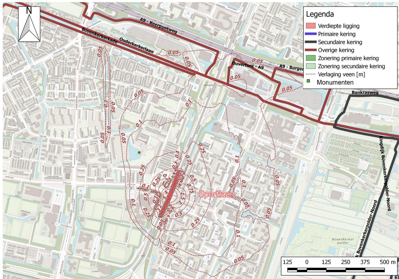
Figuur 46. Omgevingseffecten veenlaag, let op overige kering en aanwezigheid van monumentaal pand.
