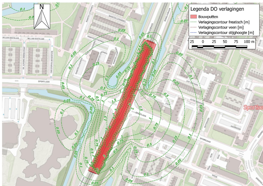
Sportlaan - verlaging freatische grondwaterstand in deklaag 1
