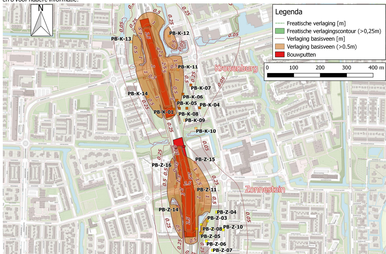
Figuur 44. Verlagscontouren (veen) en in bruin de arcering waarbinnen mogelijk grondwaterstand verder verlaagd wordt dan de signaalwaarde. Hiervoor zijn monitoringspeilbuizen gezet om dit nader te monitoren (oranje/geel=locatie monitoringspeilbuizen). Zie hoofdstuk 7.1.1 en 8 voor nadere informatie.
