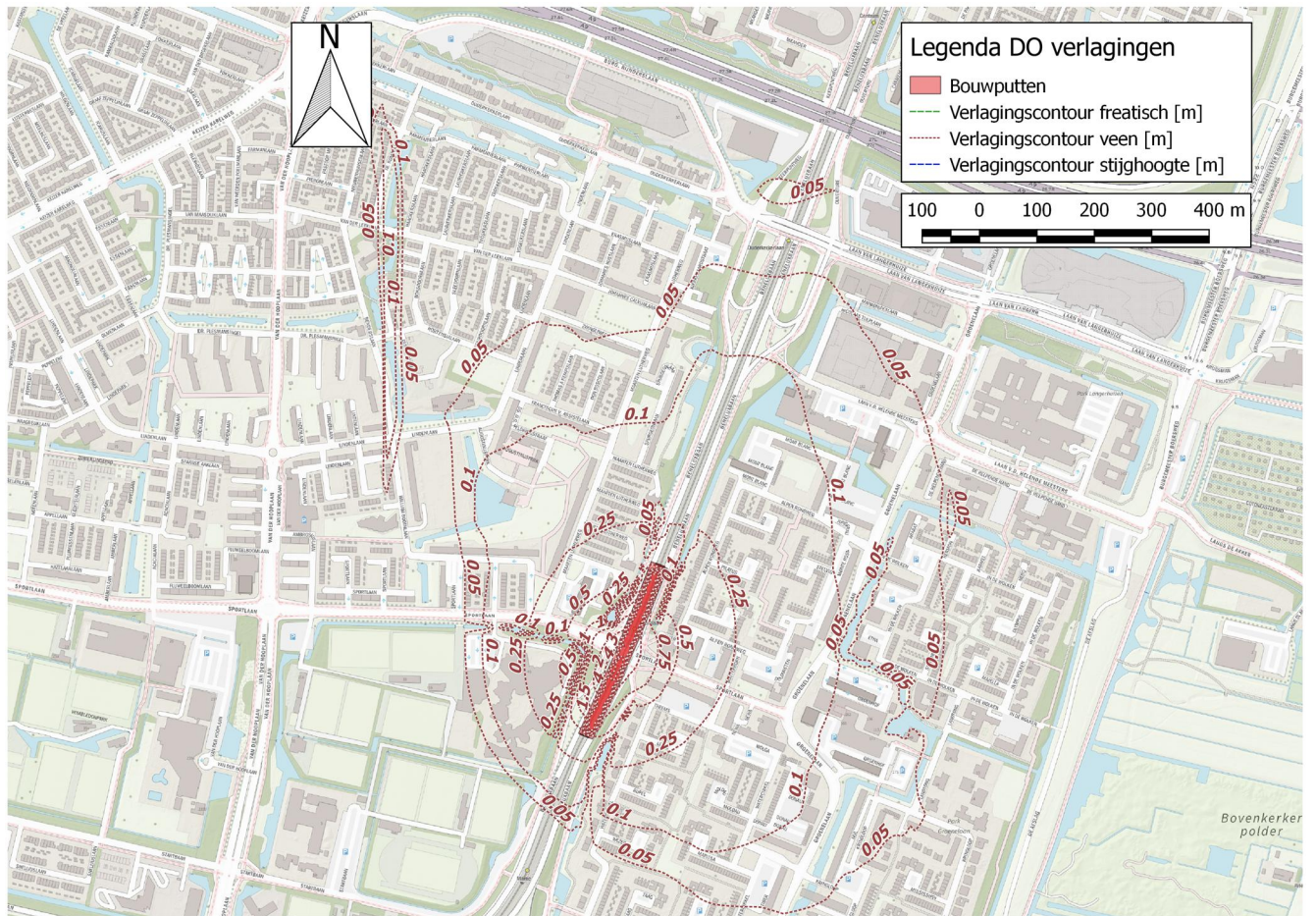
Figuur 29. Verlagsingscontouren in de veenlaag. De verlagsingscontouren beschrijven de verlaging zonder bemaling t.b.v. de waterkelder.
