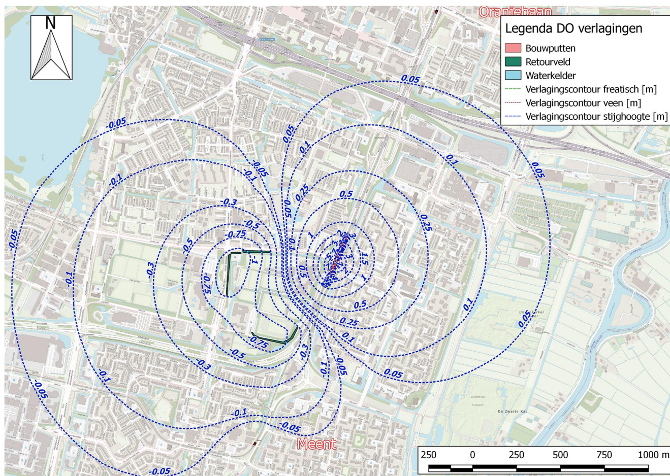
Figuur 33. Verlagsingscontouren Sportlaan in de pleistocene zanden onder de veenlaag. Inclusief bemaling waterkelder. Positief(+) = verlaging o.i.v. bemaling, negatief (-) = verhoging o.i.v. retourbemaling.
