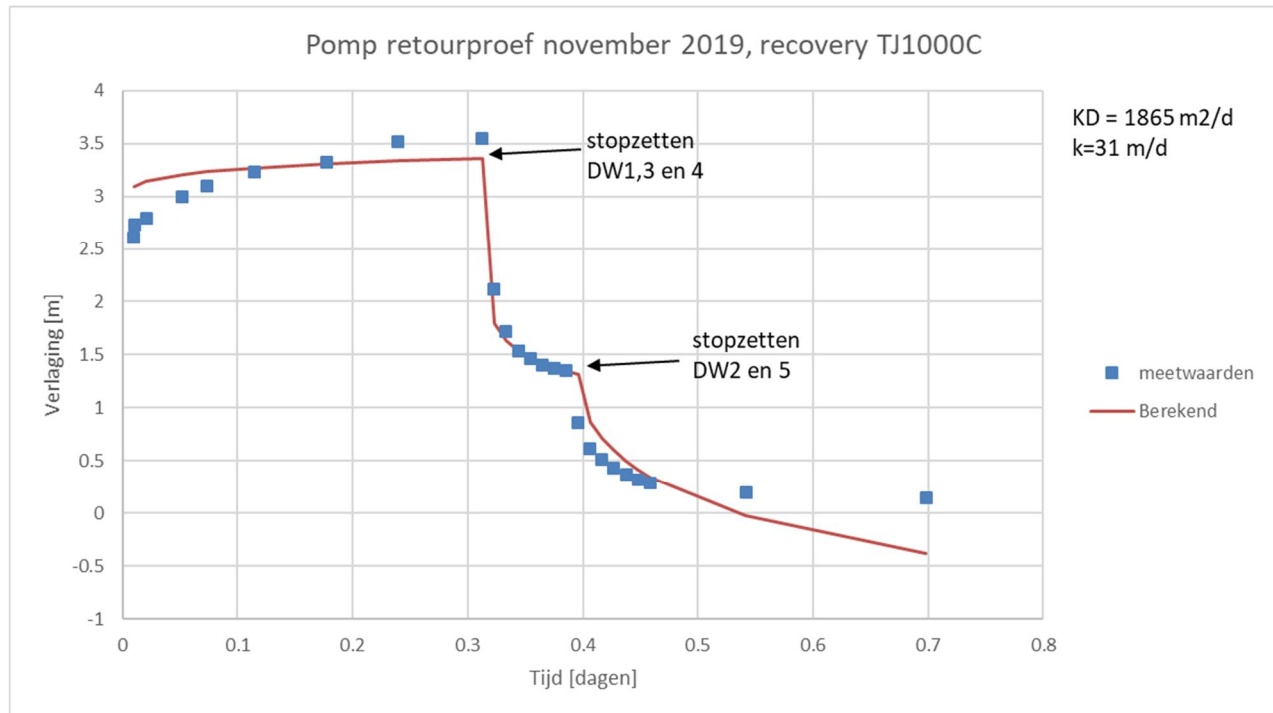
Figuur 65 Recovery in twee stappen peilbuis TJ1000C
