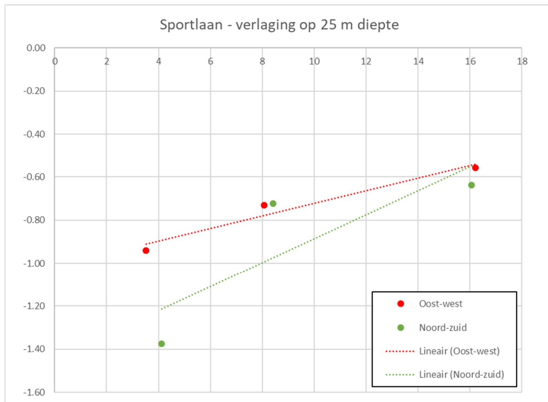
Figuur 62. Waarneming anisotropie op 25 m-mv nabij Sportlaan.
