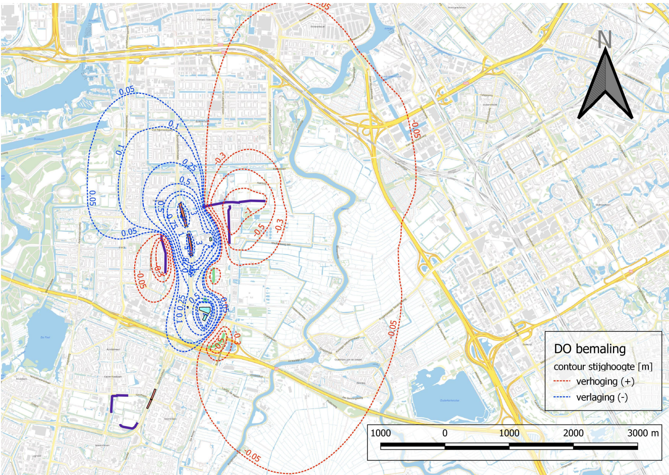
Figuur 24. Verlagscontouren 1e WVP (stijghoogte).
