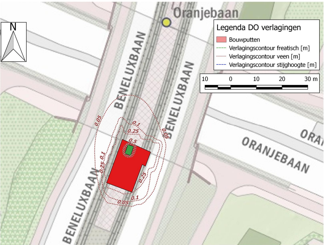
Figuur 23. Verlagsingscontouren veenlaag halte Oranjebaan.
