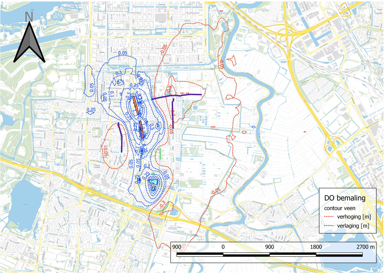
Figuur 22. Verlagsingscontouren veenlaag.
