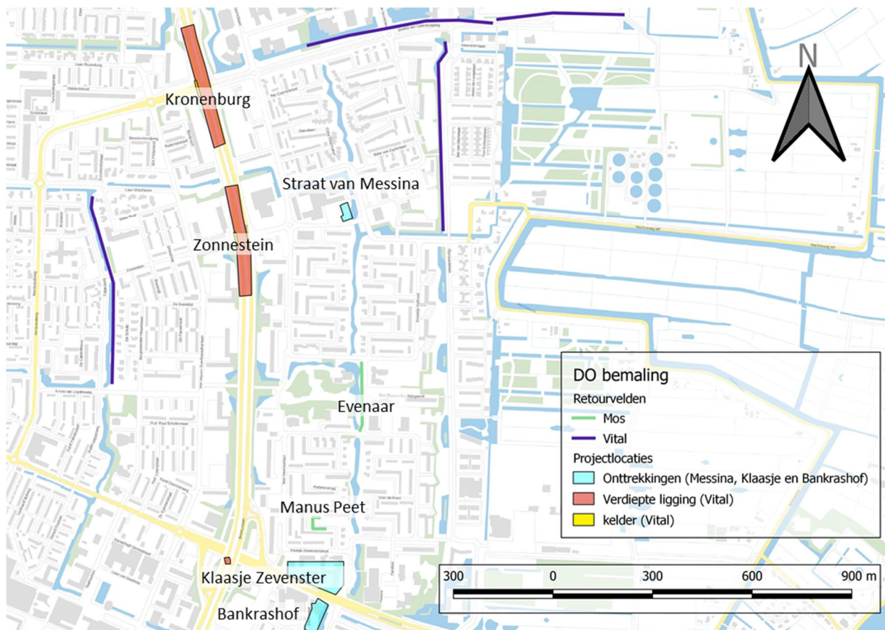
Figuur 9 Bemaling Vital en naburige bemalingen
