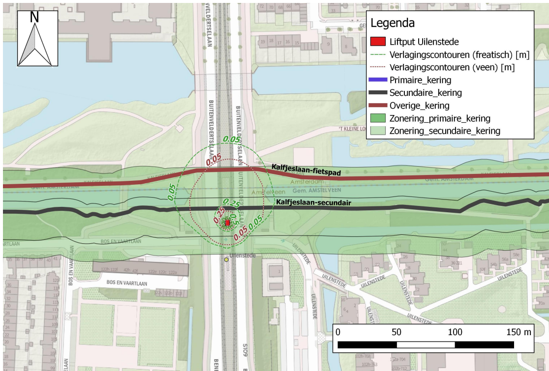
Figuur 39. Verlagingcontouren binnen secundaire en overige kering nabij Uilenstede.
