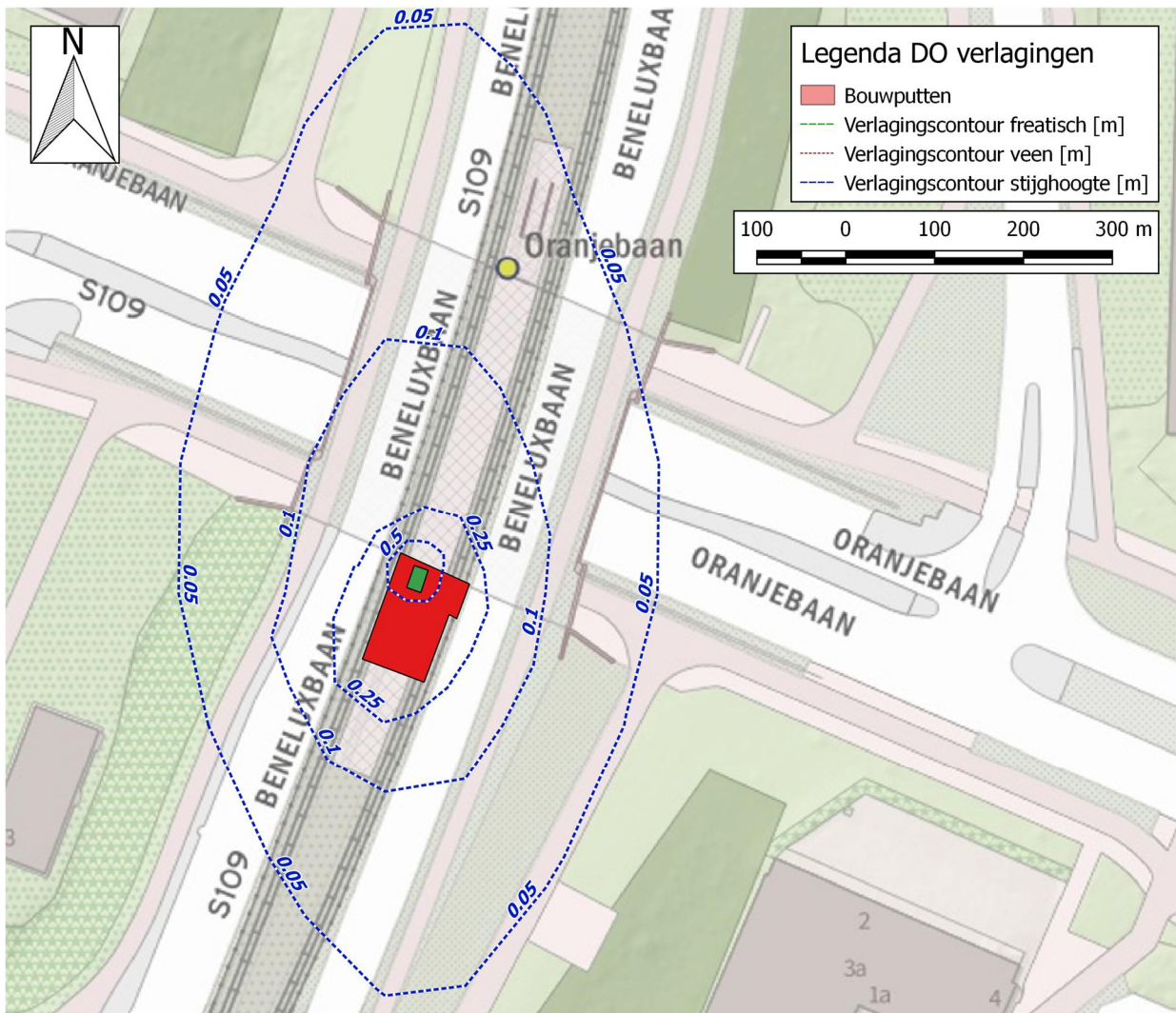
Figuur 25. Verlagingscontouren 1e WVP (stijghoogte) halte Oranjebaan.
