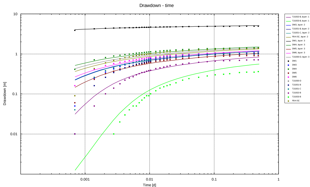
Figuur 67 Tijd versus verlaging DW1 (117 m 3 /h) met MLU fit
