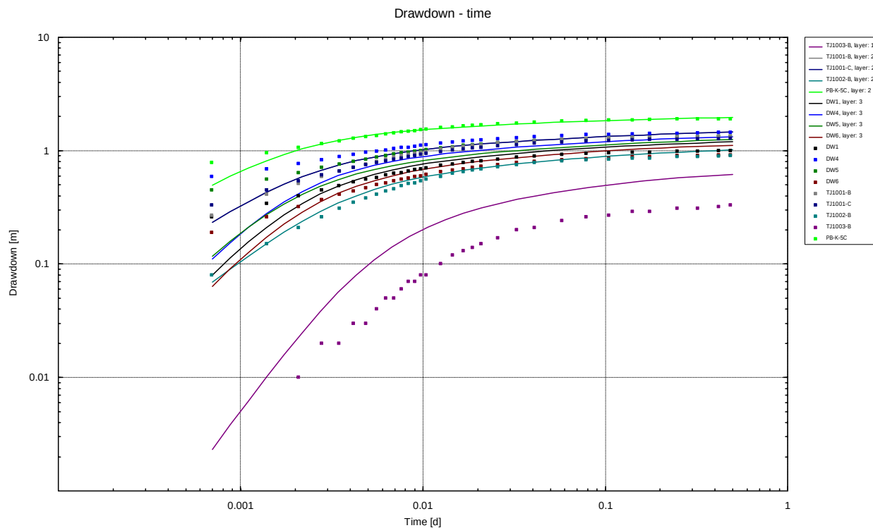
Figuur 68 Tijd versus verlaging DW3 (104 m 3 /h) met MLU fit
