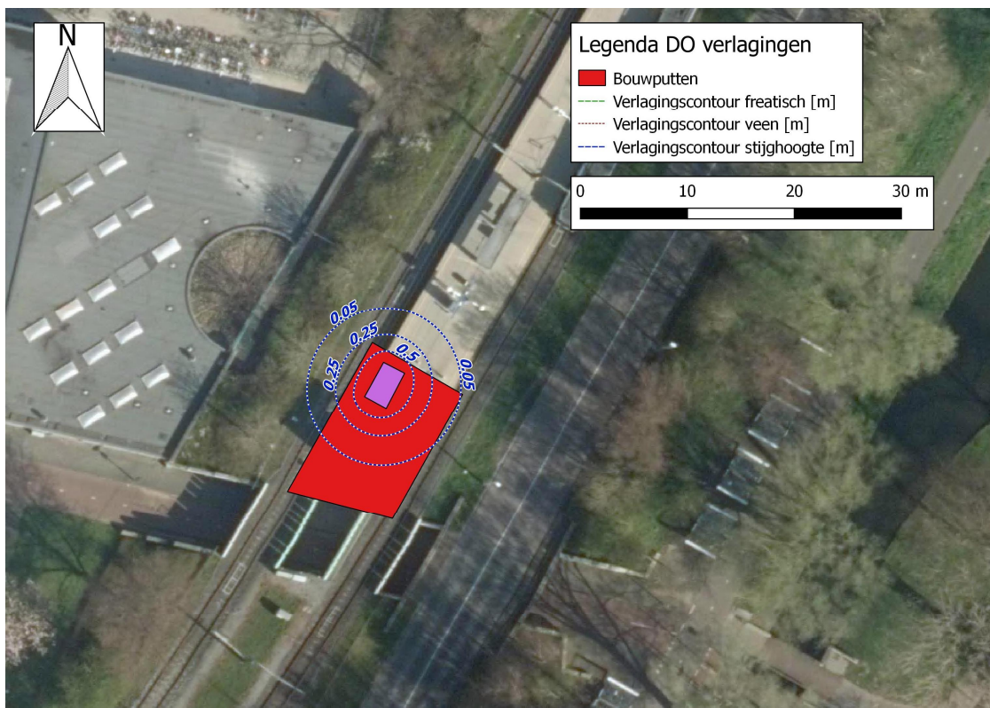
Figuur 36. Verlagscontour (stijghoogte, 1e WVP) halte Meent. In rood: bouwput en in paars: liftput.
