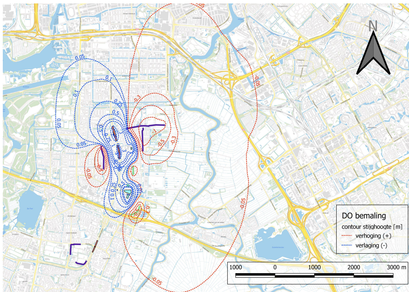
Figuur 12. Verlagingen (+) en verhoging (-) contouren in het 1 e watervoerende pakket.
