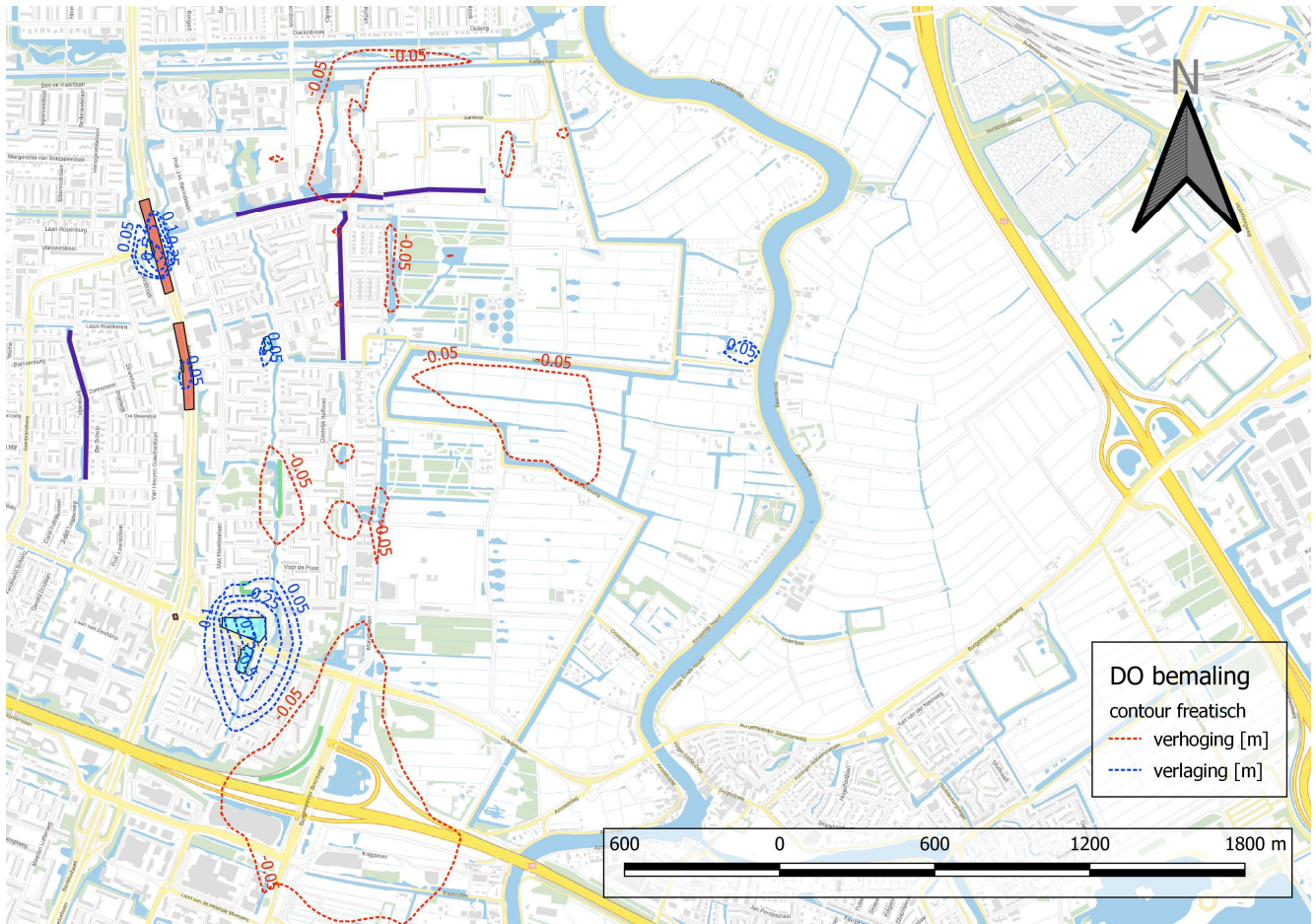
Figuur 18. Freatische verlagingcontouren [m] na 28 dagen bemalen voor de waterkelders.
