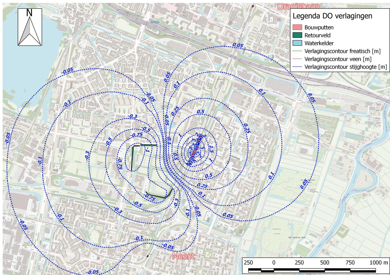
Figuur 48. Verlaging (+) door bemalingswerkzaamheden en verhoging (-) door retourveld van de stijghoogte in 1e WVP na 112 dagen bemalen.
