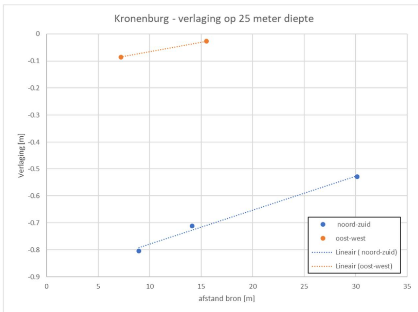
Figuur 58. Waarneming anisotropie op 25 m-mv nabij Kronenburg.
