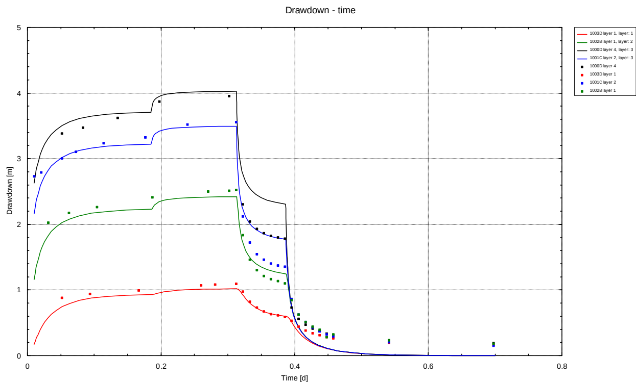
Figuur 69 Tijd versus verlaging DW1,2,3,4 en 5 (426 m 3 /h) met MLU fit
