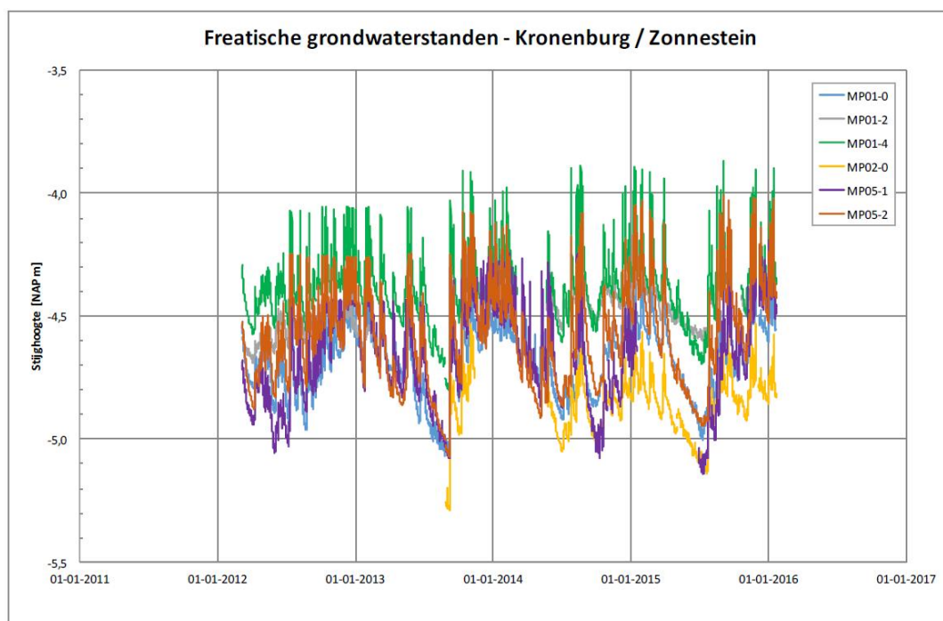
Figuur 75. Grondwaterreeks Kronenburg/Zonnestein gemeente Amstelveen.
