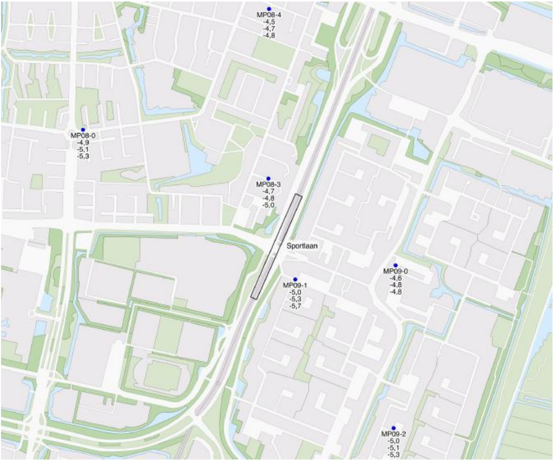
Figuur 76. Locatie peilbuizen gemeente Amstelveen.
