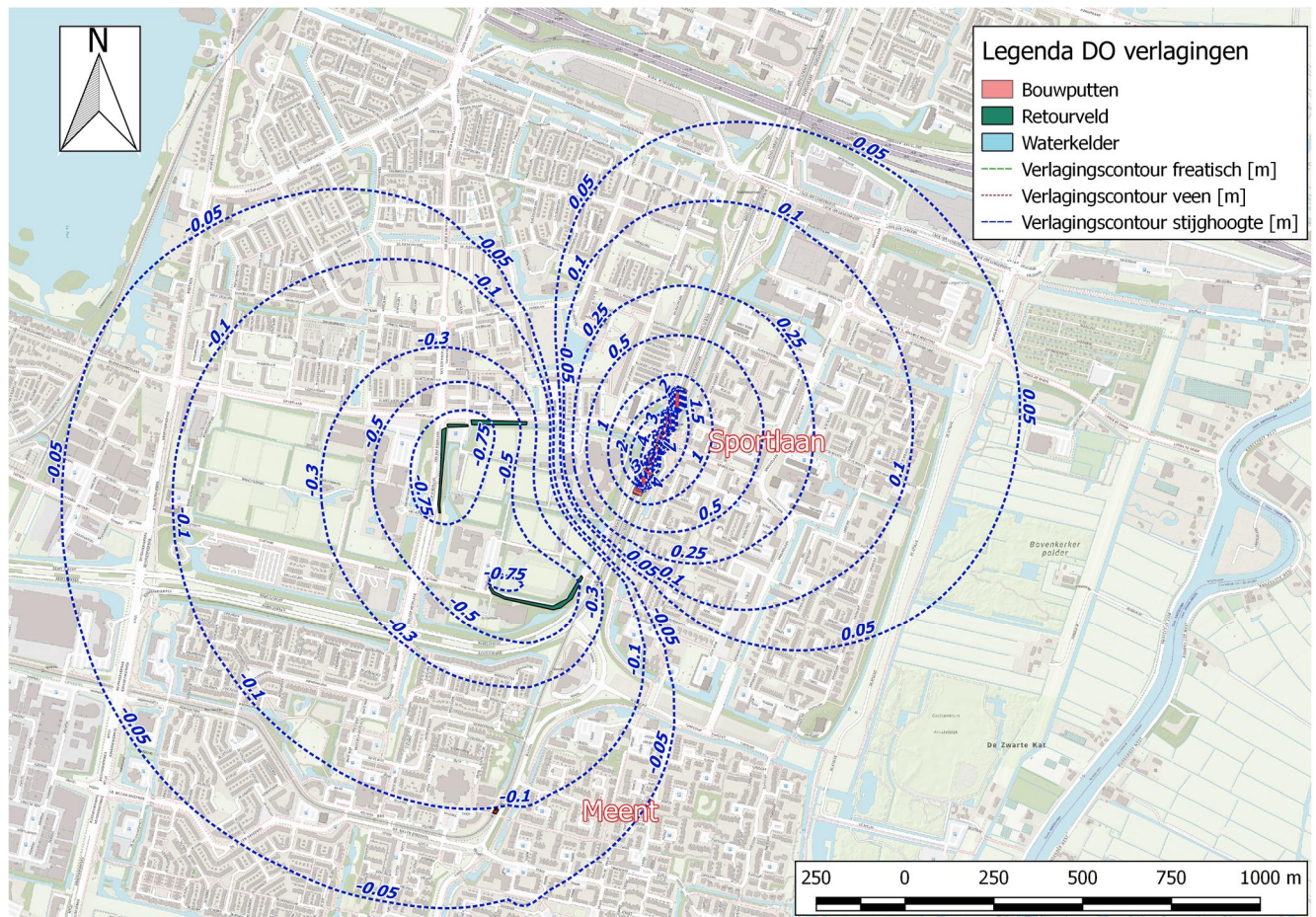
Figuur 30. Verlagingscontouren in het 1e WVP. De verlagingcontouren geven de situatie weer zonder bemaling van de waterkelder.
