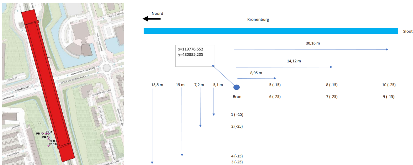
Figuur 55. Overzicht pompproef Kronenburg. Links: in roze de locatie van de peilbuizen, rechts: diepte [m-mv] en afstand van peilbuizen.
