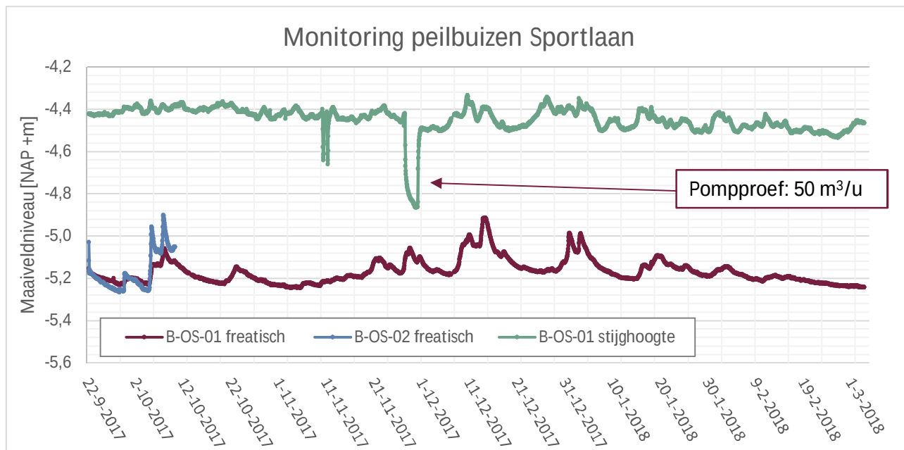
Figuur 72. Fluctuatie grondwaterstanden Sportlaan september 2017 – maart 2018.
