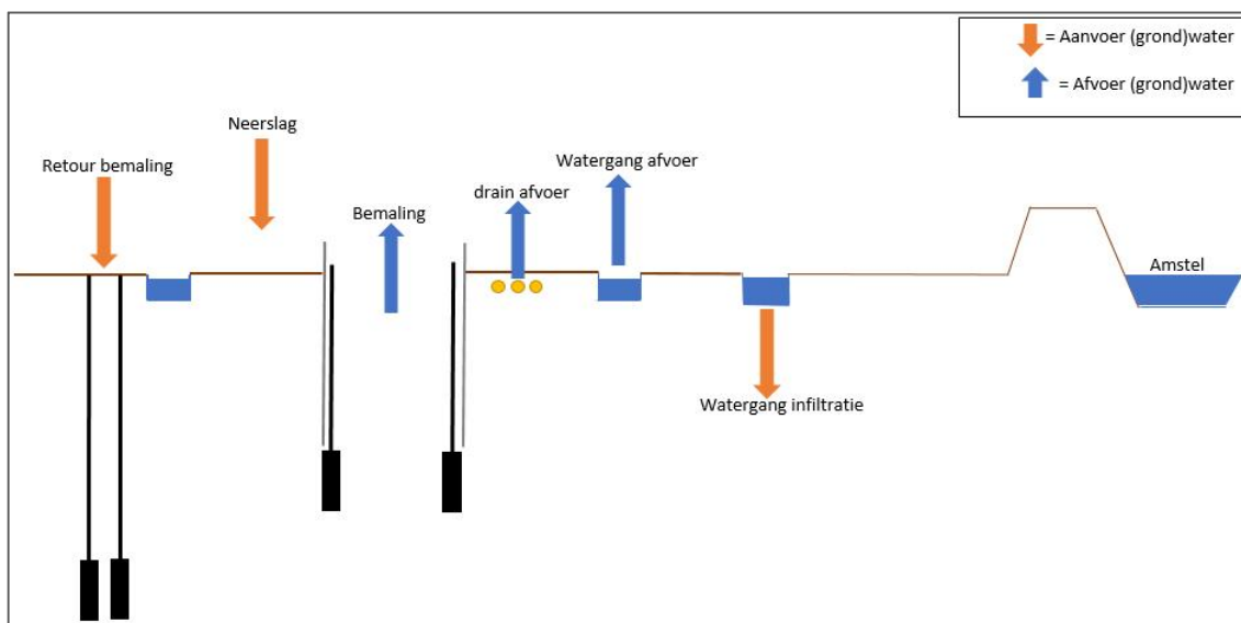
Figuur 17. Schets waterbalans
