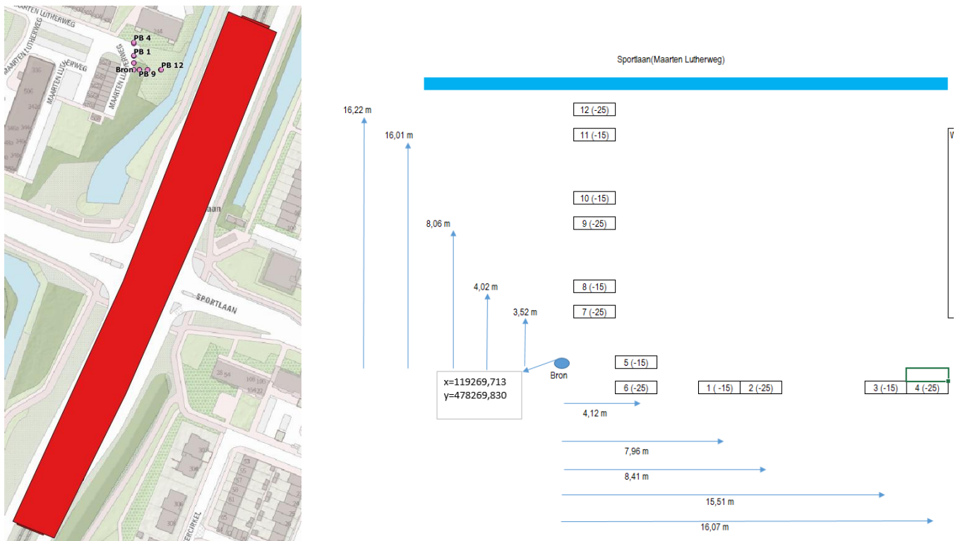
Figuur 59. Overzicht pompproef Sportlaan. Links: in roze de locatie van de peilbuizen, rechts: diepte [m-mv] en afstand van peilbuizen.
