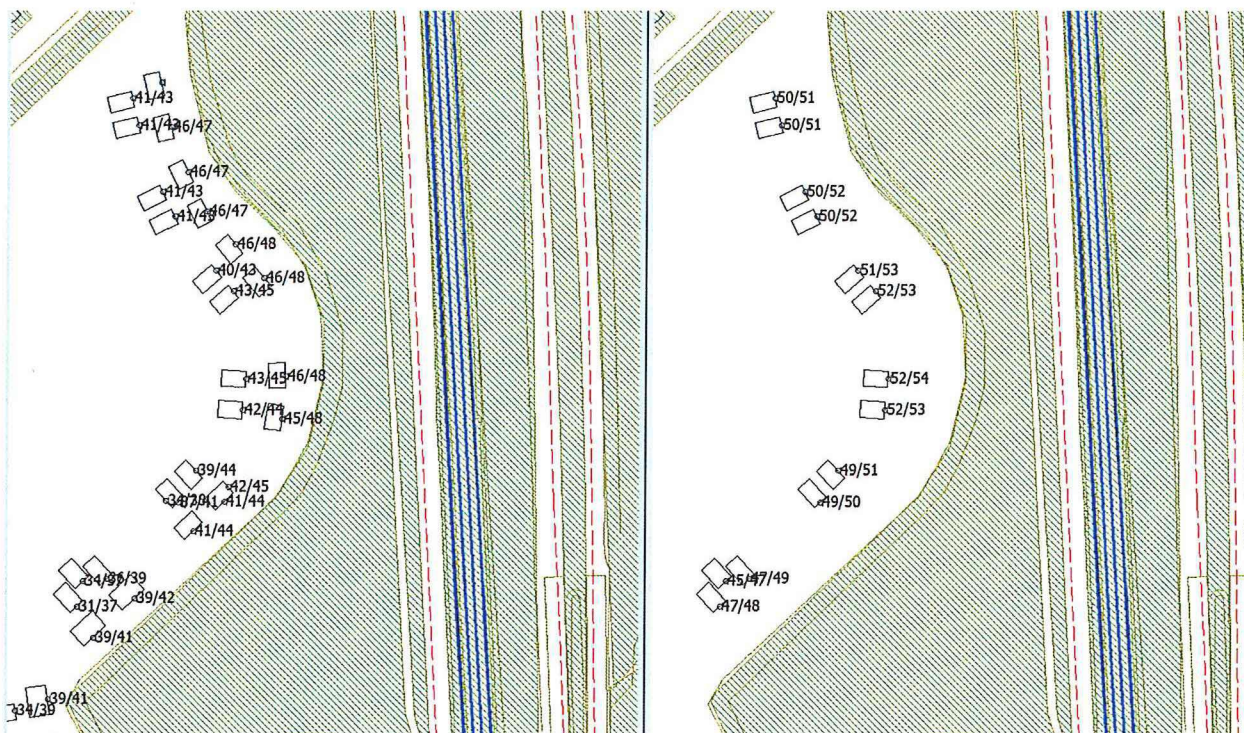
Geluidsbelasting Prins Mauritssingel drijvende woningen in de Oosterhoutseplas
