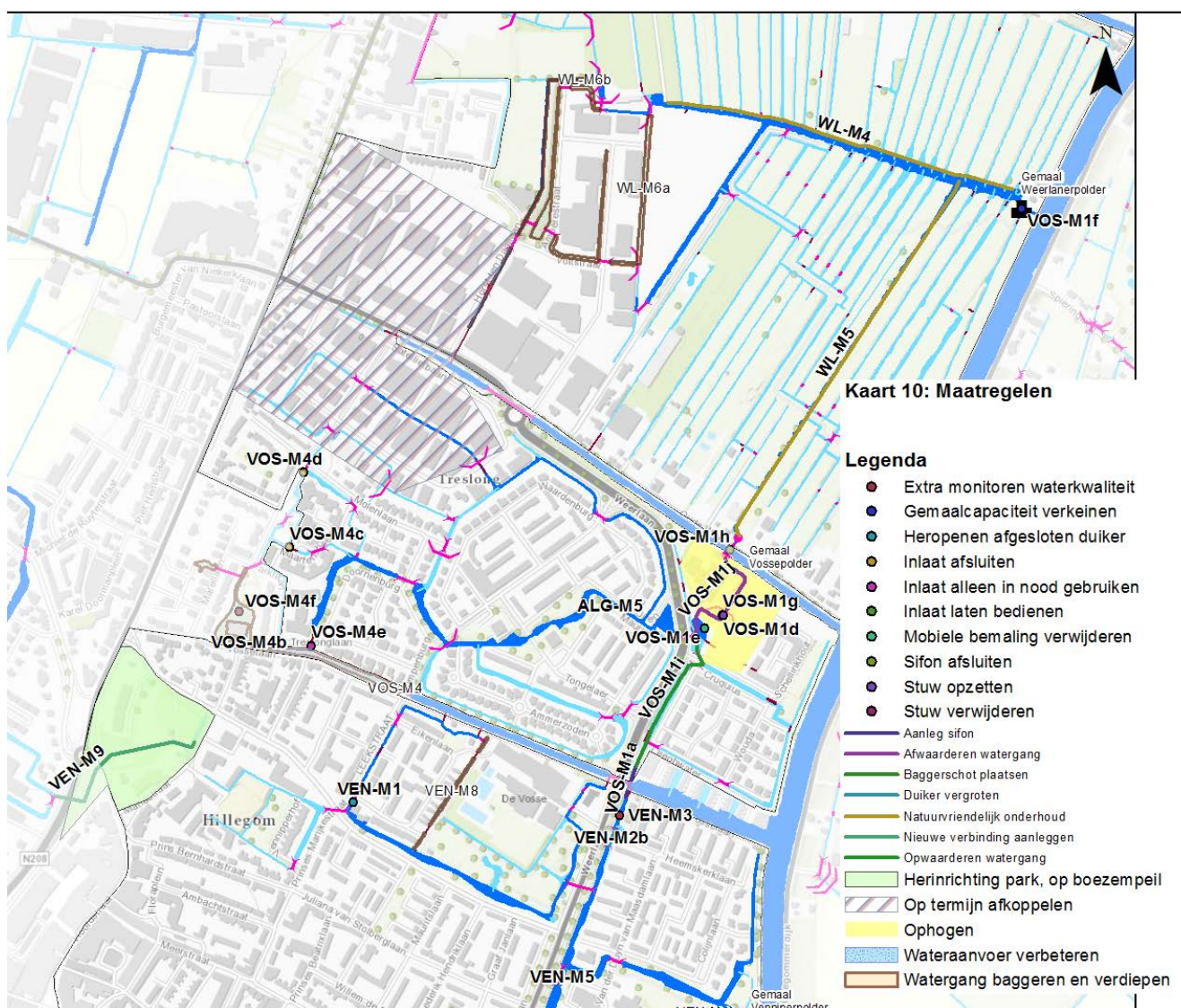
Figuur 5-1 Overzichtsk kaart van de voorgestelde maatregelen
