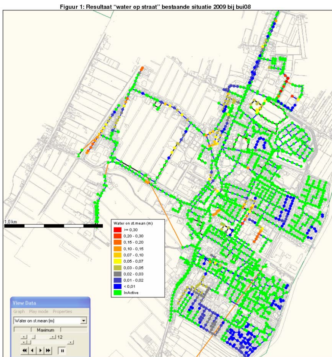
Figuur 5-4 Kaartbeeld van de toetsing op water-op-straat, Bui 8, situatie in 2009
