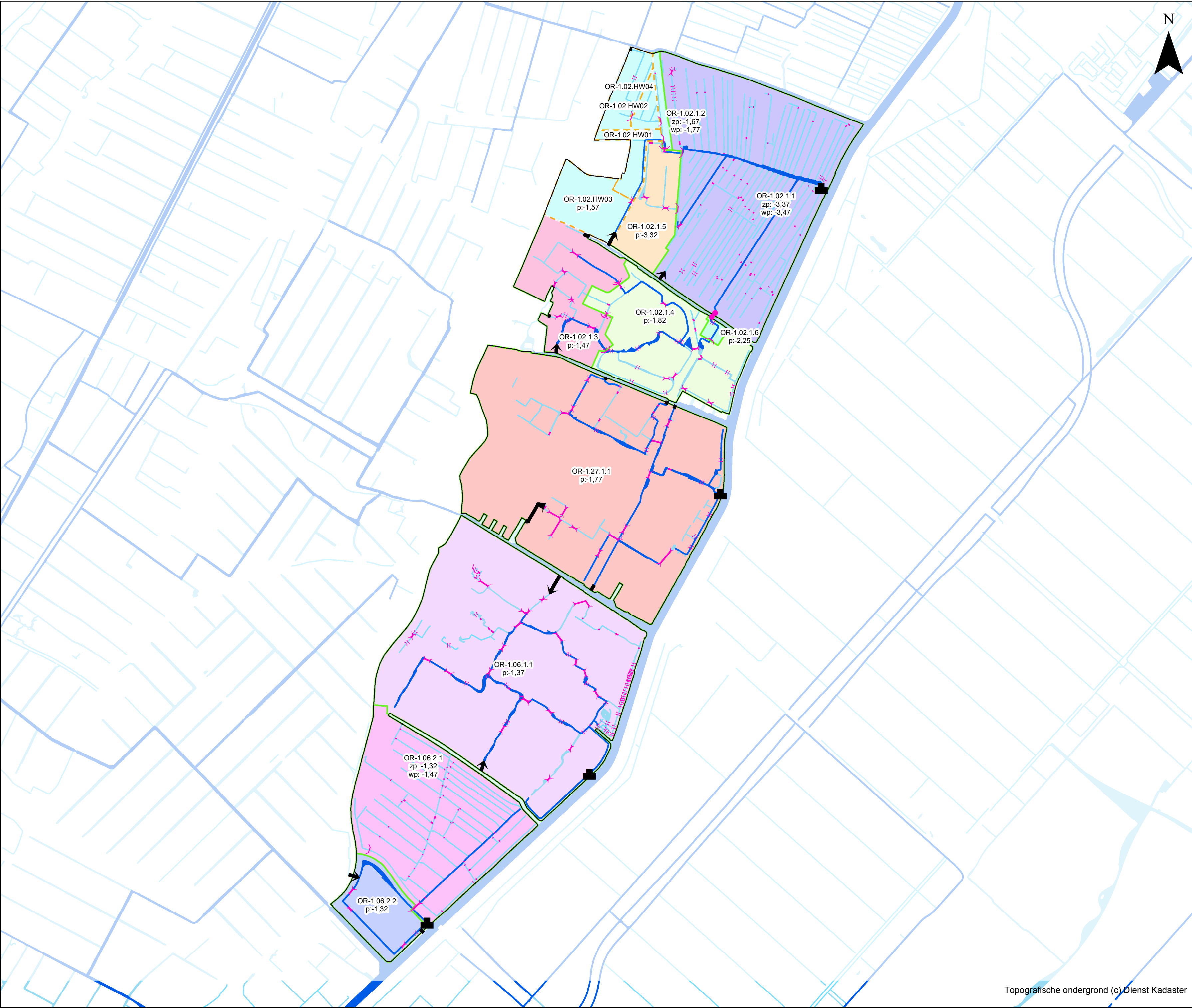
Kaart 6: Huidige waterhuishoudkundige situatie (o.b.v. praktijkpeilen)
