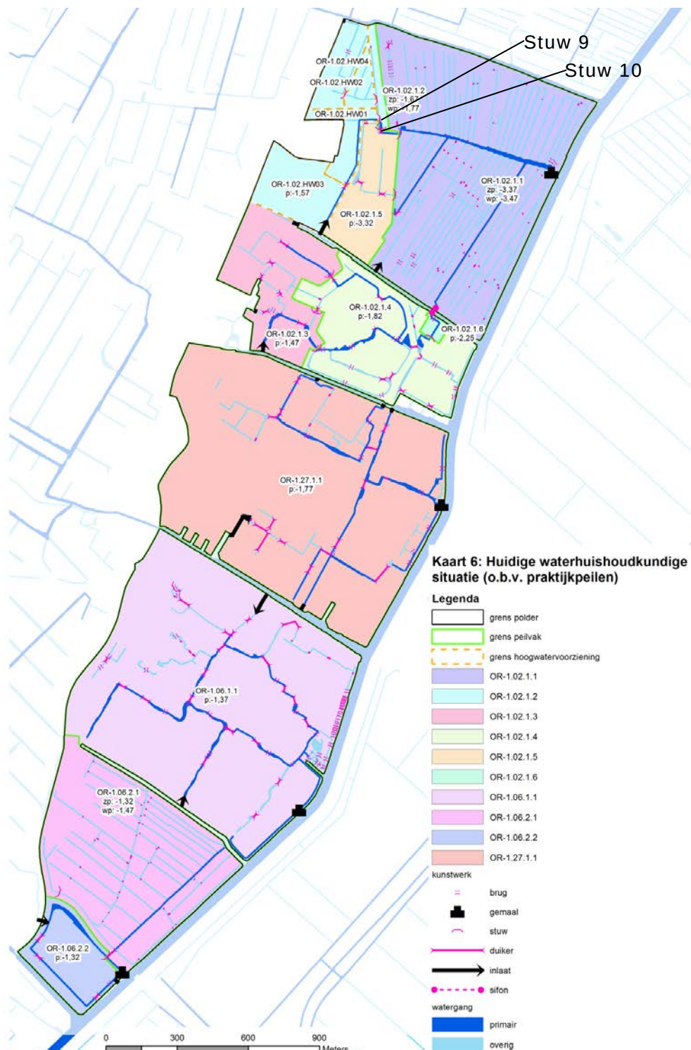
Figuur 4-1 Watersysteem van de vier polders
