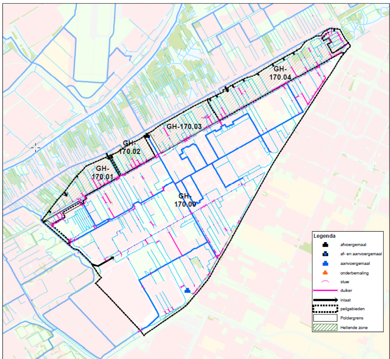
Figuur 5.1 Peilvoorstel
