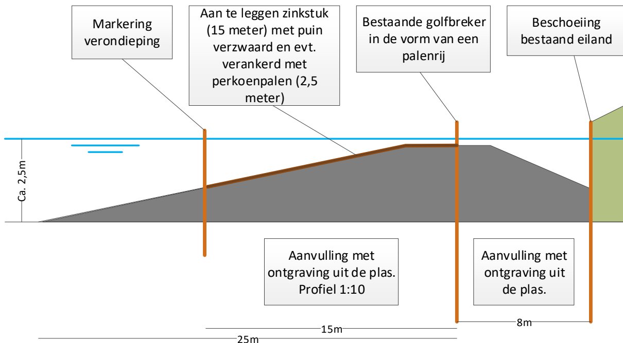
Figuur 2.3.: Dwarsdoorsnede aanleg onderwatertalud (grijs: aanvulling vaste bodem uit ontgravingslocatie).
