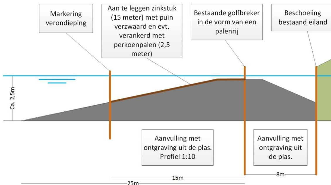
Dwarsdoorsnede aanvulling talud rieteiland
