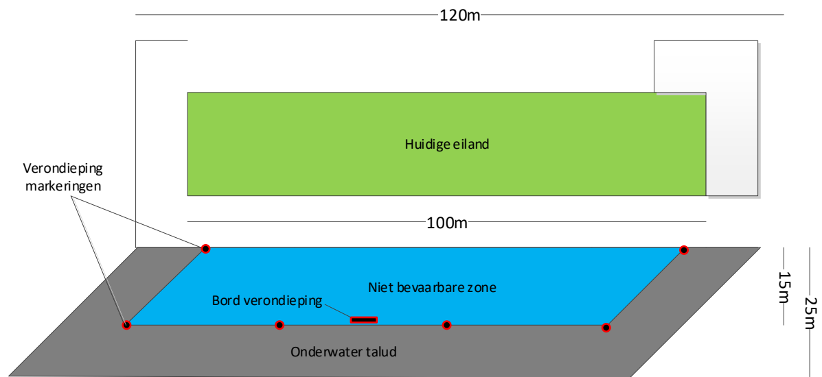
Figuur 2.4.: Bovenaanzicht verondieping met markering..
