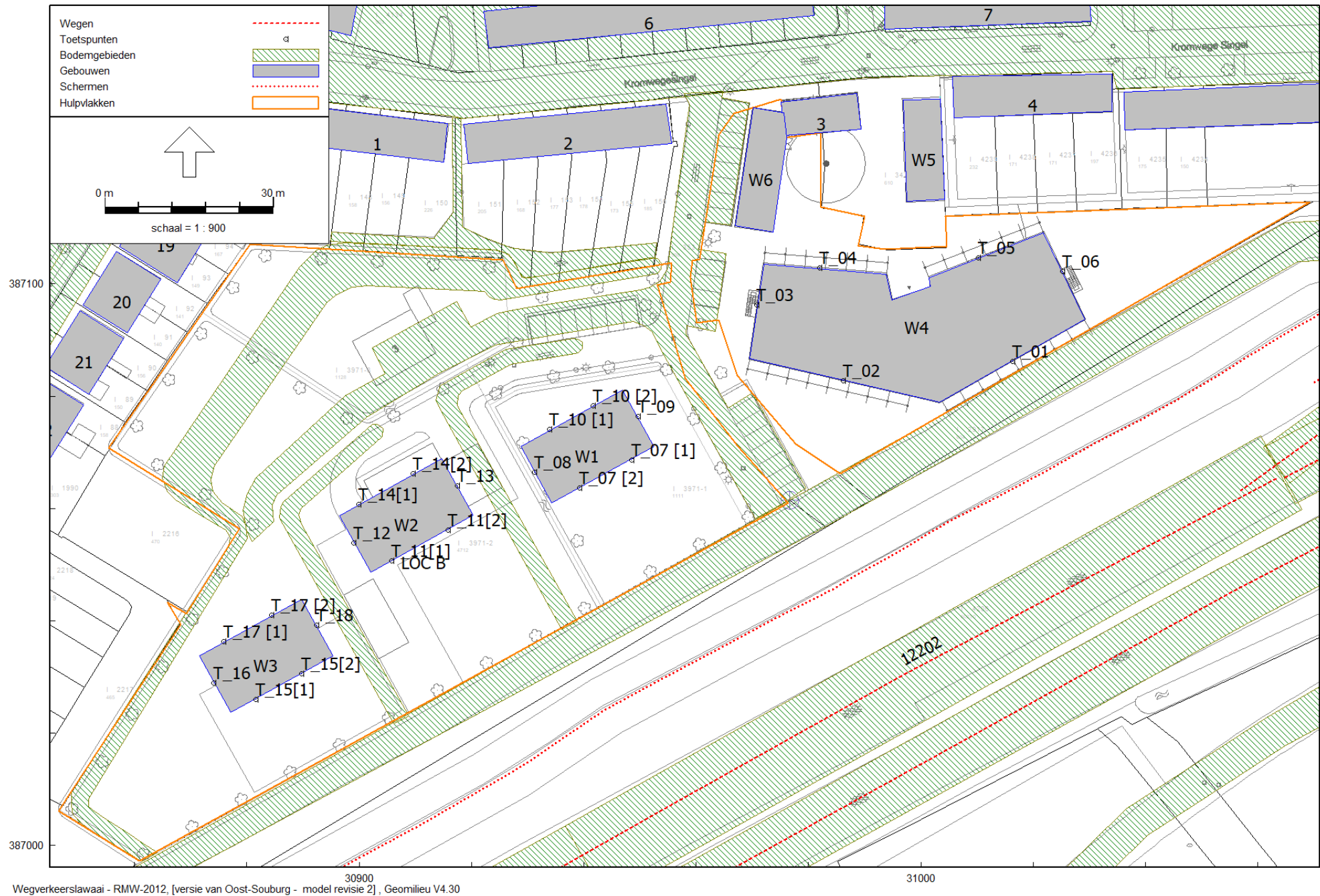
Figuur 2 Detailweergave model met ligging toetspunten
