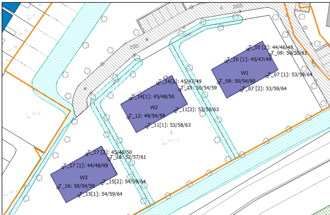
Figuur 5.1: Rekenresultaten vanwege de A58, met 2 dB aftrek.
