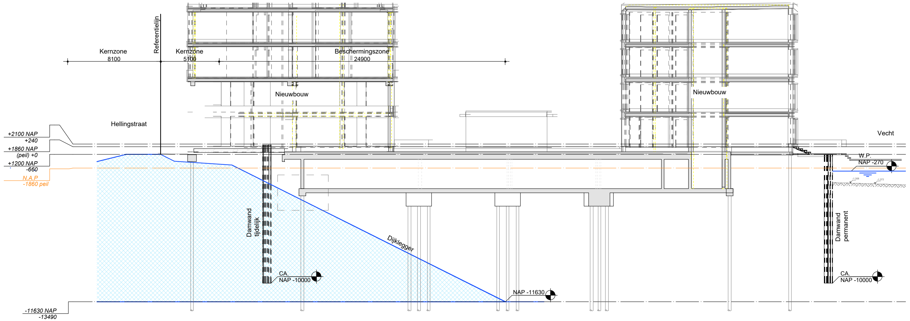
DOORSNEDE 5 1:200
