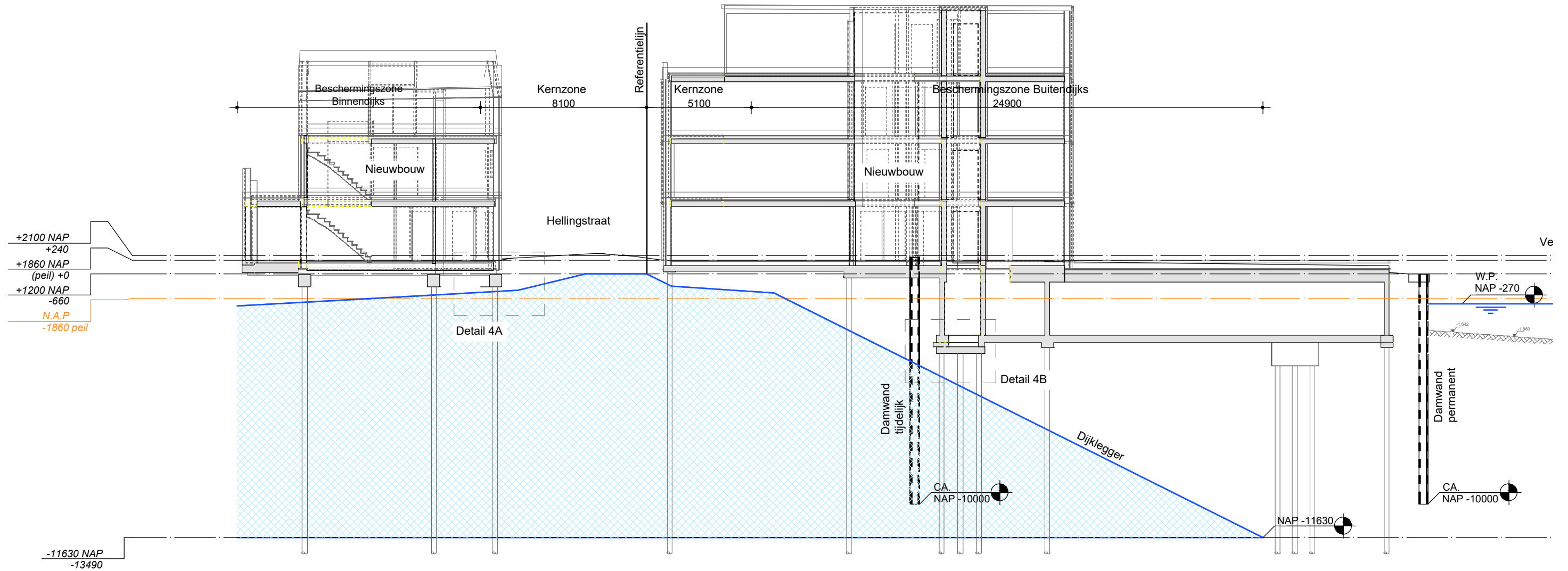
DOORSNEDE 4 1:200
