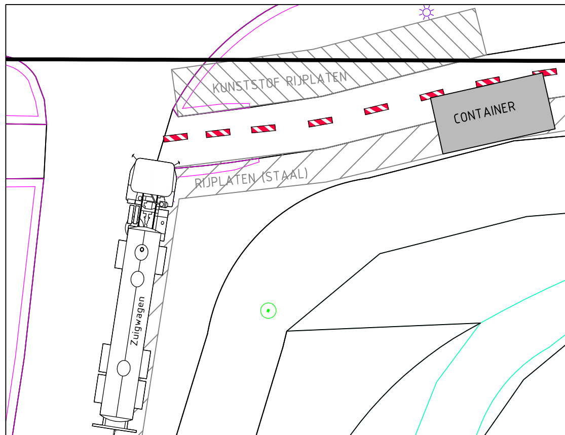
OPSTELLING UITREDEPUNT SCHAAL 1:200
