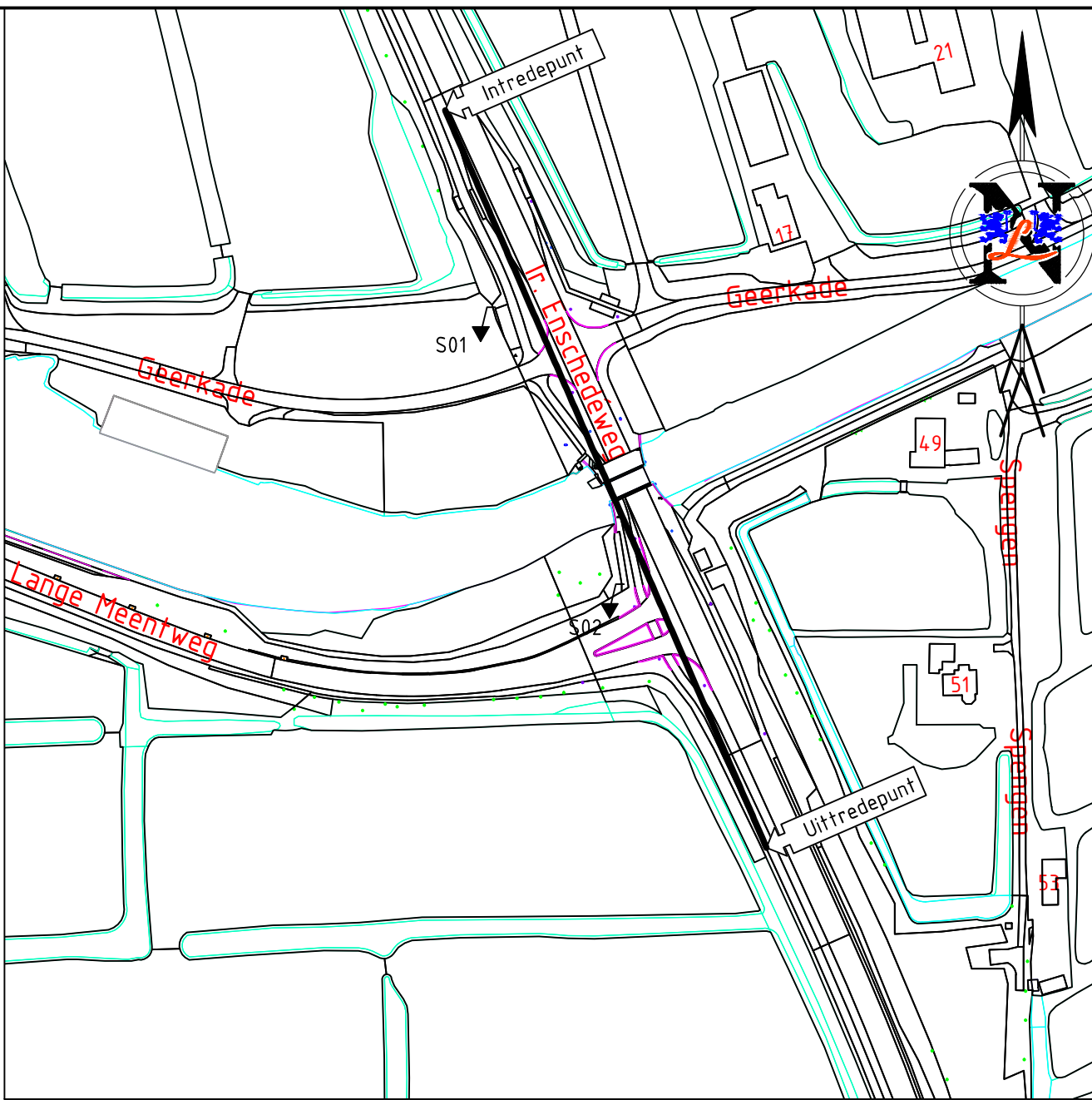
SITUATIE SCHAAL 1:2000
