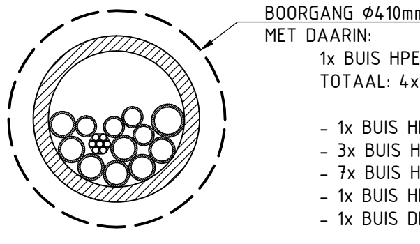
DOORSNEDEN BORING SCHAAL 1:10
