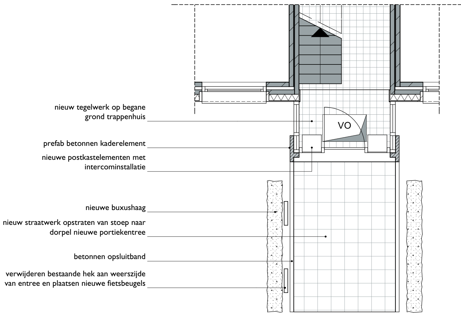
BEGANE GROND
