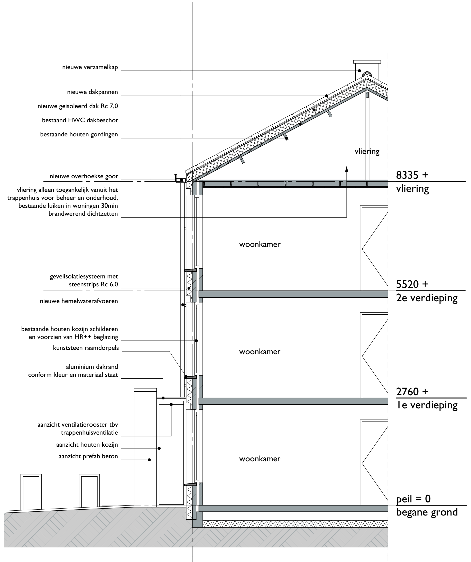
DOORSNEDE A-A
