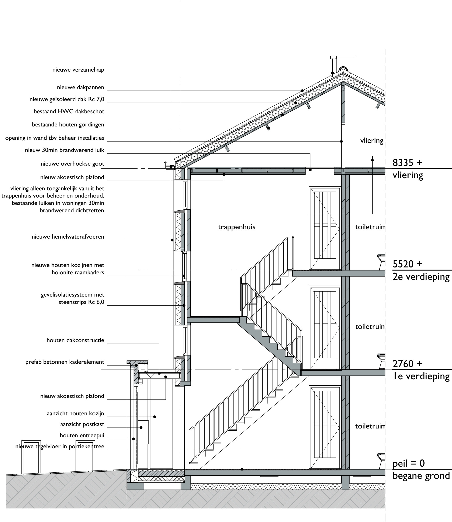
DOORSNEDE B-B
