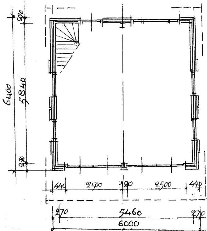
Begane grond
