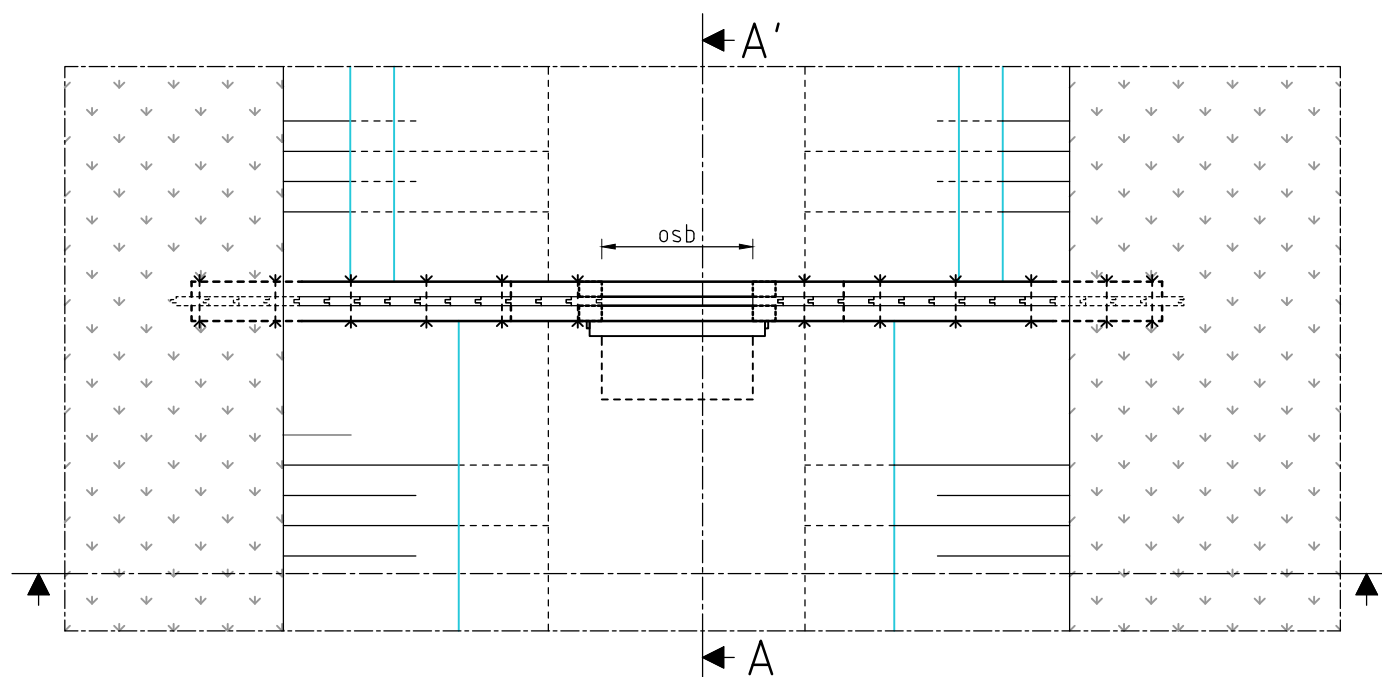
Bovenaanzicht
