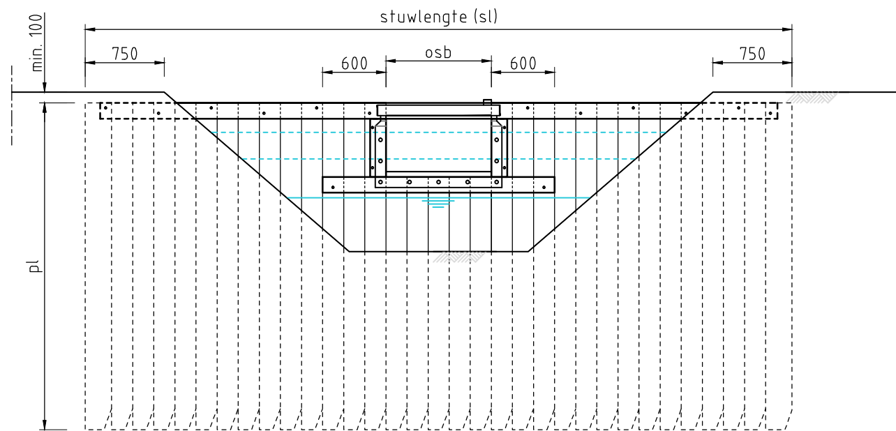
Vooraanzicht
