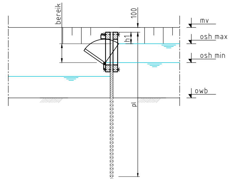
Doorsnede A-A'
