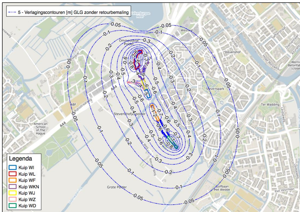
Figuur 11: Verlagingscontouren [m] deklaag a.g.v. spanningsbemaling, zonder retourbemaling, onder GLG-condities.
