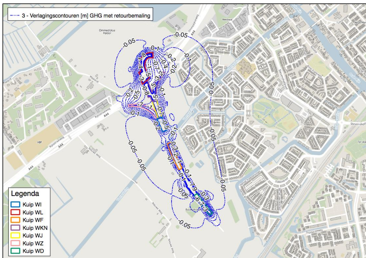
Figuur 19: Verlagingscontouren [m] deklaag a.g.v. spanningsbemaling, met retourbemaling op de systeemgrenzen, onder GHG-condities.
