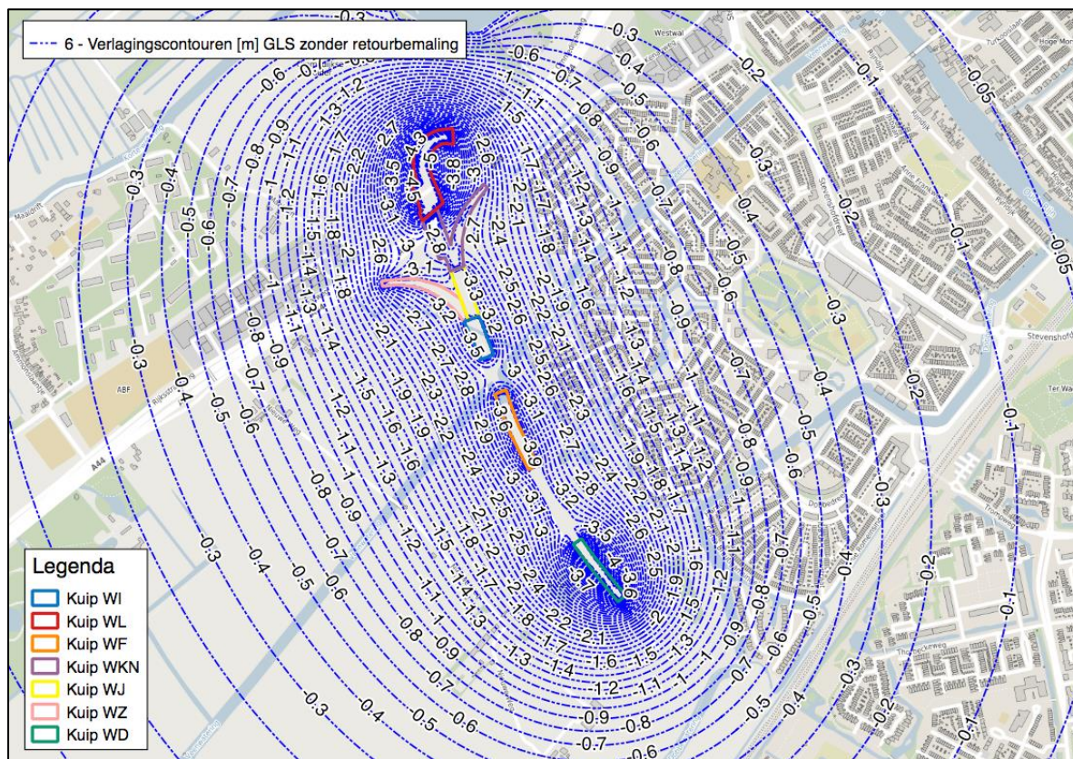
Figuur 13: (ingezoomd t.o.v. vorig figuur) Verlagingscontouren [m] eerste watervoerend pakket a.g.v. spanningsbemaling, zonder retourbemaling, onder GLS-condities.
