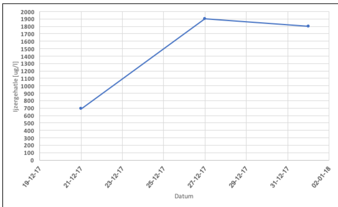
Figuur 8: Verloop ijzergehalte [ \mu\text{g/l} ] in lozingswater gedurende de proef.
