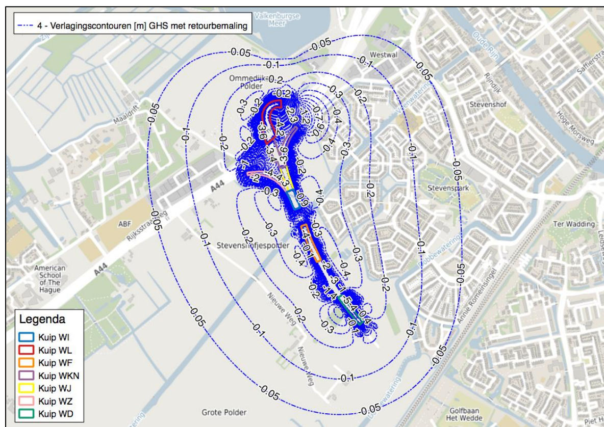
Figuur 20: Verlagingscontouren [m] eerste watervoerend pakket a.g.v. spanningsbemaling, met retourbemaling op de systeemgrenzen, onder GHS-condities.
