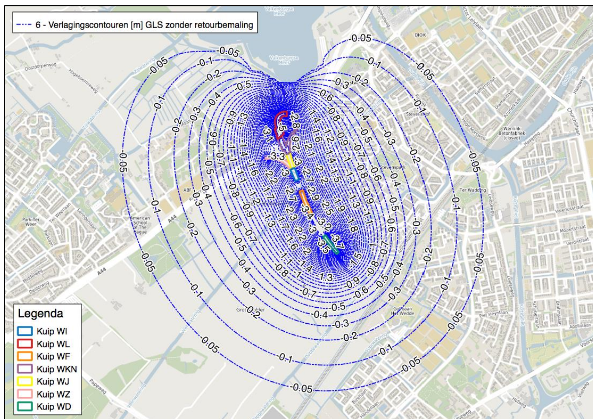
Figuur 12: Verlagingscontouren [m] eerste watervoerend pakket a.g.v. spanningsbemaling, zonder retourbemaling, onder GLS-condities.
