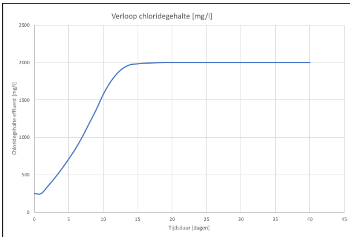
Figuur 25: Worst-case verloop chloridegehalte in het effluent a.g.v. onttrekken van dieper chloridehoudend grondwater.
