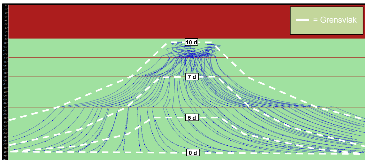
Figuur 24: Upconing zoet-zoutgrensvlak berekend met MicroFEM. Stroming opwaarts. NB. De afstand tussen twee punten op de betreffende flowline staat voor een afgelegde afstand richting de onttrekking in 1 dag. Na ca. 10 dagen bereikt het zoute grondwater de onttrekking, waar het vermengd wordt met het ondiepere zoetwater.
