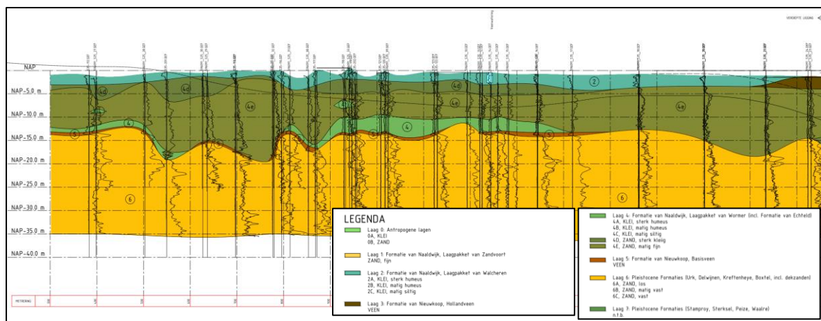
Figuur 6 – Lengteprofiel
