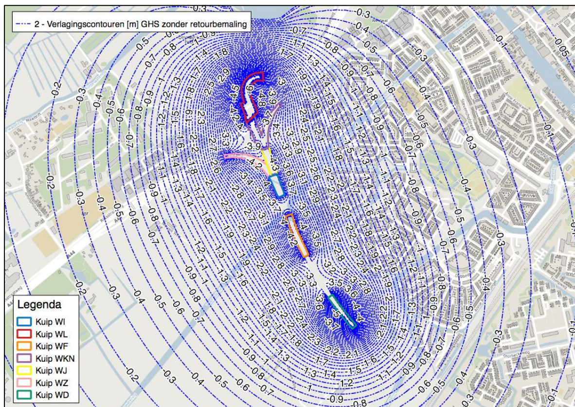
Figuur 16: (ingezoomd t.o.v. vorig figuur) Verlagingscontouren [m] eerste watervoerend pakket a.g.v. spanningsbemaling, zonder retourbemaling, onder GHS-condities.
