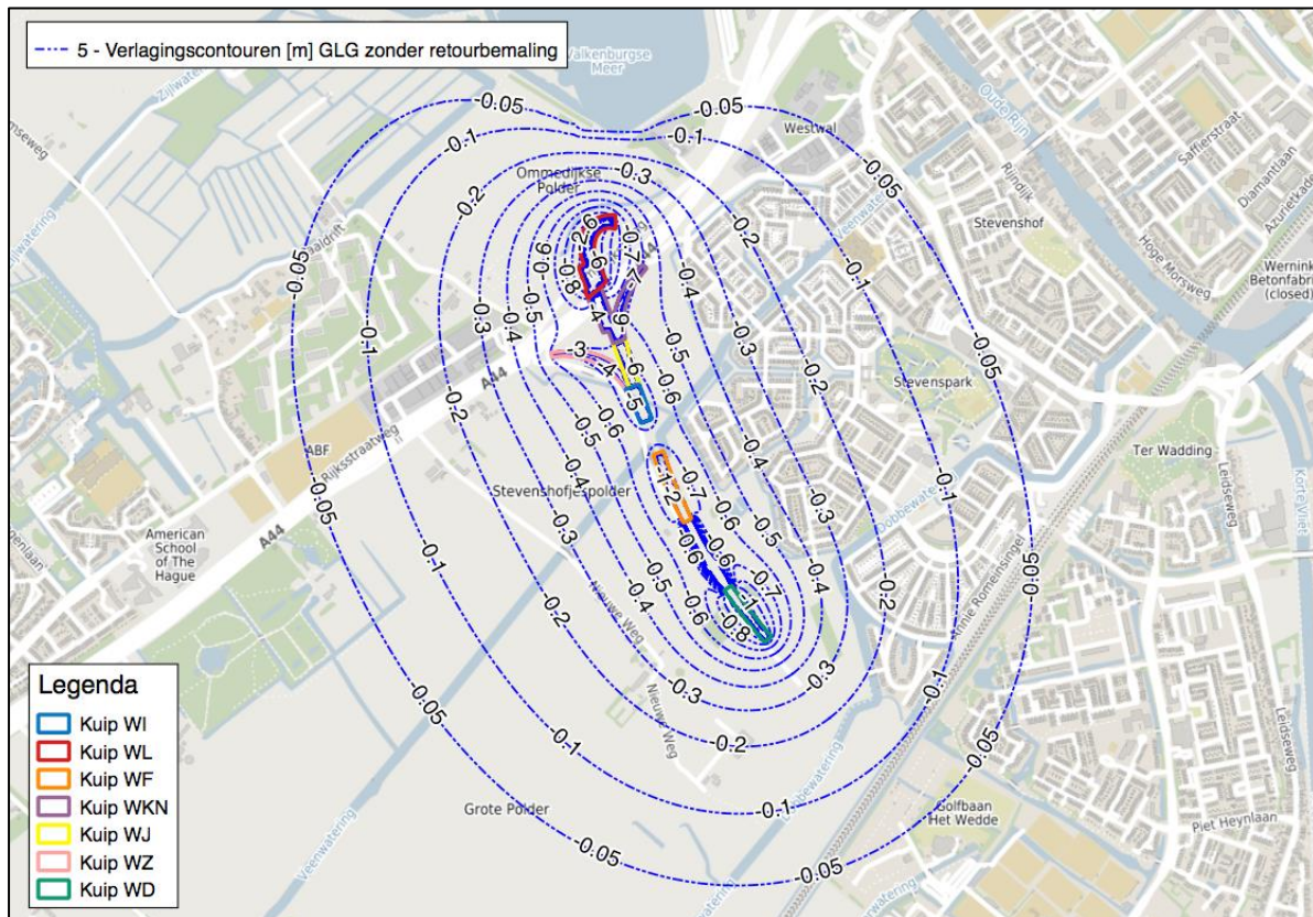
Figuur 6: Verlagingscontouren [m] deklaag a.g.v. spanningsbemaling, zonder retourbemaling, onder GLG-condities.
