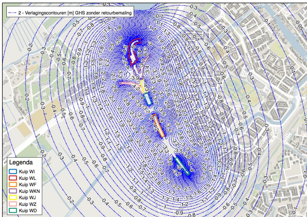
Figuur 11: (ingezoomd t.o.v. vorig figuur) Verlagingscontouren [m] eerste watervoerend pakket a.g.v. spanningsbemaling, zonder retourbemaling, onder GHS-condities.
