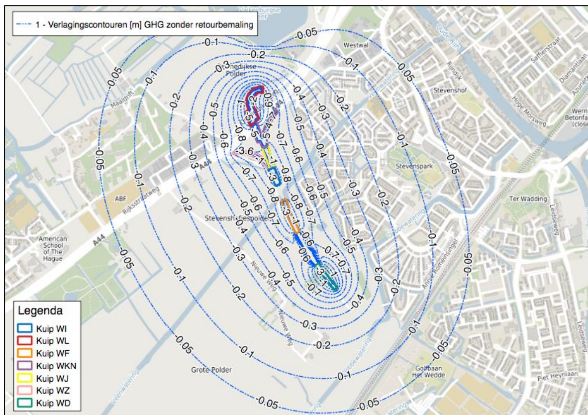
Figuur 9: Verlagingscontouren [m] deklaag a.g.v. spanningsbemaling, zonder retourbemaling, onder GHG-condities.
