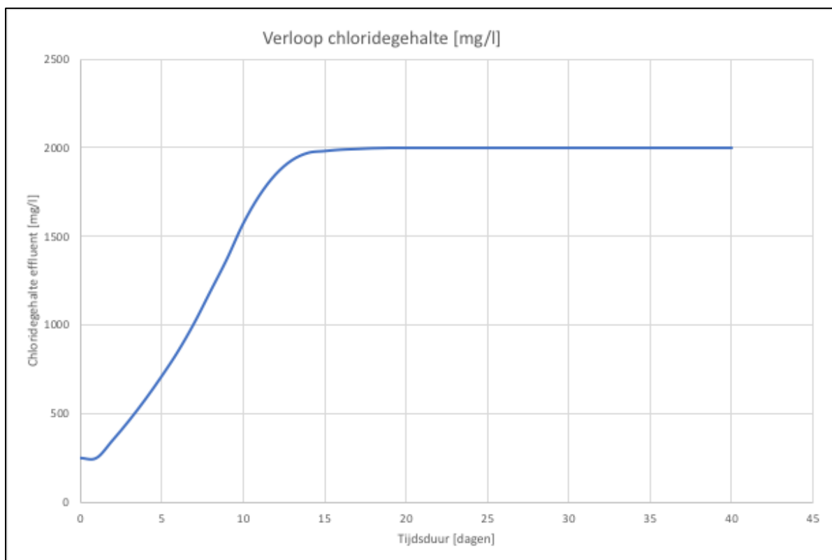
Figuur 17: Worst-case verloop chloridegehalte in het effluent a.g.v. onttrekken van dieper chloridehoudend grondwater.
