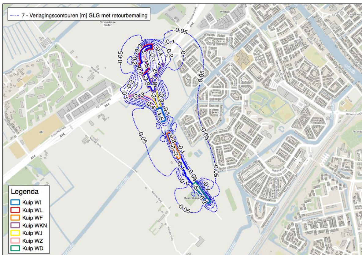
Figuur 12: Verlagingscontouren [m] deklaag a.g.v. spanningsbemaling, met retourbemaling op de systeemgrenzen, onder GLG-condities.
