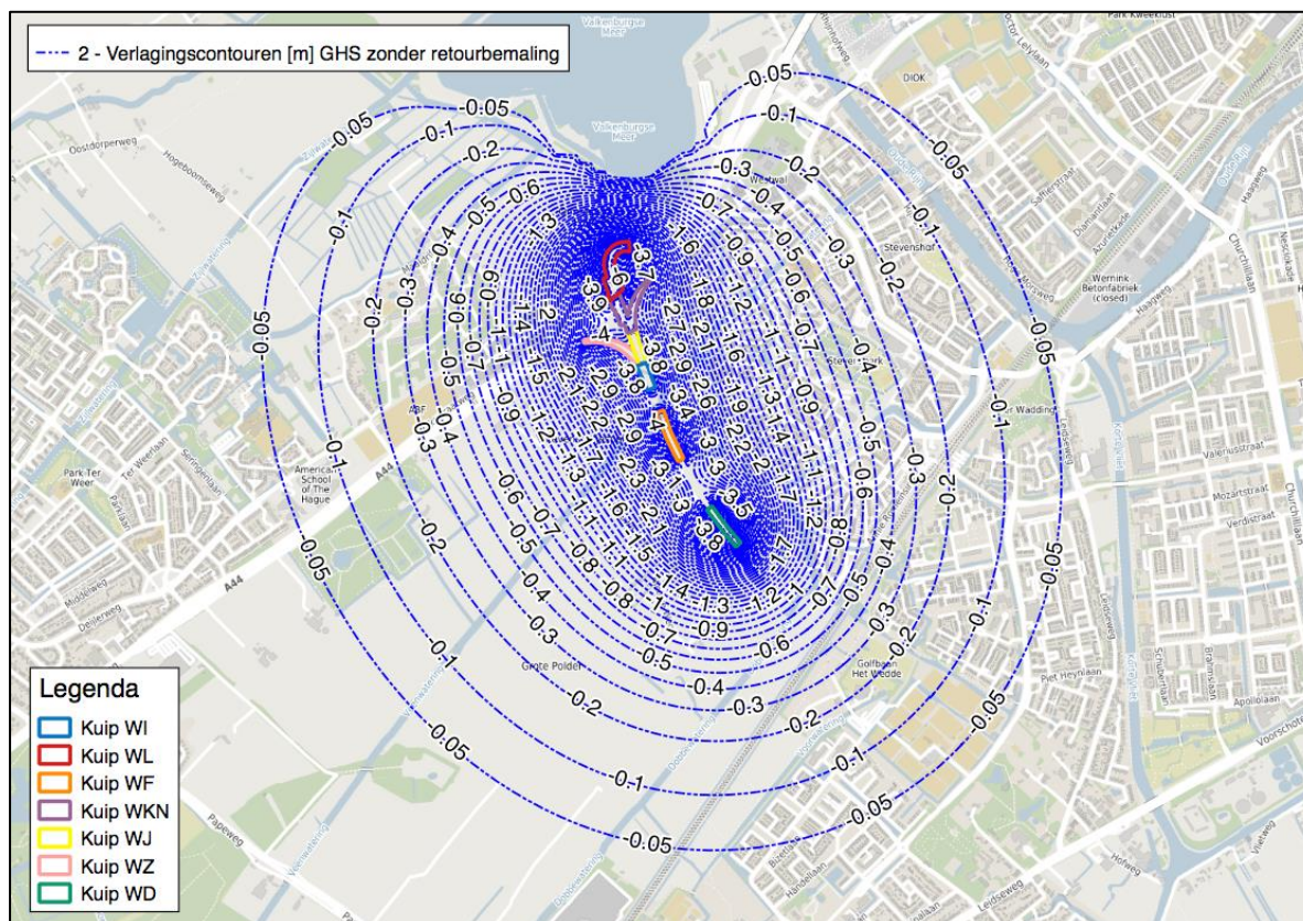
Figuur 10: Verlagingscontouren [m] eerste watervoerend pakket a.g.v. spanningsbemaling, zonder retourbemaling, onder GHS-condities.
