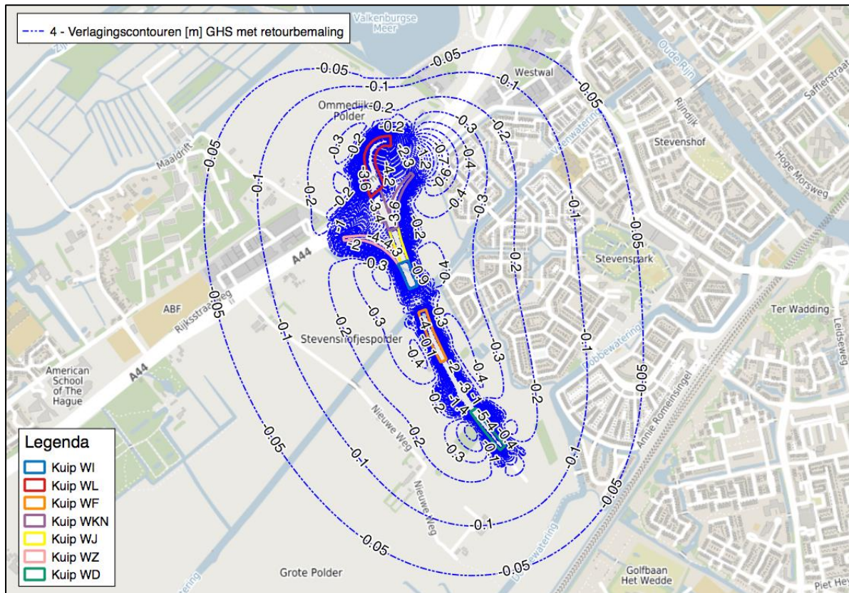
Figuur 15: Verlagingscontouren [m] eerste watervoerend pakket a.g.v. spanningsbemaling, met retourbemaling op de systeemgrenzen, onder GHS-condities.
