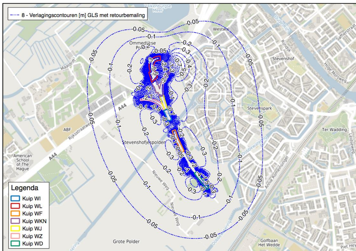
Figuur 13: Verlagingscontouren [m] eerste watervoerend pakket a.g.v. spanningsbemaling, met retourbemaling op de systeemgrenzen, onder GLS-condities.
