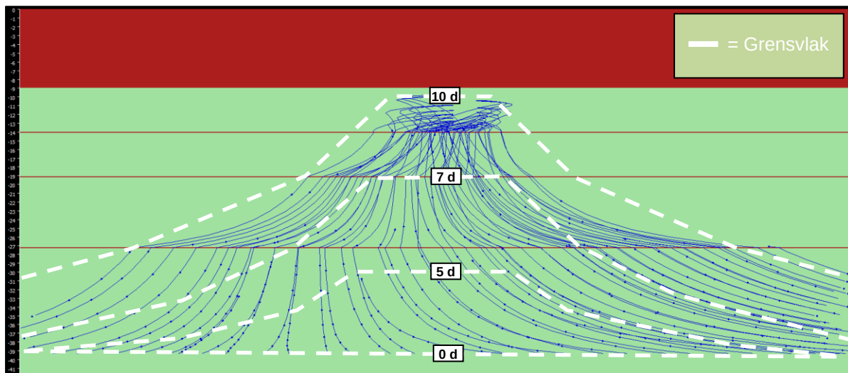
Figuur 16: Upconing zoet-zoutgrensvlak berekend met MicroFEM. Strooming opwaarts. NB. De afstand tussen twee punten op de betreffende flowline staat voor een afgelegde afstand richting de onttrekking in 1 dag. Na ca. 10 dagen bereikt het zoute grondwater de onttrekking, waar het vermengd wordt met het ondiepere zoetwater.
